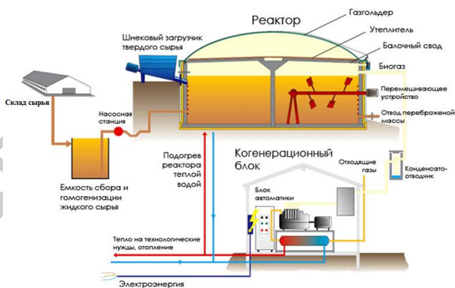
Рисунок 1. Принципиальная схема биогазового реактора
