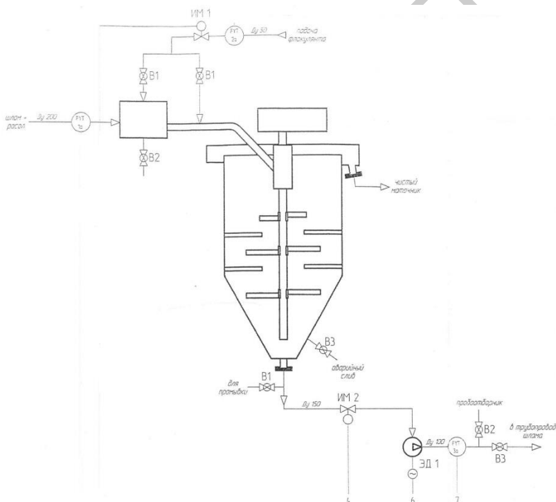
Рис. 1 – Установка выщелачивания хлорида калия из глинисто-солевого шлама
