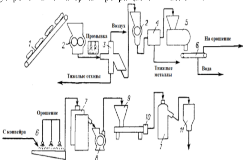
Рис. 1 – Схема регенерации пластмассовых отходов:
