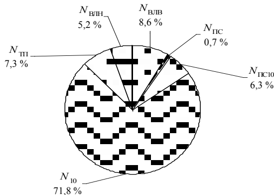
Рис. 2. Диаграмма распределения количества отключений по элементам цепи «источник – потребитель»: N_{ВЛВ} – на ЛЭП 110(35) кВ и в РУ 110(35) кВ, присоединенных к ней ПС; N_{ПС} – в трансформаторе, питающем потребителя ПС 110(35)/10 кВ; N_{ПС10} – в РУ 10 кВ питающей потребителя ПС 110(35)/10 кВ; N_{10} – на питающей потребителя ВЛ 10 кВ; N_{ТП} – в ТП 10/0,4 кВ, к которой подключен потребитель; N_{ВЛН} – на питающей потребителя линии 0,38 кВ
