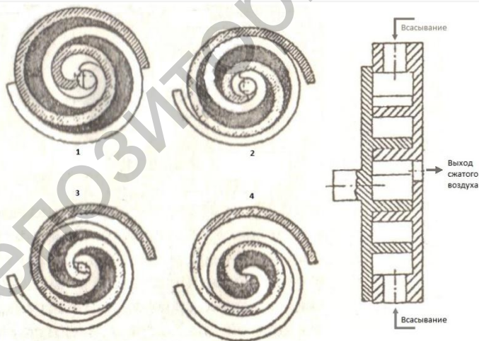
Рисунок 1 – Принцип действия спирального компрессора
