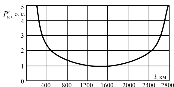
Рис. 1. Зависимость систем предела передаваемой мощности от дальности
