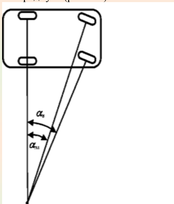
Рис.5.7. Кинематика поворота автомобиля
