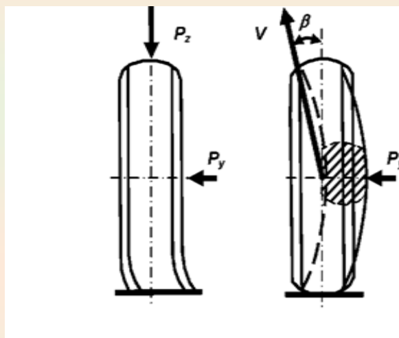
Рис.5.8 Схема увода колеса в следствии действия боковой силы
