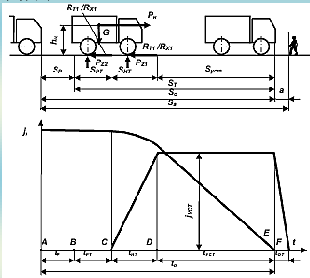
Рис. 5.4. Остановочный и тормозной пути автомобиля
