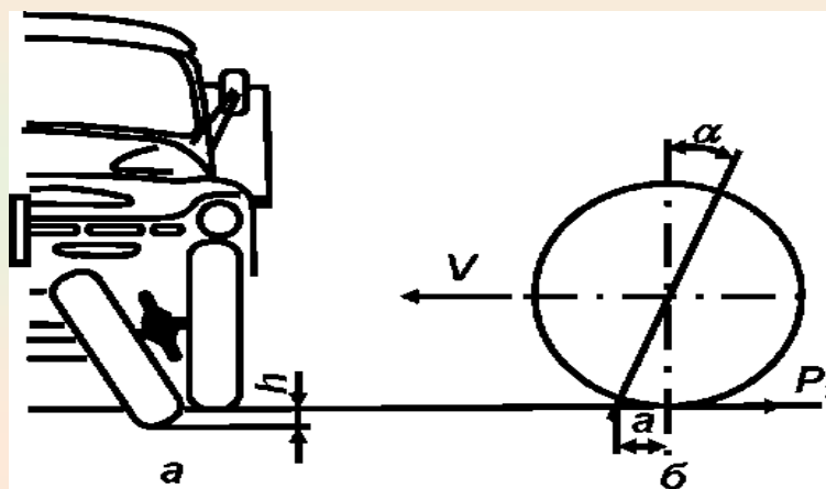
Рис. 5.6. Принцип создания весового положения
