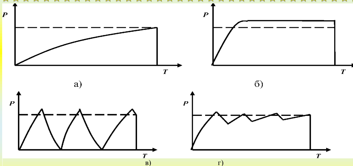
Рис. 1.10. Способы торможения: а - плавный; б - резкий; в - прерывистый; г - ступенчатый; T - время, необходимое для полной остановки автомобиля; P - усилие на педали тормоза.
