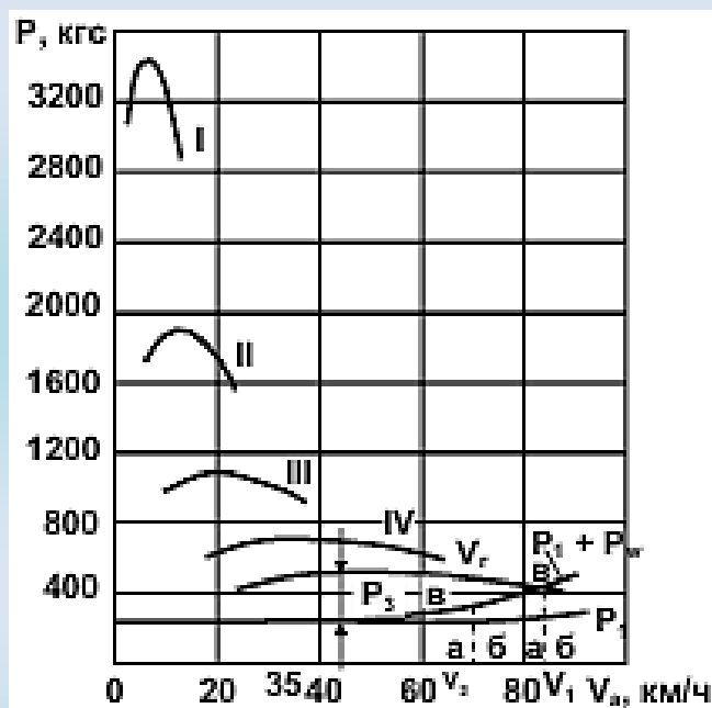
Рис.5.3. График тягового баланса автомобиля
