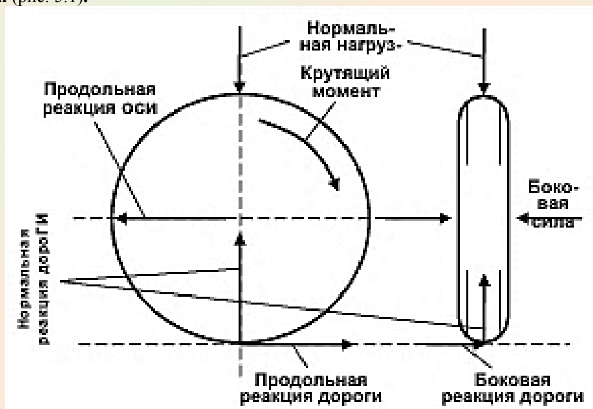
Рис.5.1 Схема сил и моментов, действующих на ведущее колесо автомобиля
