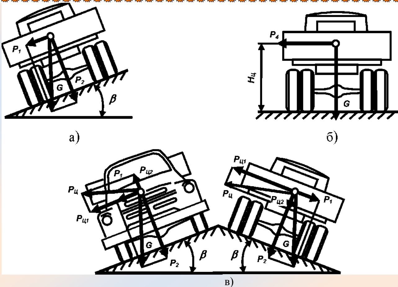
Рис.5.5. Схема сил, действующих на автомобиль
