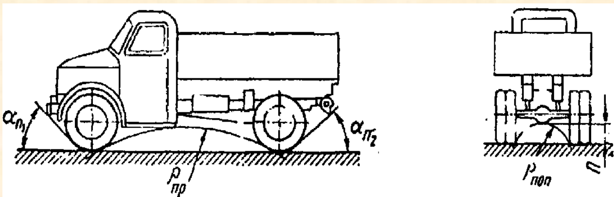
Рис.5.9 Геометрические показатели проходимости
