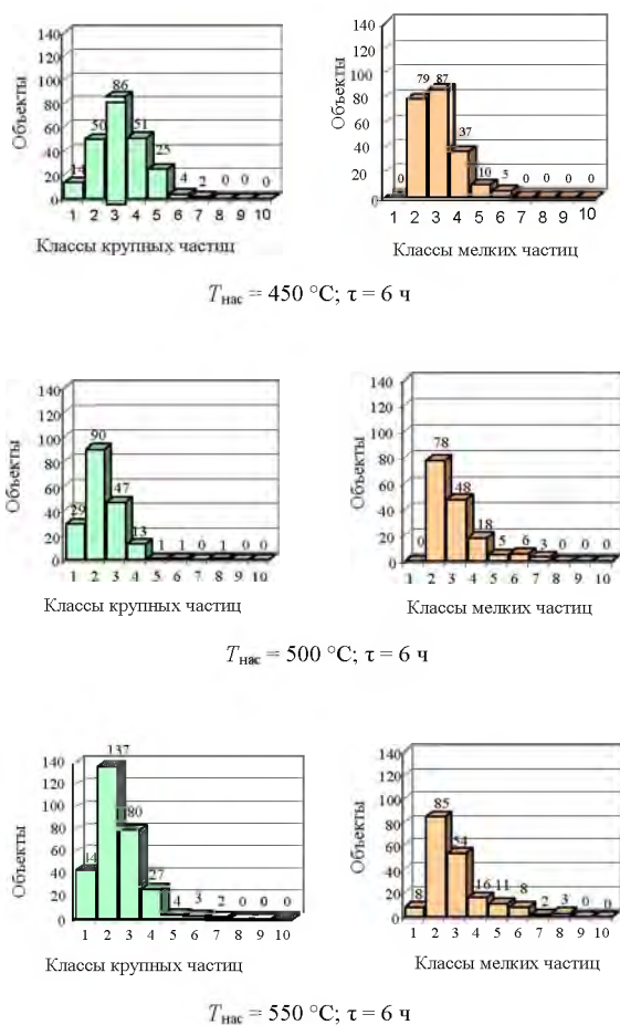
Рис. 5. Гистограммы распределения частиц по дисперсности в зависимости от температуры обработки
