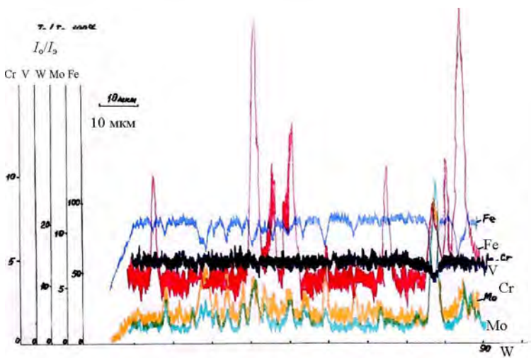
Рис. 3. Распределение элементов по толщине диффузионного слоя при T_{\text{нас}} = 500 \text{ } ^\circ\text{C}
