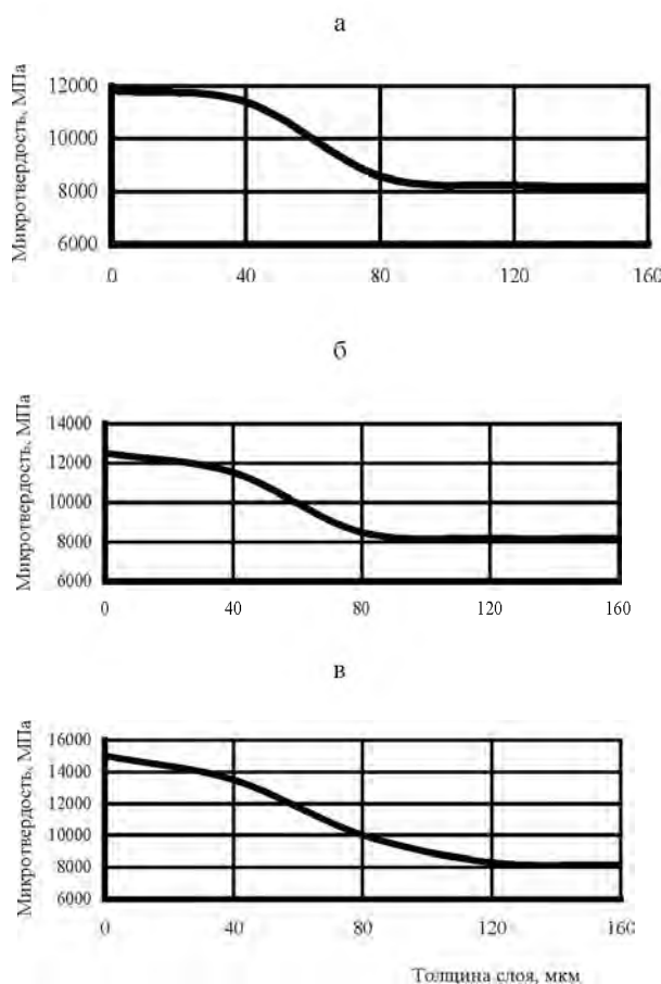
Рис. 6. Распределение микротвердости по толщине карбонитридного слоя на стали Р6М5: а – T_{\text{нас}} = 450 °С; б – 500 °С; в – 550 °С
