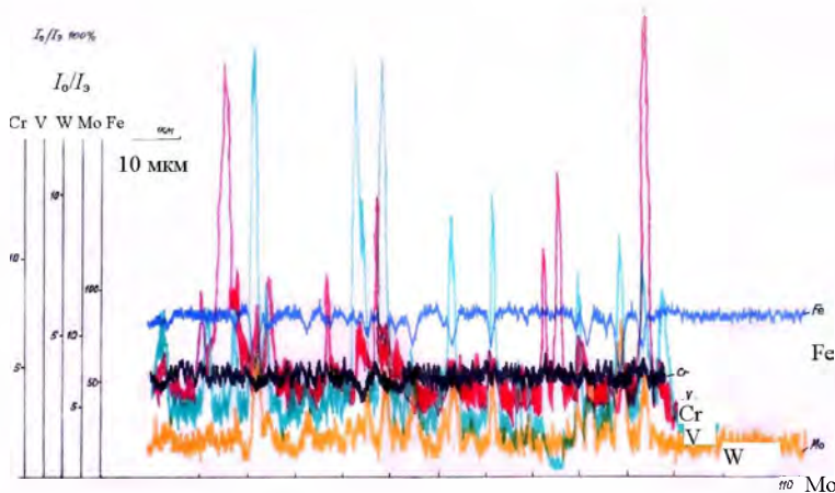
Рис. 2. Распределение элементов по толщине диффузионного слоя при T_{\text{нас}} = 450 \text{ } ^\circ\text{C}
