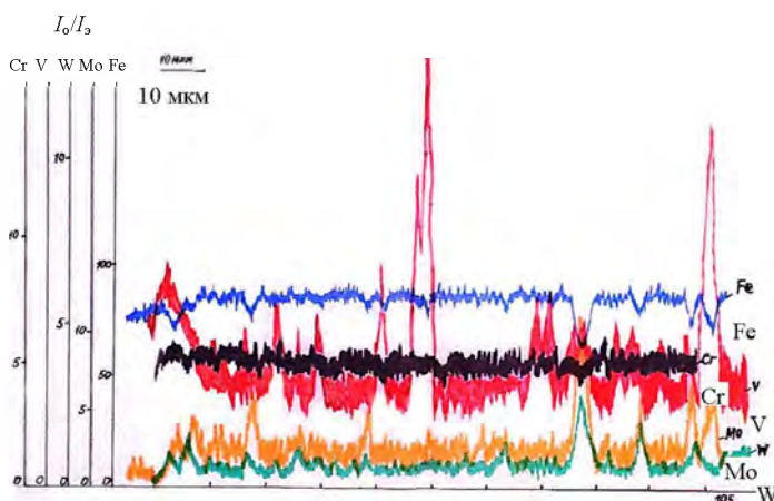
Рис. 4. Распределение элементов по толщине диффузионного слоя при T_{\text{нас}} = 550 \text{ } ^\circ\text{C}
