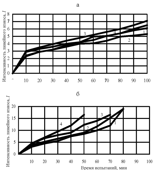
Рис. 7. Зависимость интенсивности линейного износа быстрорежущей Р6М5 от времени испытаний: а – нагрузка 50 МПа; б – 400 МПа; 1 – карбонитрированная сталь Р6М5 ( T_{нас} = 450\text{ °C} ); 2 – то же (500 °С); 3 – то же (550 °С);
