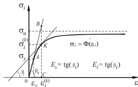
Рис. 4. Зависимость \sigma_i(\varepsilon_i) для упругого слоя основания
