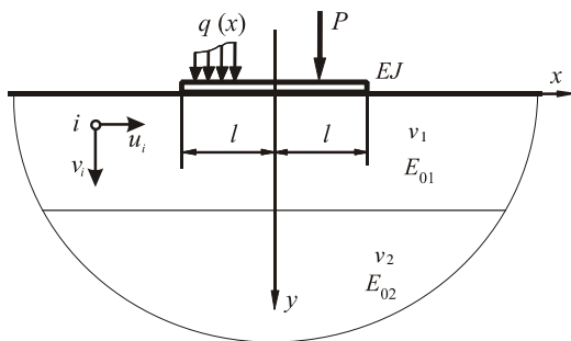
Рис. 1. Балочная плита на упругом слоистом основании
