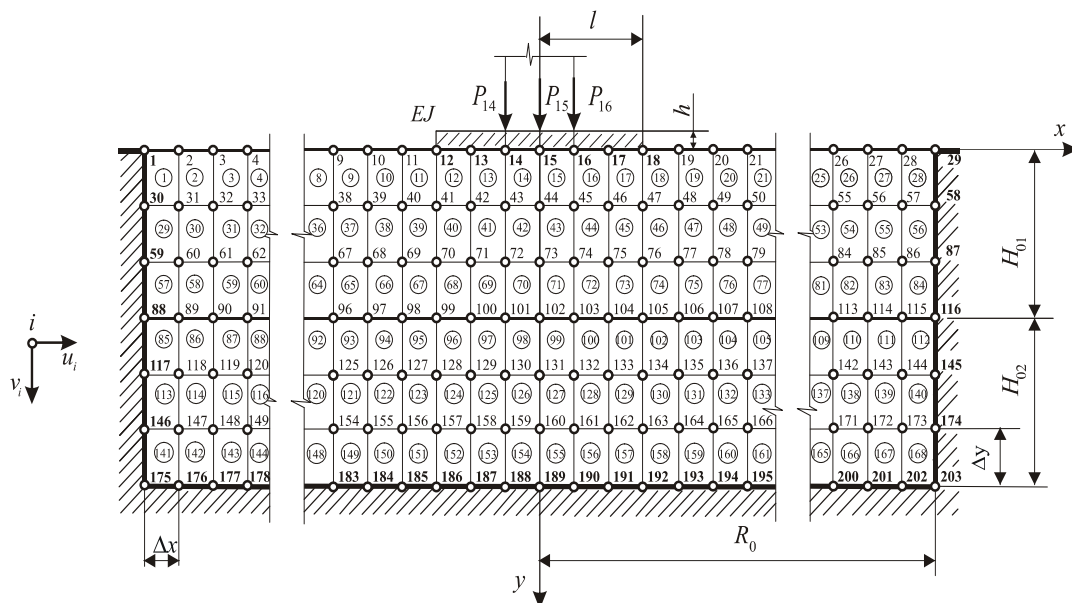
Рис. 3. Разбивочная сетка расчетной области
