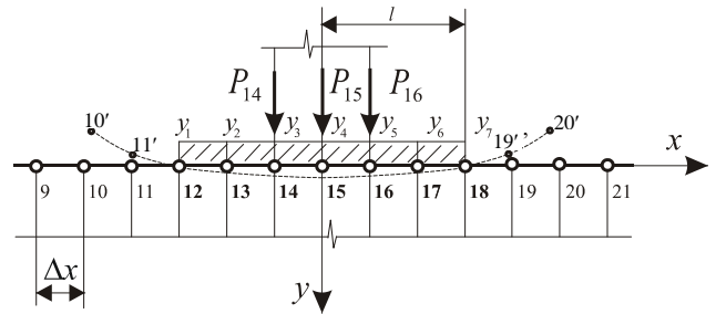
Рис. 6. К определению реактивных давлений в зоне контакта балочной плиты с основанием и внутренних усилий в плите
