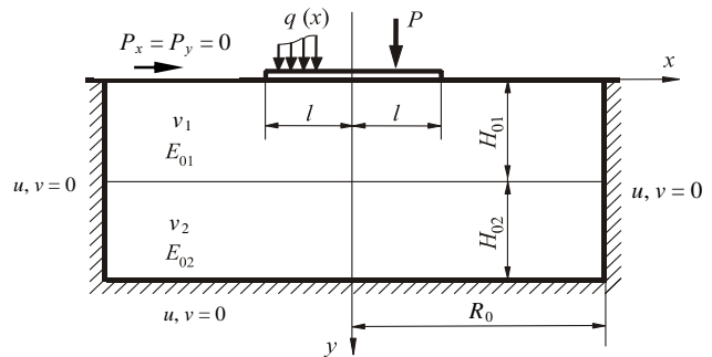
Рис. 2. Расчетная область. Граничные условия задачи
