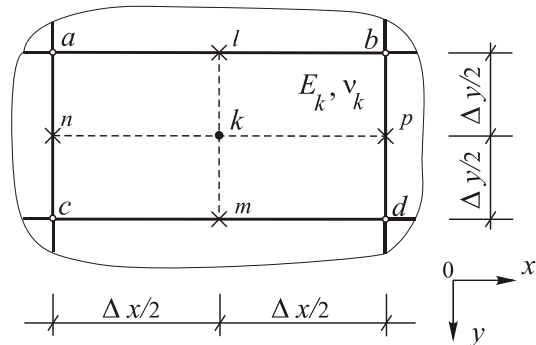
Рис. 5. Прямоугольная ячейка метода конечных разностей
