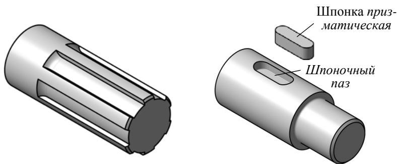
Рис. 1.10. Вал со шлицами прямоугольными
