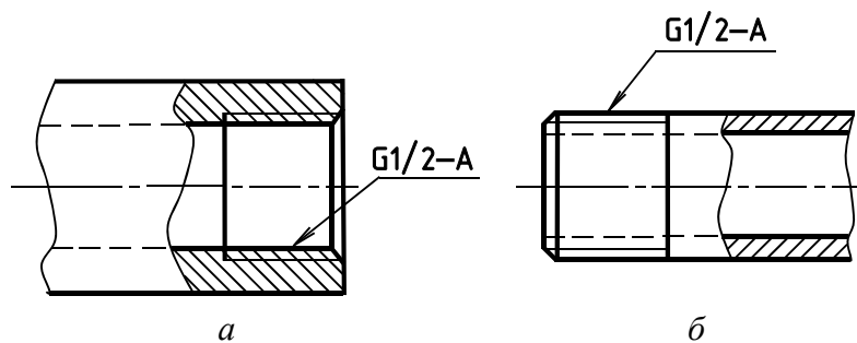
Рис. 2.3. Обозначение на чертеже трубной резьбы: a – внутренней; б – наружной (в обоих случаях в обозначении резьбы свинчиваемых деталей в дюймах указывается диаметр проходного отверстия в трубе, на которой выполнена наружная резьба, то есть изображенной справа)
