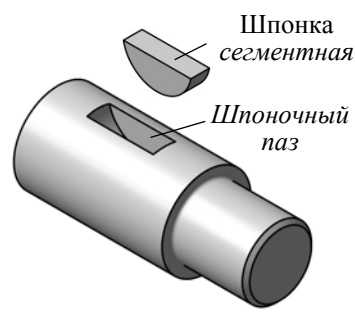
Рис. 1.12. Вал с пазом под сегментную шпонку
