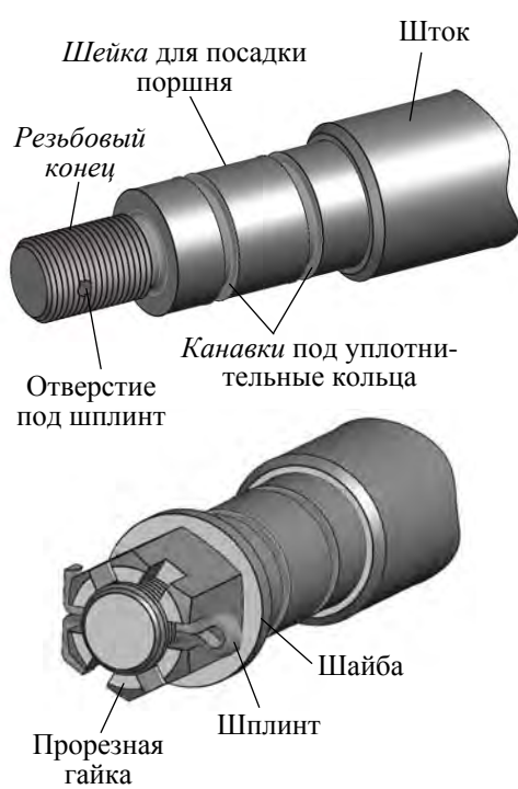
Рис. 1.29. Использование прорезной гайки, стопорящейся шплинтом, на конце штока (для удержания поршня)
