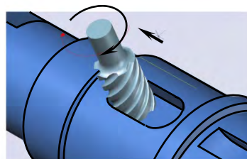
Фрезерование паза под призматическую шпонку торцевой фрезой
