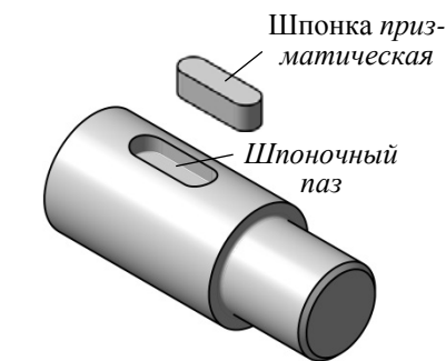
Рис. 1.11. Вал с пазом под призматическую шпонку
