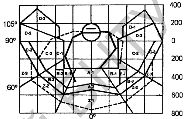
Рисунок 2. Графическое изображение способа построения рабочей зоны в горизонтальной плоскости
