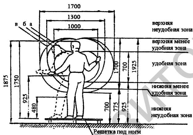
Рисунок 3 – Микроклассификация рабочего пространства в вертикальной плоскости
