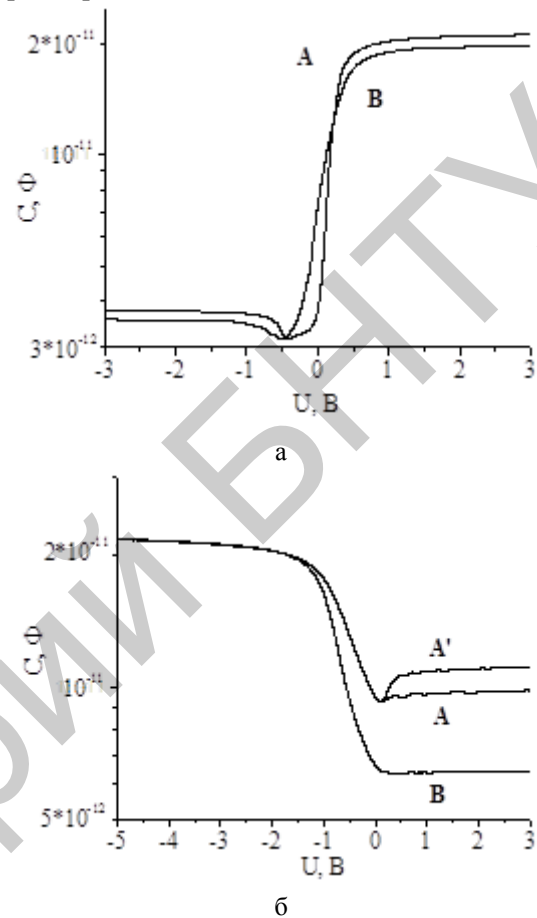
Рисунок 1 – Вольт-фарадные характеристики МОП-транзисторов, измеренные на n -кармане (а) и на p -кармане (б)
