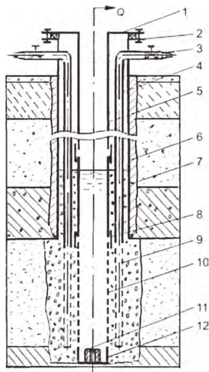
Рис. 1. Конструкция водозаборной скважины с затрубной системой регенерации
