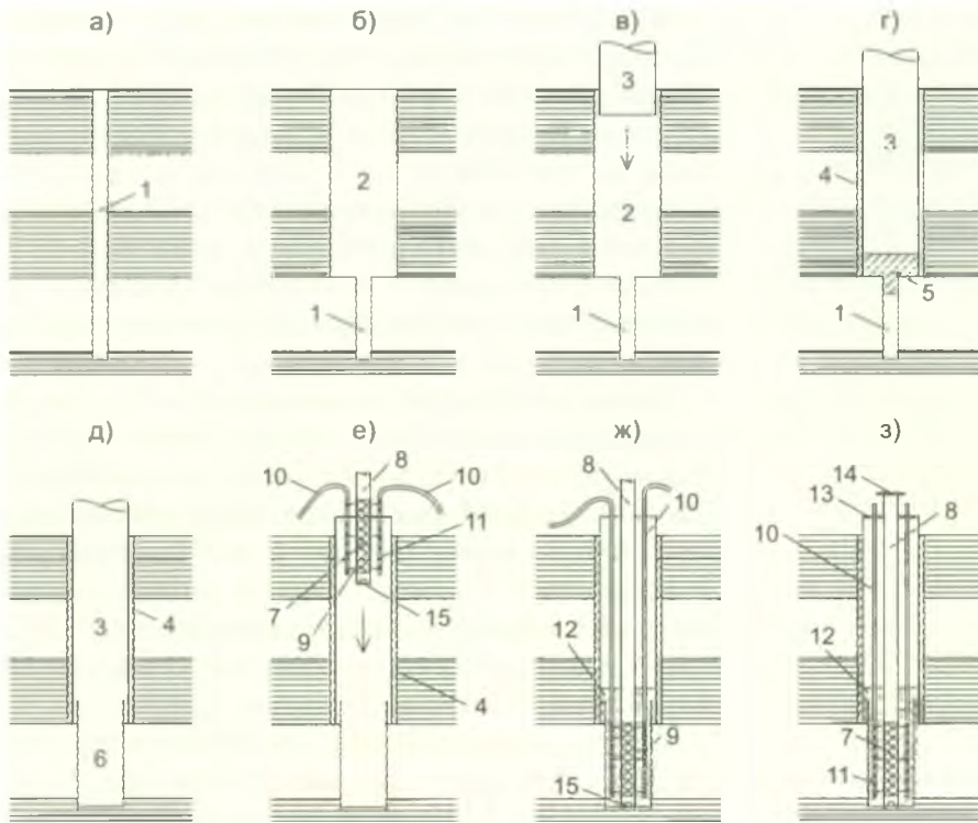
Рис. 3. Технологическая последовательность бурения водозаборной скважины
