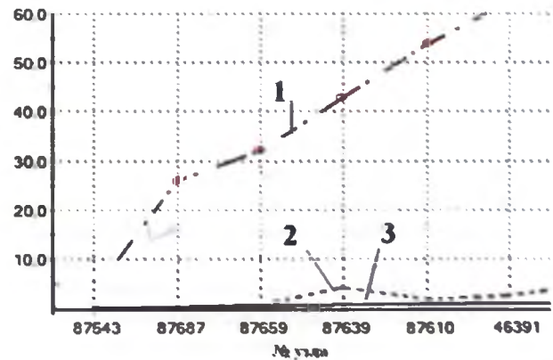
Рисунок 8 — Графики перемещений точек зондирования продольных направляющих стола с контактом: 1 — в 30 %; 2 — в 60 %; 3 — в 100 %
