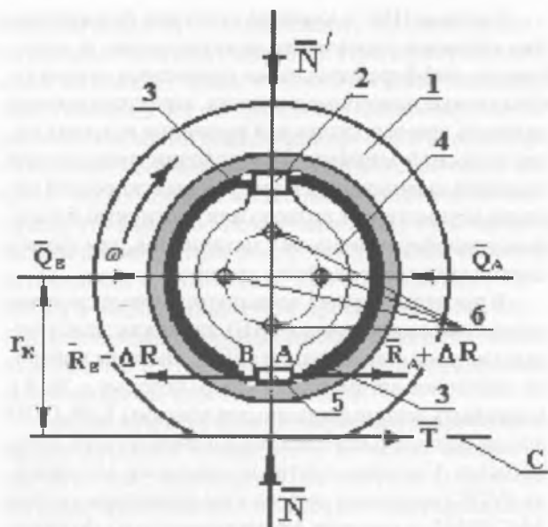
Рисунок 3 — Схема к пояснению способа измерения тормозного момента в барабанном тормозе: 1 — тормозящее колесо с тормозным барабаном; 2 — разжимное устройство колодок тормоза; 3 — тормозные колодки; 4 — суппорт тормоза; 5 — опорная пластина колодок тормоза; С — поверхность дороги; \omega — угловая скорость вращения колеса; r_k — радиус качения колеса; \bar{R}_A, \bar{R}_B — реакции в точках «А» и «В» опоры пластины 5; R_B - R_A = \Delta R — разность реакций, возникающая при приложении момента к колесу; \bar{N} — нормальная реакция дороги С; \bar{Q}_A, \bar{Q}_B — разжимные усилия колодок тормоза
