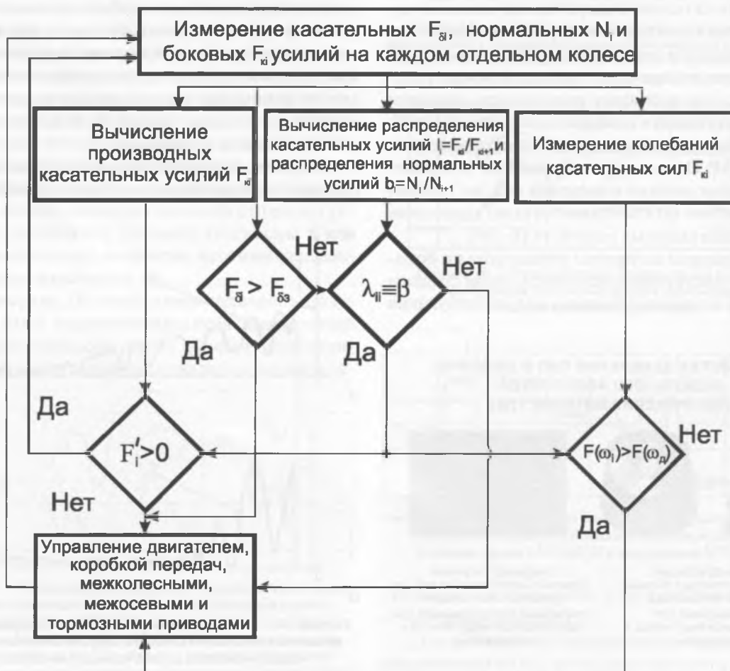
Рисунок 25 — Алгоритм управления движением полноприводной колесной машиной
