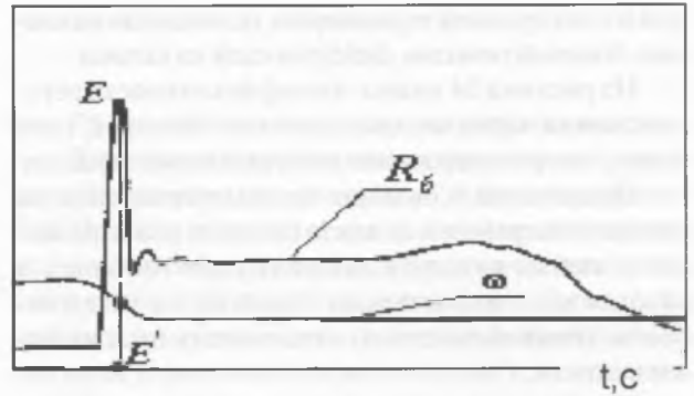
Рисунок 23 — Осциллограмма изменения боковой реакции и угловой скорости вращения заднего правого колеса автомобиля ВА3-2108 при экстренном торможении (начальная скорость торможения V=90 км/ч; опорная поверхность типа «μ-split»): R_b — боковая реакция; \omega — угловая скорость вращения колеса тормозящего колеса
