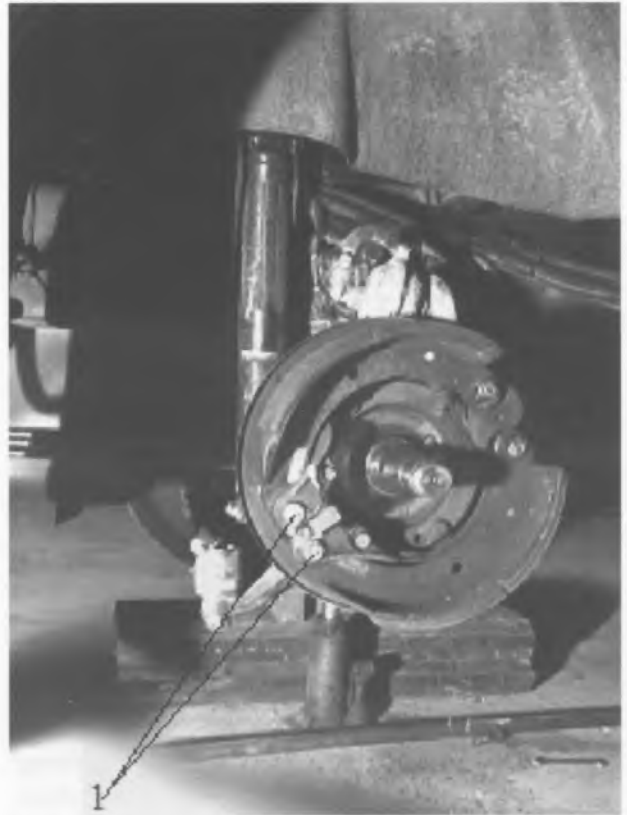
Рисунок 7 — Барабанный тормоз с поворотными осями колодок, включающих индукционные датчики измерения сил: 1 — поворотные оси колодок барабанного тормоза автомобиля МАЗ-544018-320-030, включающие индукционные датчики измерения сил
