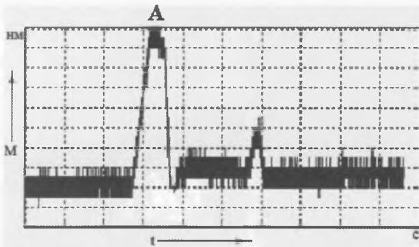
Рисунок 9 — Осциллограмма изменения \Delta R (тормозной момент колеса барабанного тормоза) при экстренном торможении седельного тягача МАЗ-544018-320-030 (начальная скорость торможения 15 км/ч, торможение без АБС)
