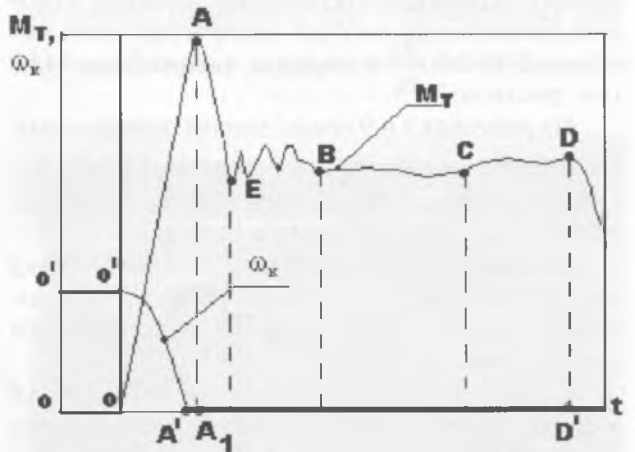
Рисунок 8 — Осциллограмма изменения \Delta R , пропорционального тормозному моменту, фактически реализуемому колесом автомобиля ВАЗ-2108 с опорной поверхностью при его экстренном торможении:
