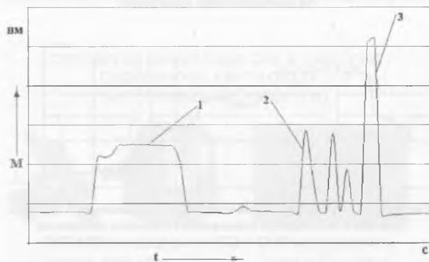
Рисунок 15 — Осциллограмма изменения тормозного момента при торможении колеса легкового автомобиля «Фольксваген»: 1 — торможение с удержанием педали тормоза нажатой; 2 — кратковременное торможение с различной силой нажатия на тормозную педаль; 3 — экстренное торможение колеса с максимальной интенсивностью нажатия на тормозную педаль
