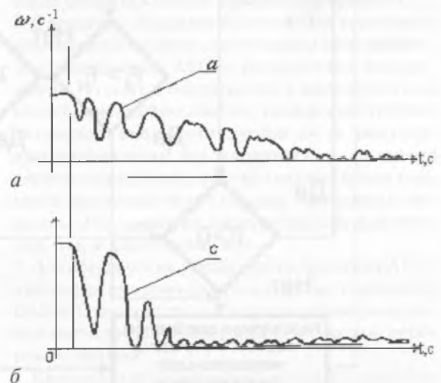
Рисунок 24 — Осциллограммы регулирования угловой скорости вращения тормозящего колеса по опорной поверхности типа «микст» (скорость начала торможения 100 км/ч): а — регулирование по тормозному моменту; б — регулирование по боковой реакции колеса
