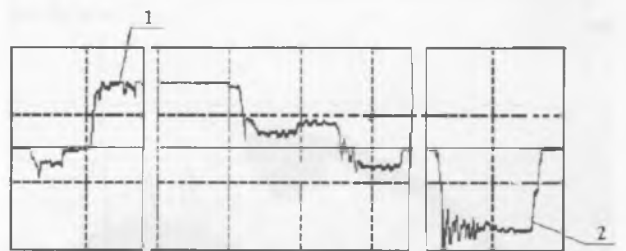
Рисунок 21 — Осциллограмма изменения сил в шкворне в процессе разгона и экстренного торможения седельного автопоезда в составе тягача МАЗ-64229 и полуприцепа МТМ 9330
