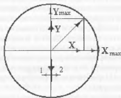
Рисунок 1 — Взаимосвязь между касательной и боковой реакциями в контакте колеса с опорной поверхностью: 1 — тяговый режим; 2 — тормозной режим; Y — касательная реакция в контакте колеса с опорной поверхностью; X — боковая реакция в контакте колеса с опорной поверхностью
