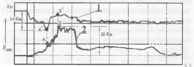
Рисунок 20 — Осциллограмма изменения сил в шкворне автопоезда при его экстренном торможении на криволинейной траектории
