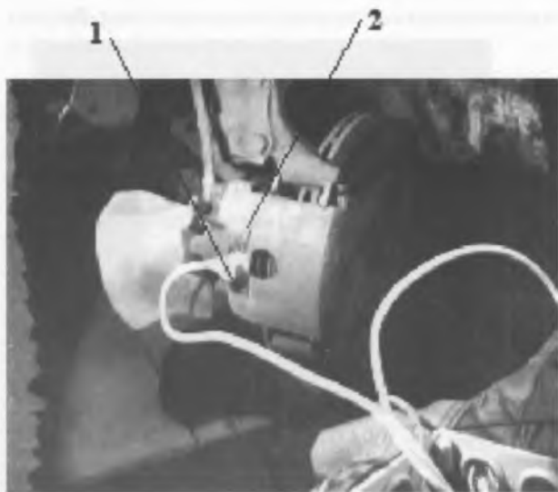
Рисунок 14 — Установка датчика измерения тормозного момента, основанного на изменении внутренних механических напряжений на скобе переднего дискового тормоза легкового автомобиля «Фольксваген»: 1 — датчик измерения тормозного момента; 2 — скоба дискового тормоза
