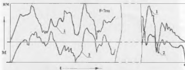
Рисунок 17 — Осциллограмма изменений тормозных моментов на переднем (дисковый тормоз) и заднем (барабанный тормоз) колесах автомобиля «ВАЗ-2108» при экстренном торможении (частота срабатывания электромагнитного клапана модулятора Биш-2 составляла f = 7 Гц, дорога — уплотненный снежный покров): 1 — тормозной момент на колесе с дисковым тормозом; 2 — тормозной момент на колесе с барабанным тормозом
