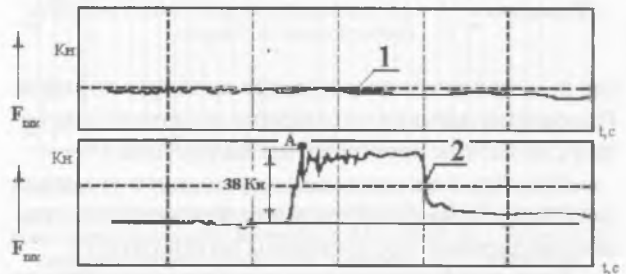
Рисунок 19 — Осциллограмма изменения сил в шкворне при прямом торможении седельного автопоезда в составе тягача МАЗ-64229 и полуприцепа МТМ 9330: 1 — силы в поперечном направлении; 2 — силы в продольном направлении
