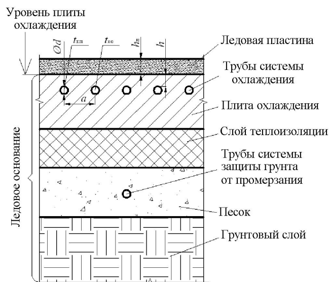
Рис. 1. Конструкция основания ледового поля на грунте: a = 100 мм; \varnothing 25 мм; d_n = 32 мм; h_{л} = 25 мм; h = 25 мм
