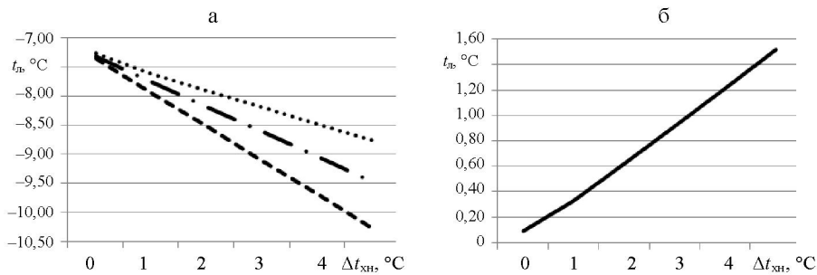
Рис. 4. Зависимости: а – средней, максимальной и минимальной температур поверхности льда; б – температурной неоднородности поверхности ледовой пластины от разности температур хладонносителя ( t_{хп} , °C) в подающем и обратном трубопроводах бетонной плиты охлаждения: t_{опр} = 8\text{ °C} ; t_{хо} = -10\text{ °C} ; t_{хп} = (-10)\text{--}(-15)\text{ °C} ; ..... – T_{\max} ; - · - · - · – T_{\text{средн}} ; - - - - - T_{\min}
