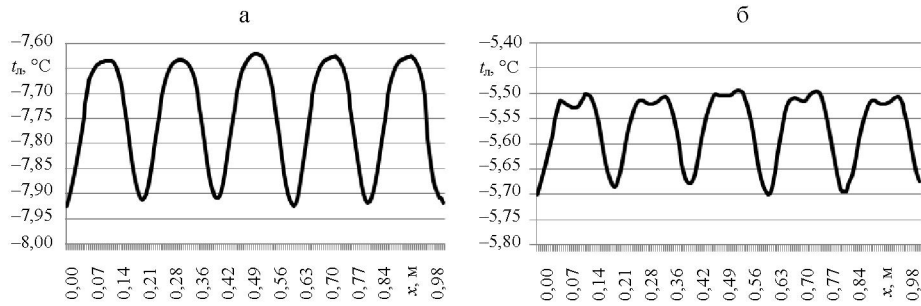
Рис. 3. Распределение температуры на поверхности льда: а – бетонная плита охлаждения; б – плита охлаждения из песчаной засыпки: t_{хп} = -11\text{ °C} ; t_{хо} = -10\text{ °C} ; t_{оп} = 10\text{ °C} ; t_{оо} = 5\text{ °C}
