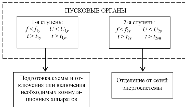
Рис. 1. Структурно-функциональная схема делительной автоматики
