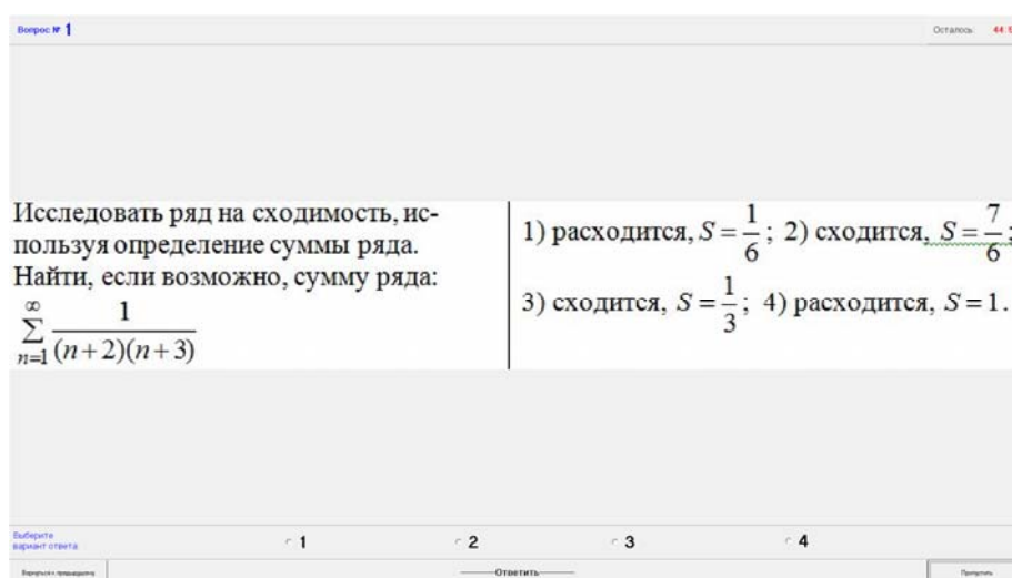
Рисунок 3. Выполнение заданий.
