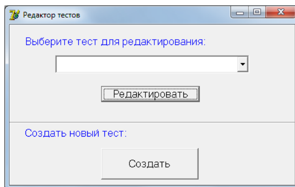
Рисунок 1. Редактор тестов.
