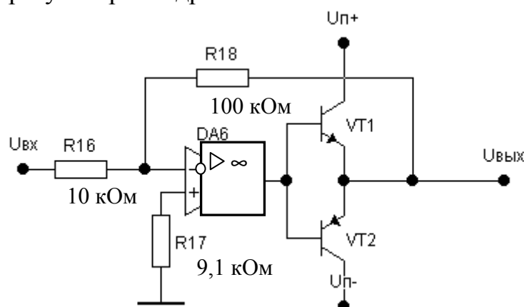
Рисунок 1. Усилитель мощности.
