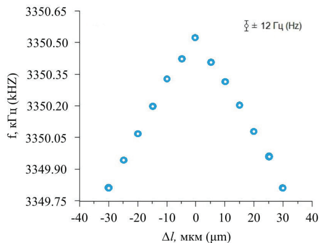
Рисунок 4 – Изменение частоты рециркуляции при смещении торца измерительного волоконного световода
