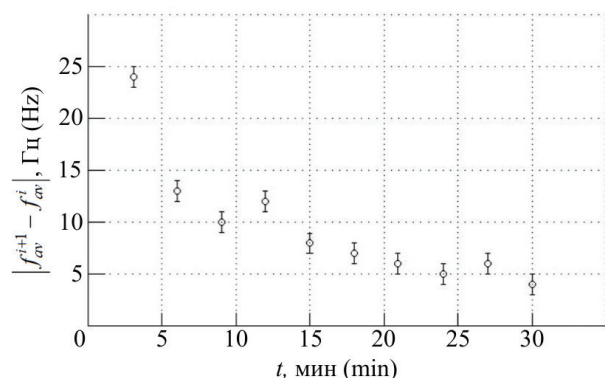
Рисунок 2 – Процесс стабилизации частоты рециркуляции
