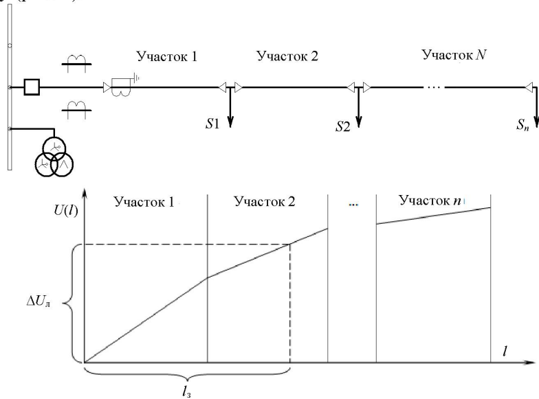
Рис. 3. Диаграмма падения напряжений вдоль линии с отборами мощности при простом однофазном замыкании
