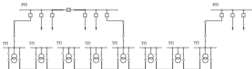
Рис. 1. Структура петлевой схемы электроснабжения
