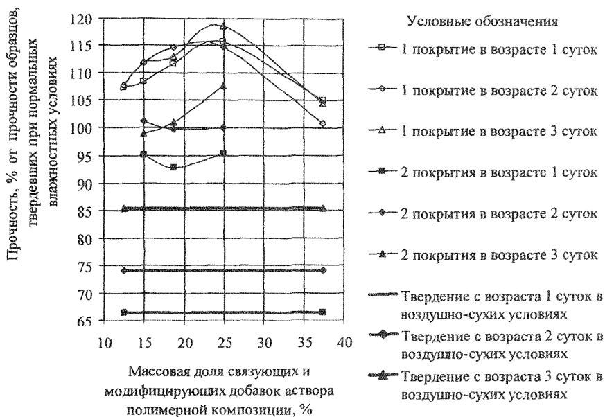
Рисунок 4 - Влияние водных растворов полимерной композиции в течение 19,9 \cdot 10^5 \dots 21,6 \cdot 10^5 с ( 23 \dots 25 суток) на среднюю относительную прочность при осевом сжатии образцов бетона, изготовленных из низкопластичной бетонной смеси
