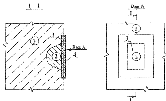
Рисунок 2 - Схема бетонного элемента после приклеивания полиэтиленовой пленки всей поверхностью к бетону ремонтируемого и прилегающему к нему участкам
