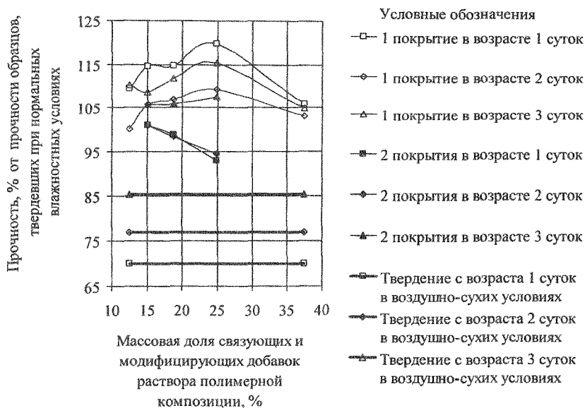
Рисунок 3 – Влияние водных растворов полимерной композиции в течение 9,5 \cdot 10^5 \dots 11,2 \cdot 10^5 с (11...13 суток) на среднюю относительную прочность при осевом сжатии образцов бетона изготовленных из низкопластичной бетонной смеси
