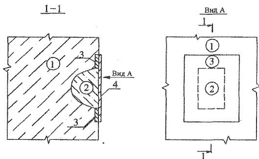
Рисунок 1 – Схема бетонного элемента после приклеивания полиэтиленовой пленки к участку, прилегающему к свежесуложенному бетону
