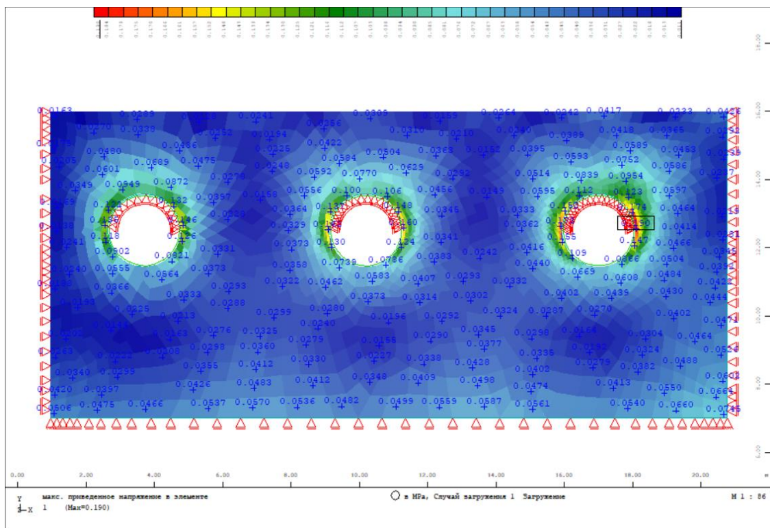
Рисунок 3 – Напряжения в грунте
