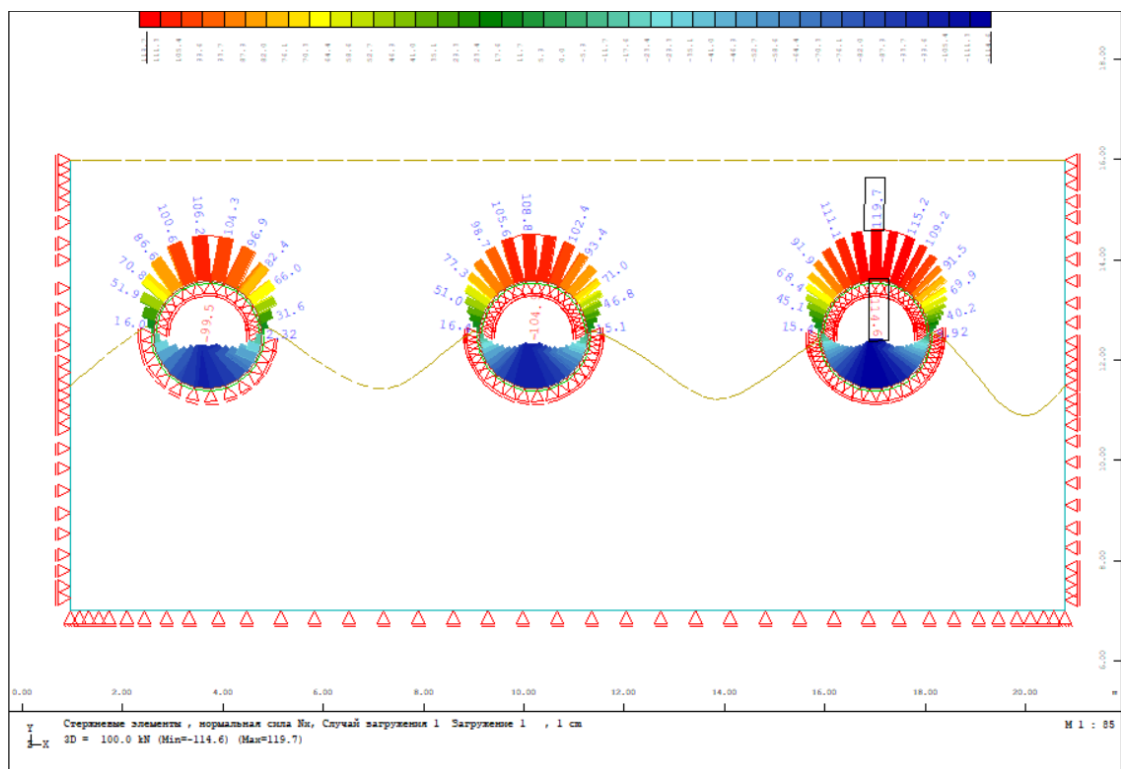
Рисунок 5 – Нормальные силы в элементах
