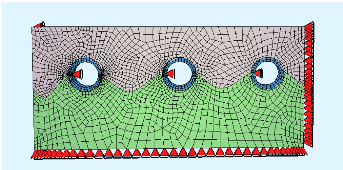
Рисунок 2 – Расчетная схема тоннелей в объеме грунта
