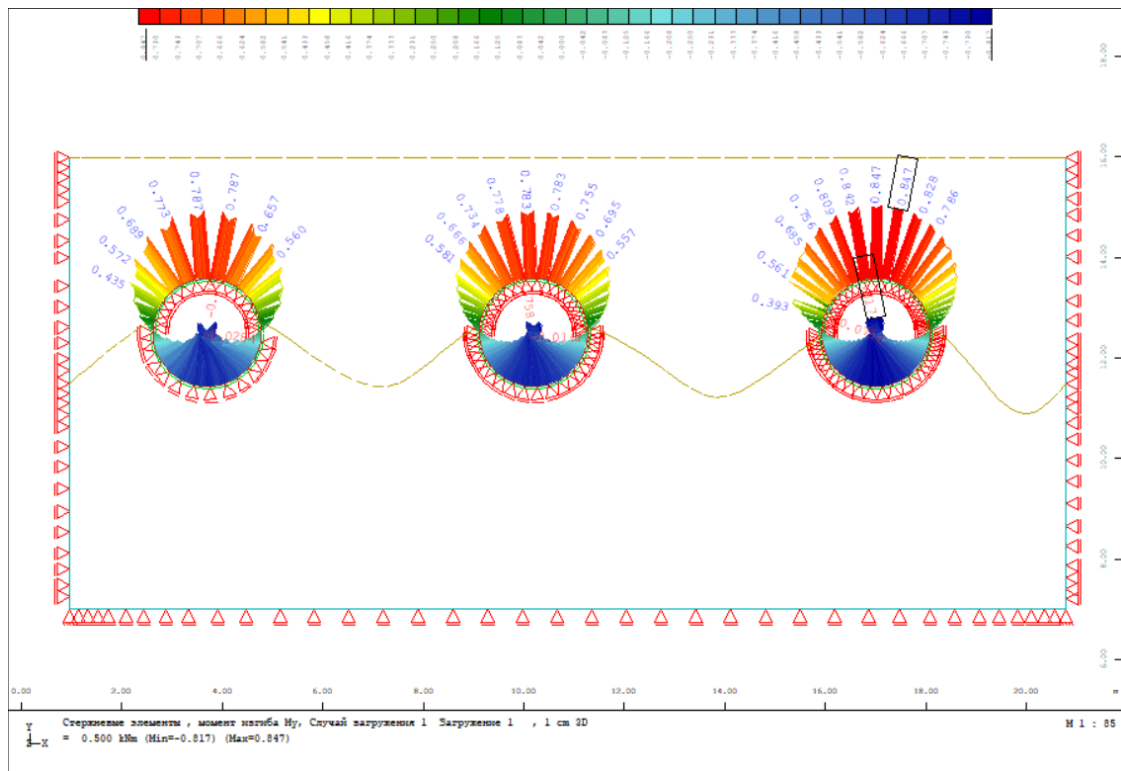
Рисунок 4 – Изгибающие моменты в элементах
