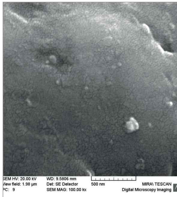
Рис.3. СЭМ-изображение поверхности частиц губчатого порошка марки ТПП-5. × 100 000
