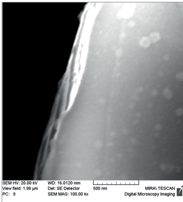
Рис. 2. СЭМ-изображение поверхности скола частицы губчатого порошка марки ТПП-5. × 100 000
