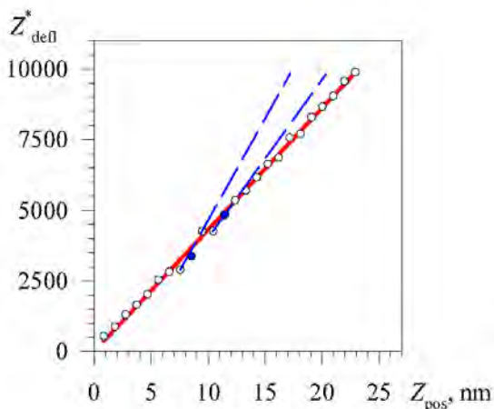
Рисунок 1 – Калибровочная кривая по кремнию
