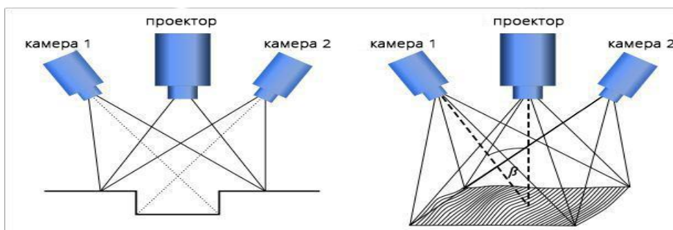
Рисунок 3 – Оптический сканер
