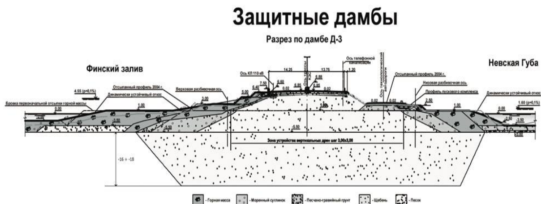
Рисунок 2 – Схема поперечного сечения защитной дамбы
