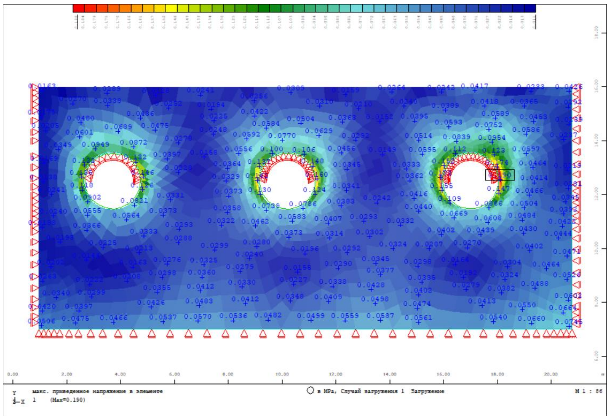
Рисунок 3 – Напряжения в грунте
