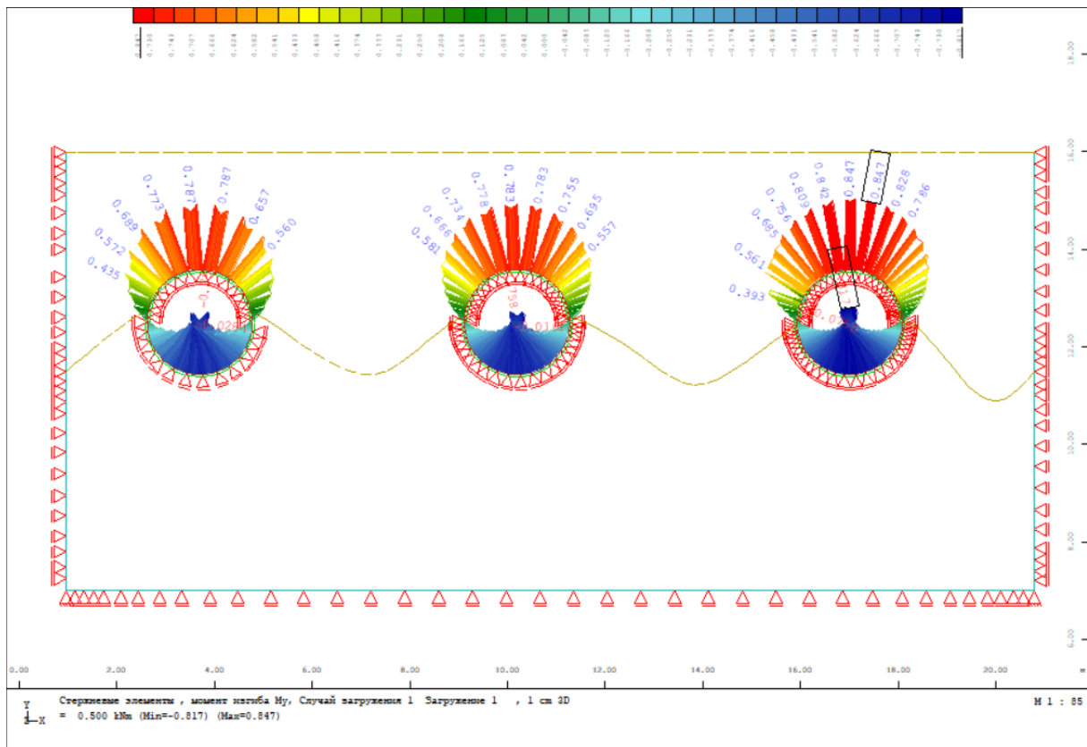
Рисунок 4 – Изгибающие моменты в элементах
