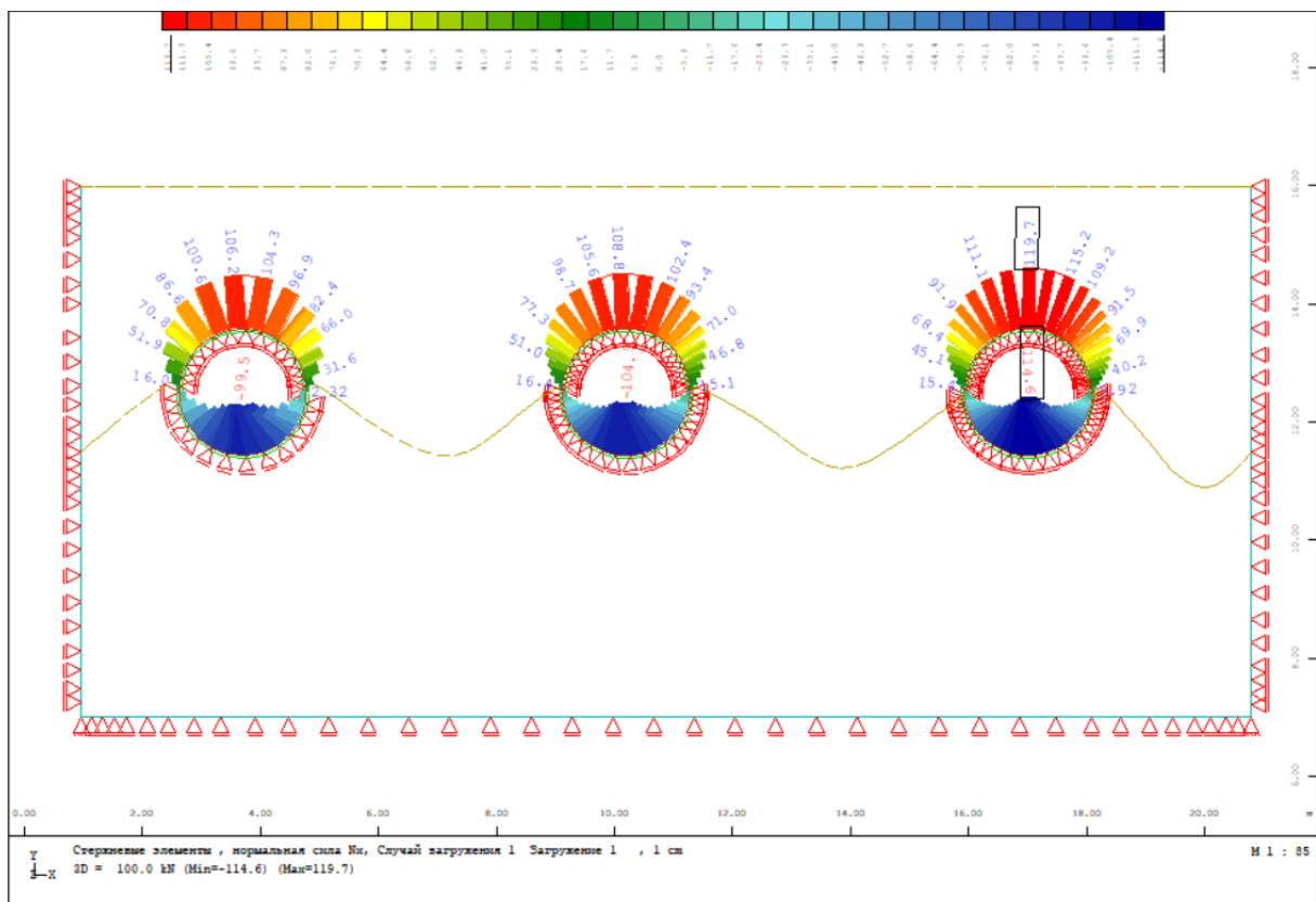
Рисунок 5 – Нормальные силы в элементах
