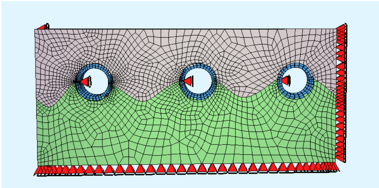
Рисунок 2 – Расчетная схема тоннелей в объеме грунта
