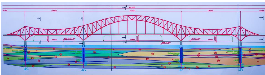
Рисунок 2 – Конструкция моста через реку Иртыш
