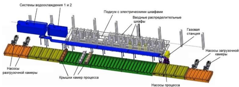
Рисунок 1 - Магнетронный коатер BUHLER Leybold Optics Apollon 3300
