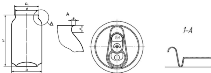
Рисунок 1 – Конструкция алюминиевой банки и легкоскрываемой крышкой
