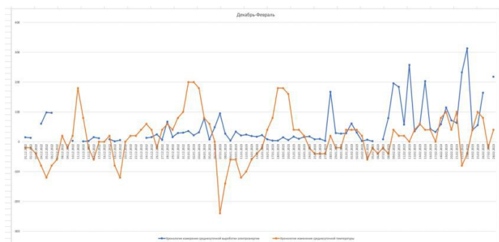
Рисунок 2. – Хронология изменения в течение декабря 2022г. - февраля 2023 г. суточной выработки фотовольтаической станцией Chaplin 1 и среднесуточной температуры окружающего воздуха в районе размещения фотовольтаической станции.
