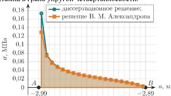
Рисунок 6 – Совместная эпюра контактных напряжений в опорной зоне под абсолютно жесткой балочной плитой
