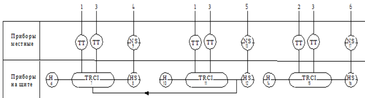
Рисунок 2 – Схема автоматизации
