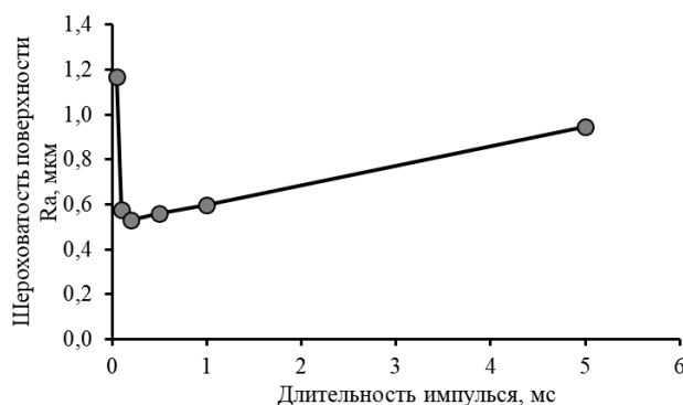
Рисунок 4 - Зависимость шероховатости поверхности оксидного слоя при различной длительности импульсов технологического напряжения
