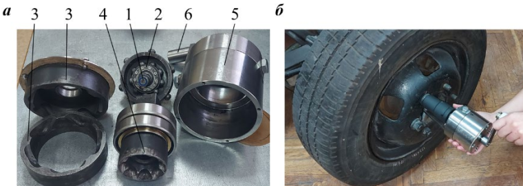
a – основные узлы; б – установка на колесе автомобиля; 1 – ведущий вал с установленным на нем эксцентриком; 2 – спутник; 3 – наружные кулачки; 4 – ведомые вал с кулачком; 5 – корпус; 6 – упор
