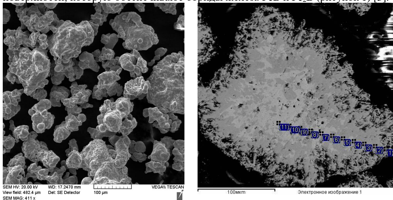
Рисунок 1 – Борированный порошок из дисперсных металлических отходов: а – морфология; б – структура частиц
