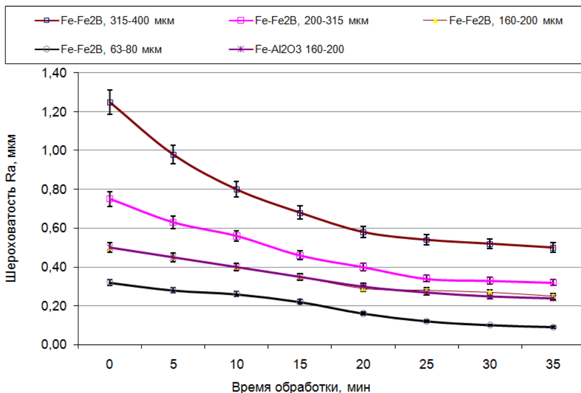
Рисунок 3 – Изменение шероховатости в процессе магнитно-абразивной обработки с использованием различных порошков
