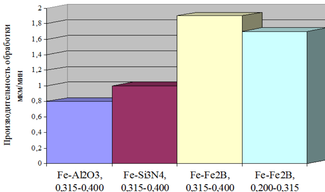
Рисунок 2 – Производительность магнитно-абразивной обработки с использованием различных порошков
