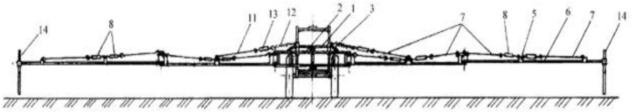
Рис. 1. Штанга опрыскивателя
