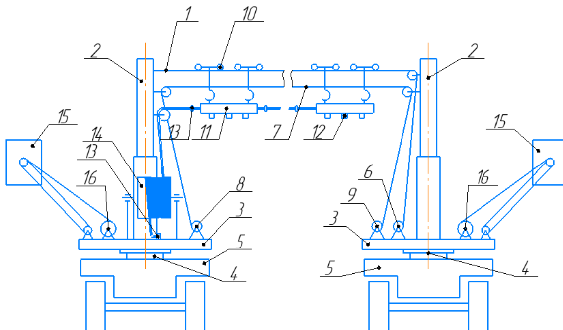
Рис. 4. Мобильная дождевальная установка с использованием канатно-блочной системы:
