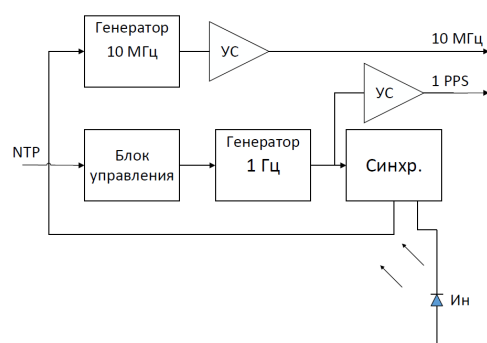
Рисунок 1 – Блок-схема устройства
