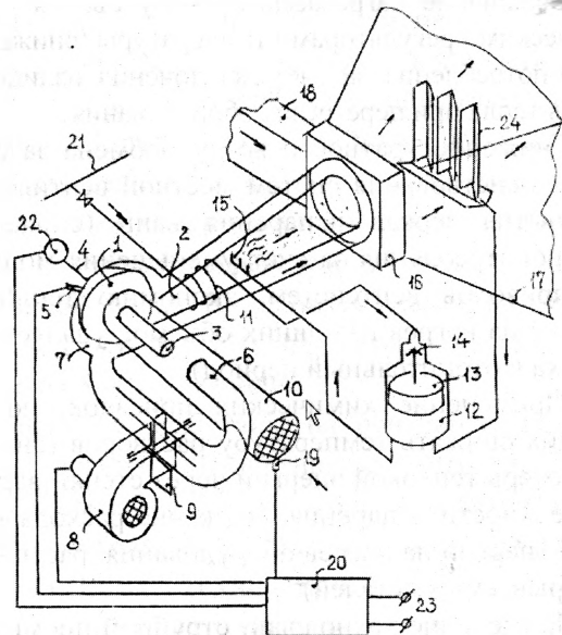
Парогазогенератор
