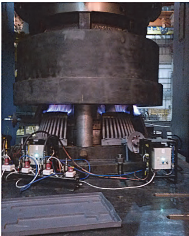
Рис. 3. Установка нагрева штампов
