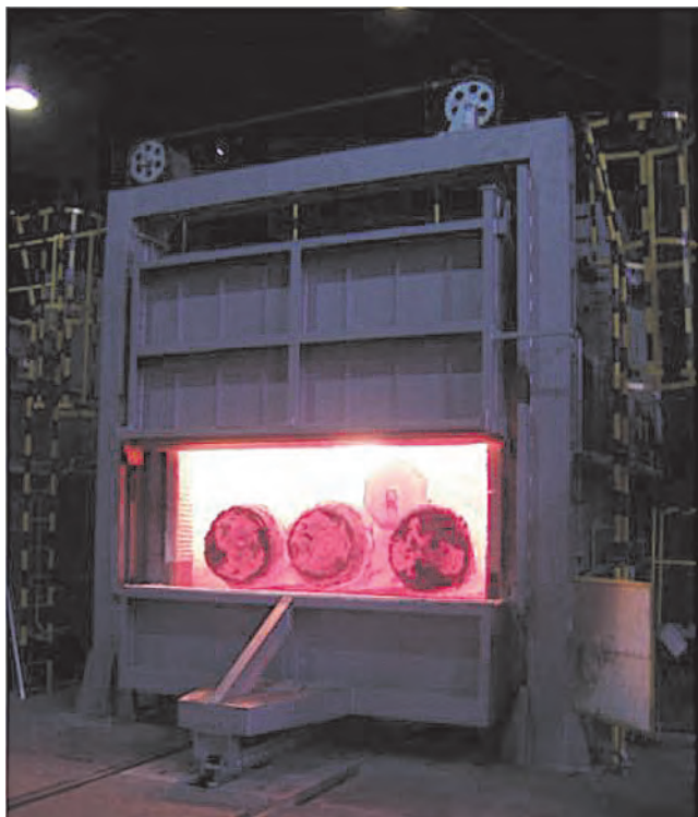
Рис. 1. Печь с выкатным подом
