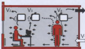
Рис. 3. Схема движения потоков воздуха вытесняющей вентиляции в непроизводственных помещениях
