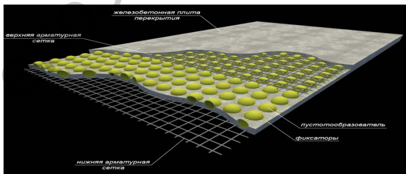
Рисунок 1 – Конструктивное решение многоступенчатого безбалочного перекрытия
