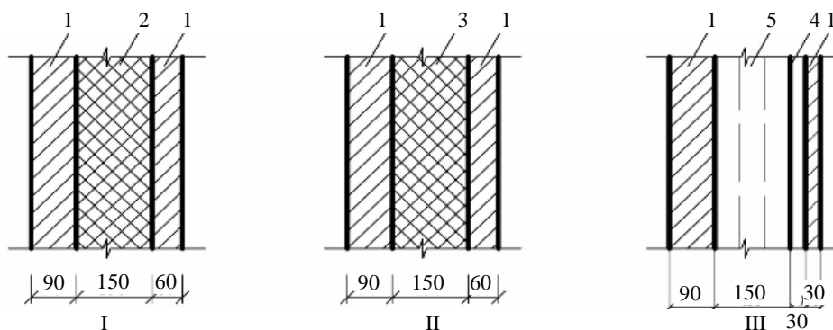
Рис. 2. Варианты наружного ограждения
