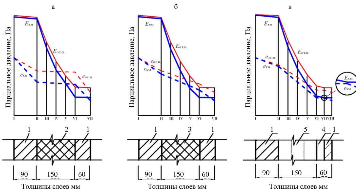
Рис. 3. Графики влажностного режима наружной стены: а – вариант I; б – вариант II; в – вариант III
