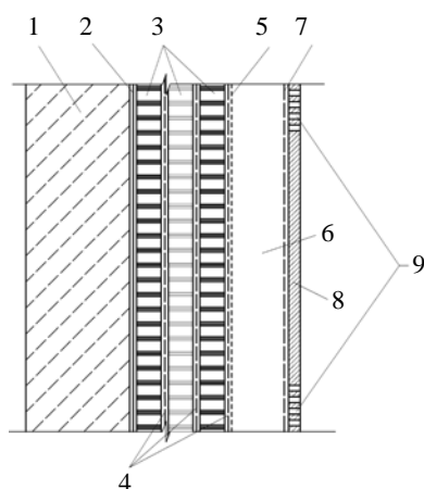
Рис. 1. Вертикальное сечение фрагмента стеновой панели
