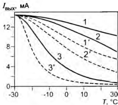
Рис. 2. Температурная чувствительность датчика на основе полоскового (кривые 1, 1'), щелевого (2, 2') и двойного щелевого (3, 3') волноводов с ЖК-заполнением при радиусах резонатора 16 и 32 мкм, соответственно сплошные и штриховые линии
