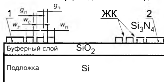
Рис. 1. Поперечное сечение кольцевого микрорезонатора на щелевых волноводах:
