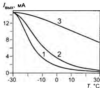
Рис. 4. Температурная чувствительность датчика на основе двойного щелевого волновода с разнесением щелей 600 (1), 400 (2) и 200 (3) нм
