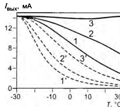
Рис. 3. Температурная чувствительность датчика на основе щелевого (сплошные кривые) и двойного щелевого (штриховые линии) волнопроводов в зависимости от ширины щели с ЖК-заполнением: 1, 1'—ширина щели 100 ( 2 \times 50 ) нм; 2, 2'—200 ( 2 \times 100 ) нм; 3, 3'—300 ( 2 \times 150 ) нм
