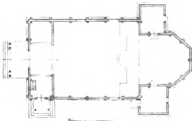
Рис. 1. План деревянной униатской церкви в д. Леонполь Витебской области. 1929 г. Арх. Б. Левко
