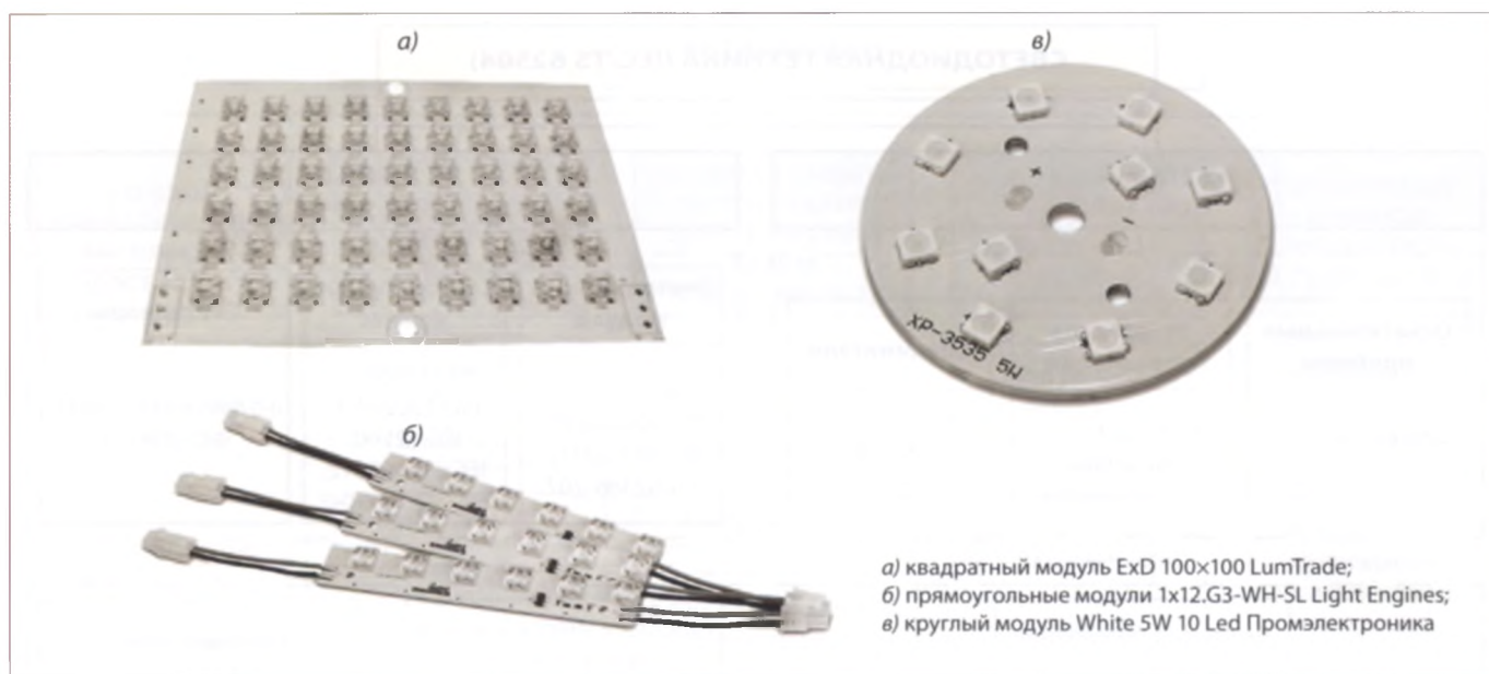
Рисунок 4 – Светодиодные модули
