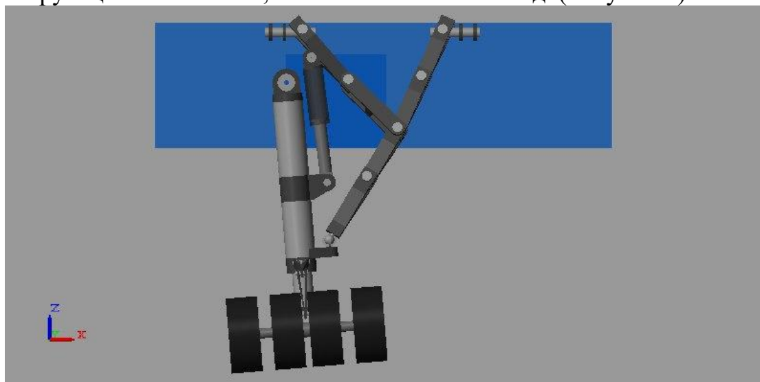
Рисунок 2. Структурные изменения модели – увеличение количества колес
