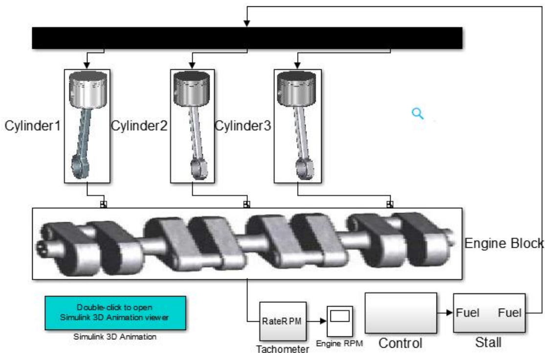
Рисунок 1 Структурное изменение модели – удаление цилиндра двигателя
