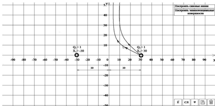
Рис. 13. Окно программы в режиме исследования электрического поля с помощью силовых линий
