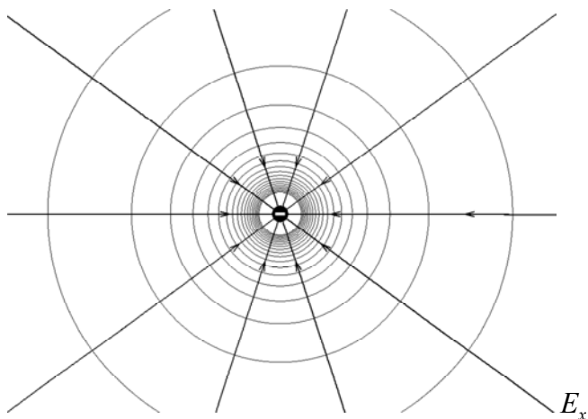
Рис. 4. Силовые линии и эквипотенциальные поверхности отрицательного заряда
