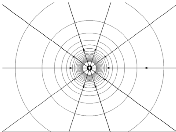
Рис. 3. Силовые линии и эквипотенциальные поверхности положительного заряда
