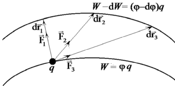
Рис. 5. Вектор силы Кулона и эквипотенциальные поверхности
