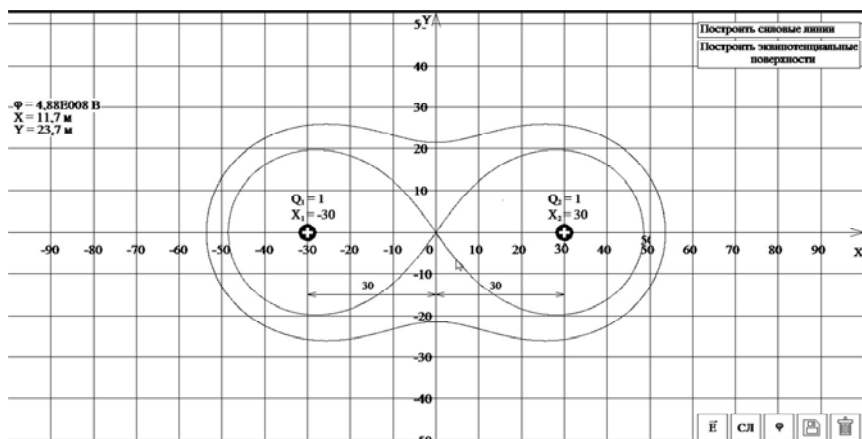
Рис. 14. Окно программы в режиме исследования электрического поля с помощью эквипотенциальных поверхностей
