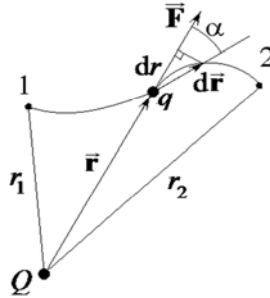
Рис. 2. К вычислению работы при перемещении заряда
