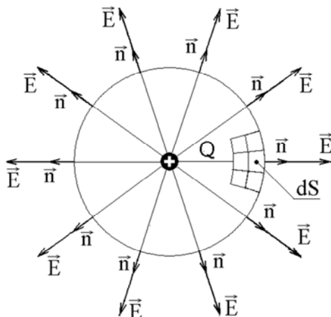
Рис. 7. К расчету потока вектора напряженности
