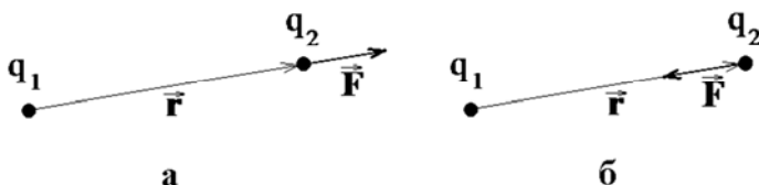
Рис. 1. К определению силы Кулона
