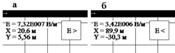
Рис. 12. Индикация слишком большого (а) и слишком малого (б) значений напряженности электростатического поля.
