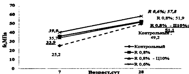
Рисунок 1 — Кинетика набора прочности бетона Составов 1.1-1.4
