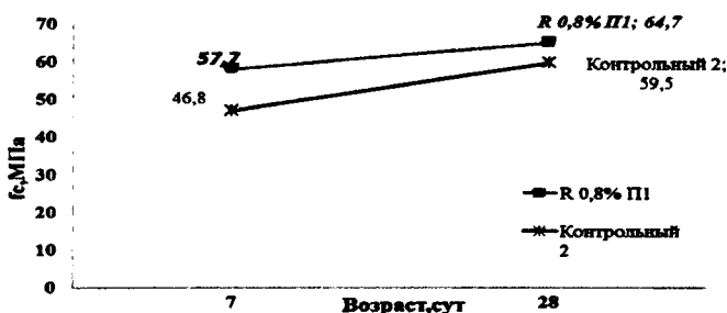
Рисунок 2 — Кинетика набора прочности бетона Составов 1.5-1.6
