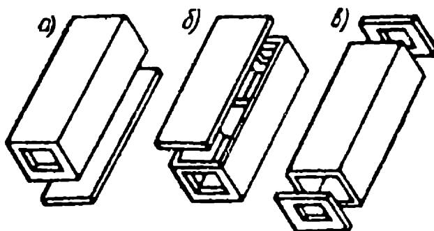
Рис. 4.29. Конструктивные решения объемных блоков
