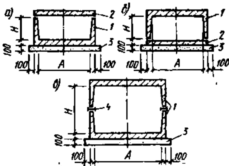
Рис. 6.21. Поперечные разрезы односекционного канала: 1 – лоток; 2 – плита; 3 – песчаная подготовка; 4 – швеллер
