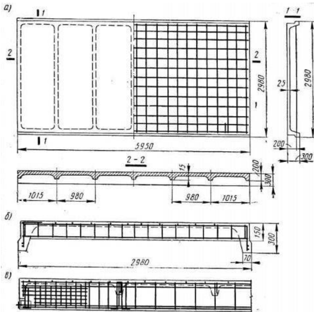
Рис. 5.20. Конструкция крупноразмерной панели покрытия 6×3 м: а – конструкция панели; б – армирование поперечного ребра; в – армирование продольного ребра
