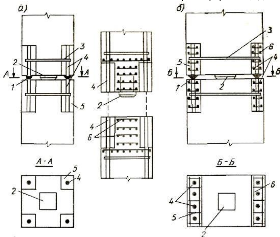
Рис. 4.19. Конструкция жесткого стыка колонн с ванной сваркой арматурных выпусков:
