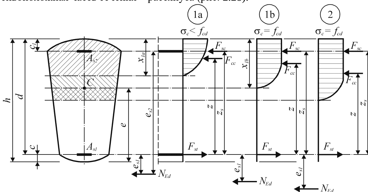
Рис. 2.28. Напряженно-деформированное состояние сечения растянутого элемента (случай больших эксцентриситетов)
