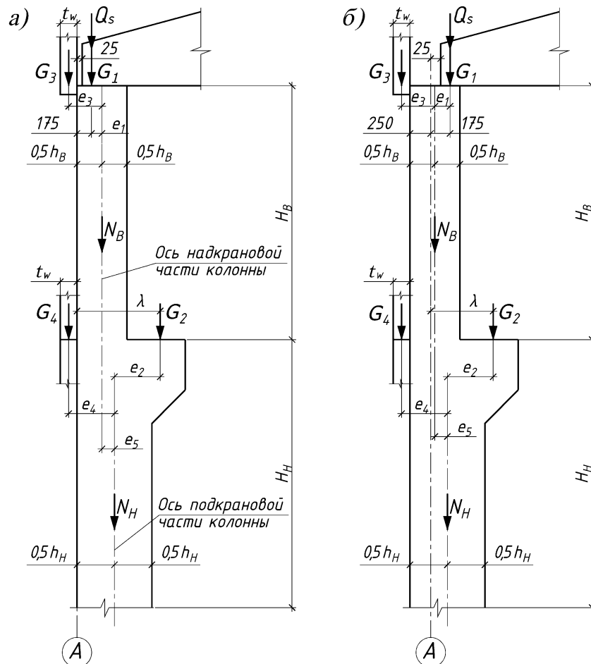
Рис 5.7. Схема для определения эксцентриситетов продольных сил в крайней колонне:
