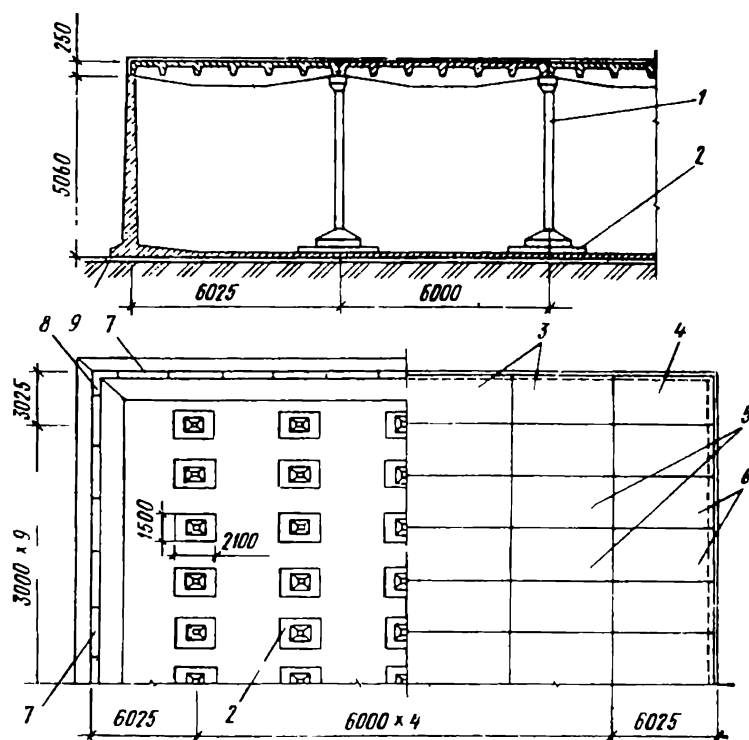
Рис. 6.3. Резервуар вместимостью 6000 м 3 с сеткой колонн 3×6 м и плоскими стеновыми панелями с пятой:
