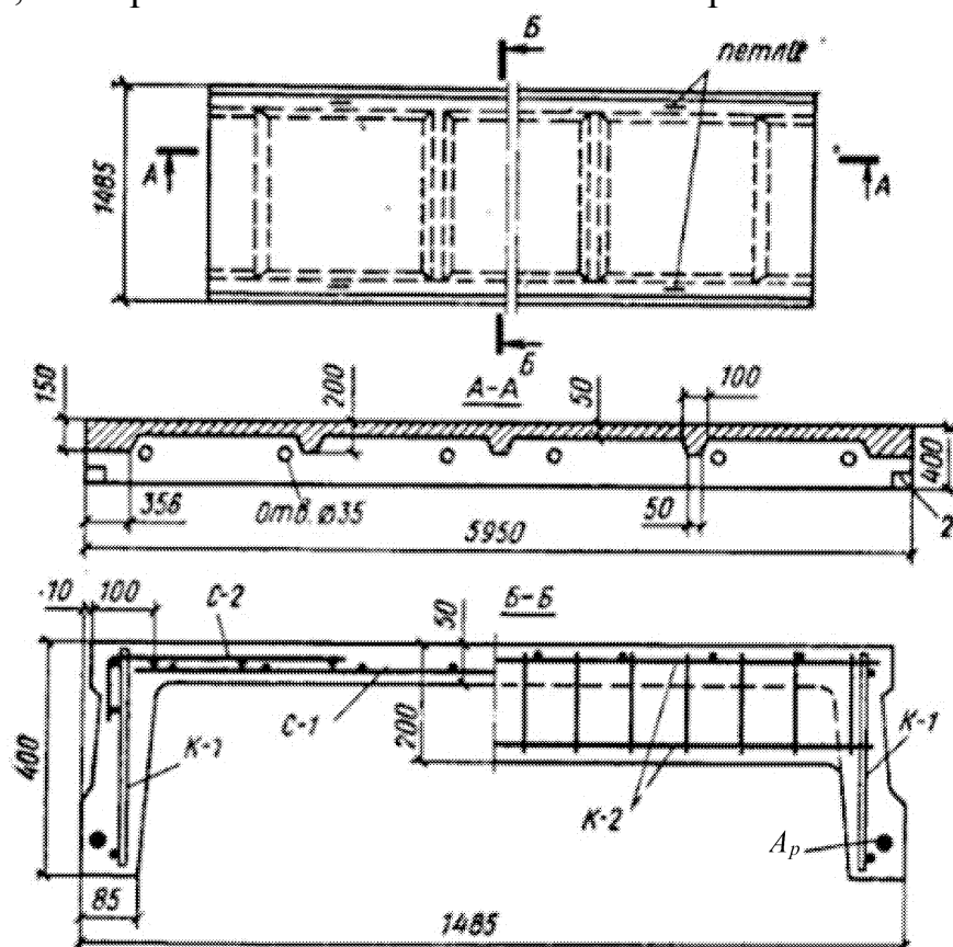
Рис. 4.38. Армирование ребристой плиты перекрытия
