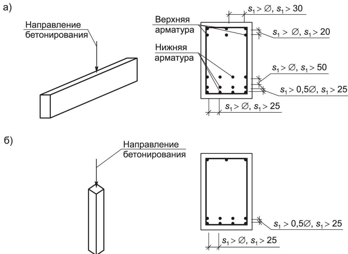
Рис. 1.14 (рис. 11.14 [7]). Минимально допустимые расстояния между стержнями продольной арматуры в зависимости от положения конструкции при бетонировании: а – горизонтальных элементов; б – вертикальных элементов
