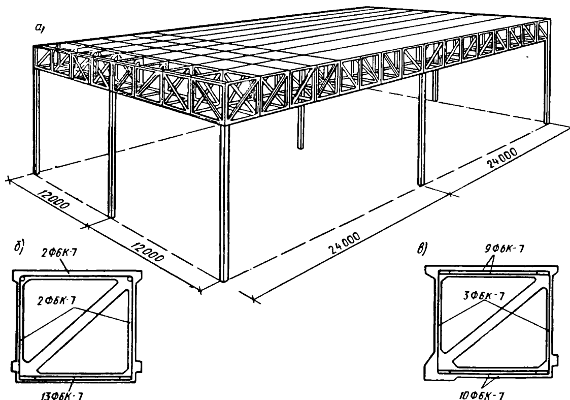
Рис. 5.40. Покрытие структурного типа из сборных железобетонных элементов заводского изготовления:
