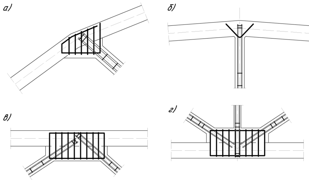
Рис. 5.27. Армирование узлов ферм а - в – верхнего пояса; г – нижнего пояса
