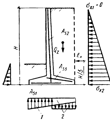
Рис. 6.18. К определению давления засыпки на подпорную стену в простейшем случае (1, 2 – эпюры)
