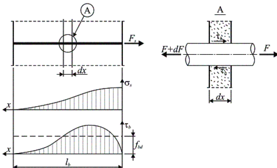
Рис. 1.15. К определению длины анкеровки l_b арматурного стержня
