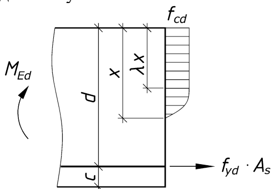
Рис. 1.23. Схема усилий в сечении с прямоугольной эпюрой напряжений в сжатой зоне бетона
