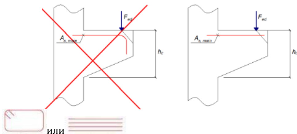
Рис. 5.10. Армирование консоли колонны
