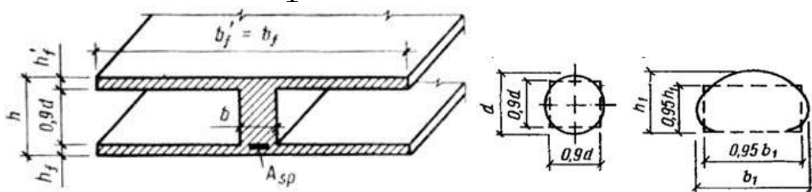
Рис. 4.36. Эквивалентные сечения плит для расчета прогибов
