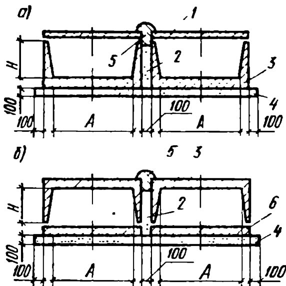
Рис. 6.22. Поперечные разрезы двухсекционных каналов: а – из лотковых элементов, перекрываемых плоскими плитами; б – то же, опирающихся на плоские плиты; 1, 6 – плиты; 2 – засылка песком; 3 – лоток; 4 – песчаная подготовка; 5 – цементный раствор
