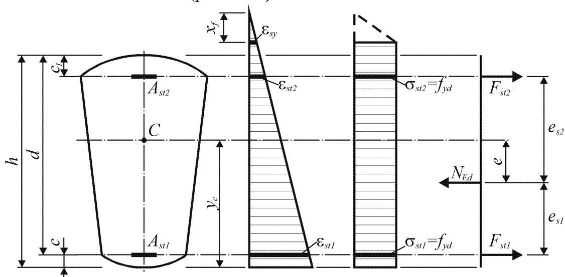
Рис. 2.27. Напряженно-деформированное состояние сечения растянутого элемента (случай малых эксцентриситетов)
