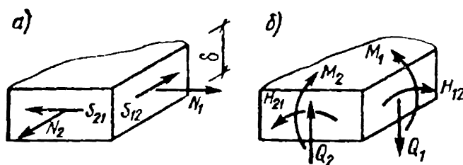
Рис 5.36. Напряженное состояние элемента оболочки: а – продольные и сдвигающие силы; б – изгибающие и крутящие моменты, поперечные силы
