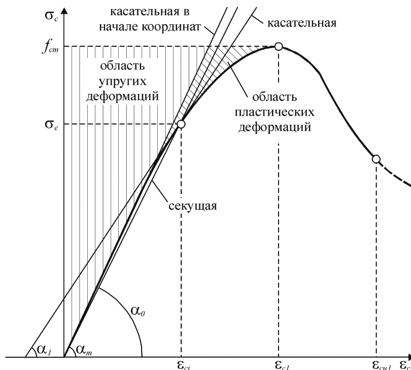
Рис. 1.7. К определению модуля деформаций бетона
