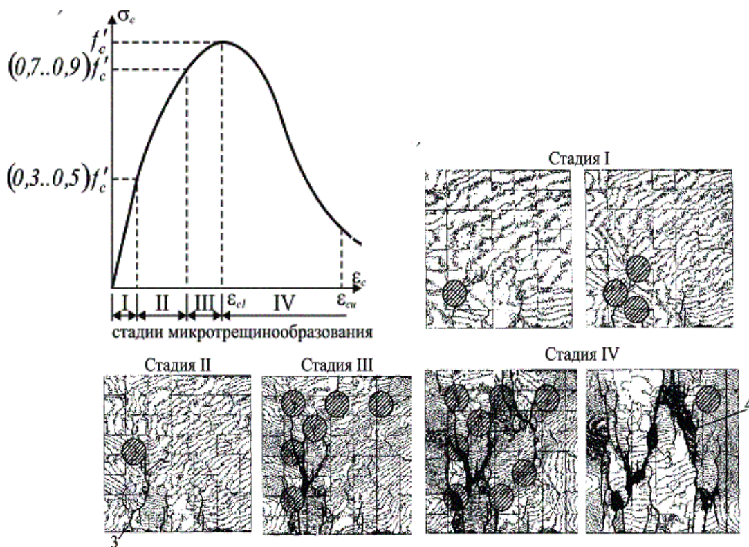
Рис.1.3. Формирование и развитие микротрещин в модельной структуре бетона 1 – контактные микротрещины; 2 – комбинированные микротрещины; 3 – микротрещины в растворной матрице; 4 – магистральная трещина
