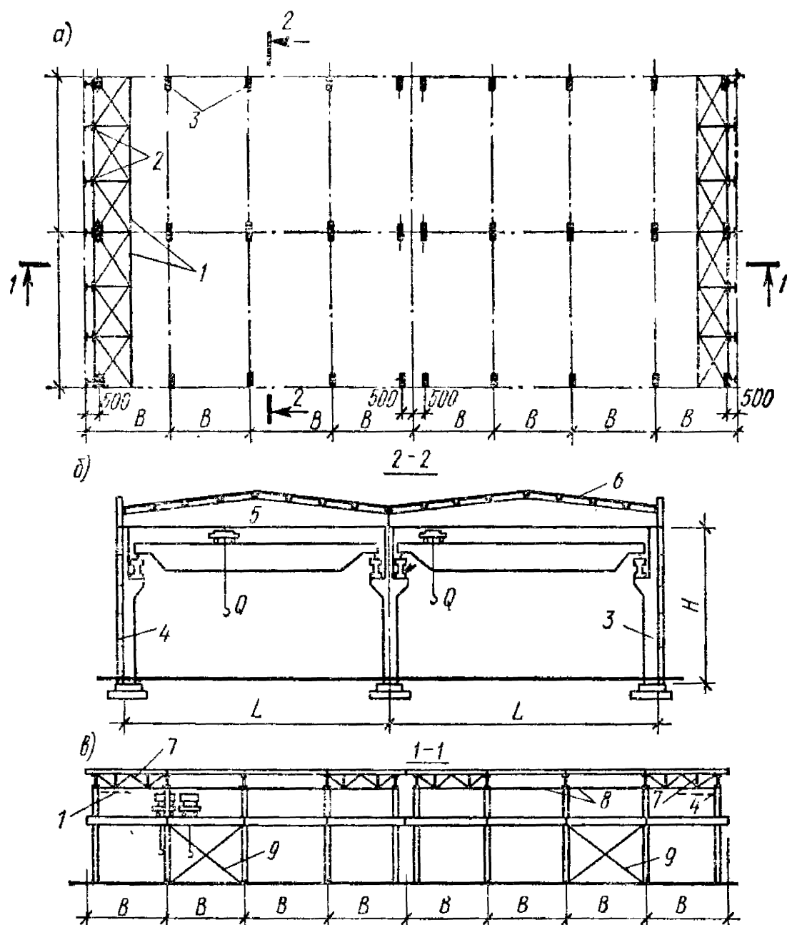
Рис. 5.1. Основные конструктивные элементы одноэтажного производственного здания:
