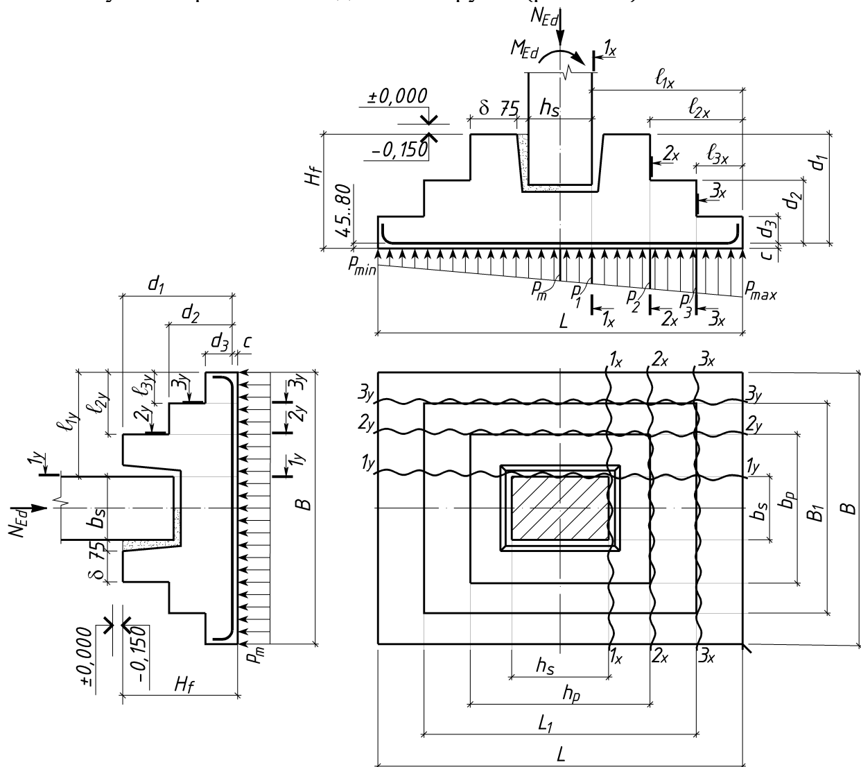
Рис. 4.49. К расчету внецентренно нагруженного фундамента
