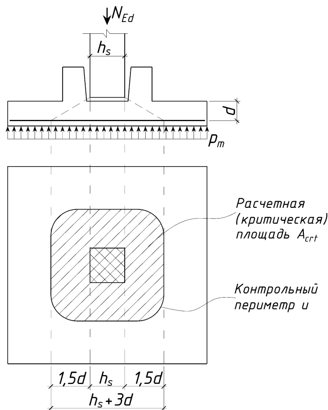
Рис. 4.48. Расчетная схема фундамента при проверке на продавливание
