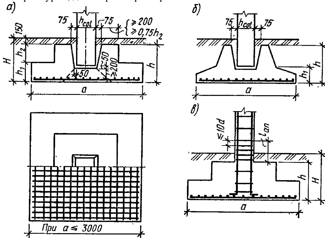
Рис. 4.42. Отдельные центрально нагруженные фундаменты: а – монолитный под сборную колонну; б – сборный под сборную колонну; в – монолитный под монолитную колонну
