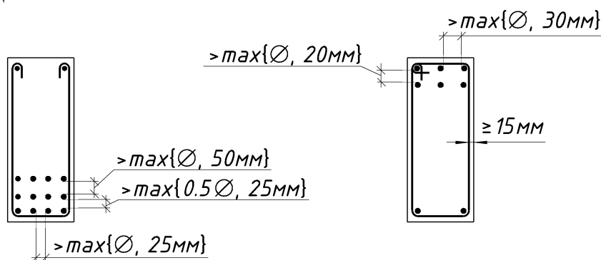
Рис. 2.5. Размещение продольной арматуры в сечении железобетонной балки
