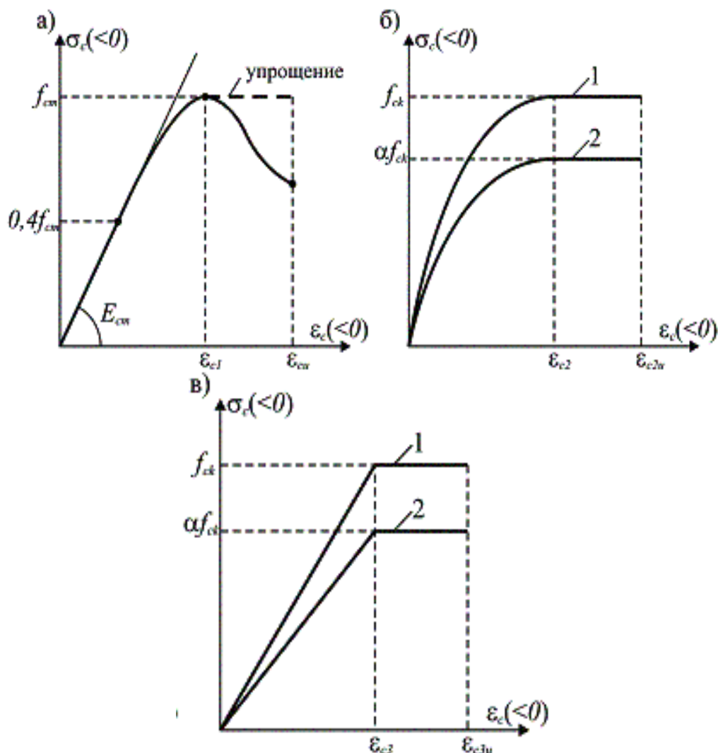
Рис. 1.8. Идеализированные диаграммы деформирования бетона а) полная идеализированная; б) упрощенная линейно-параболическая; в) упрощенная двухлинейная. 1 – нормативная; 2 – расчетная.
