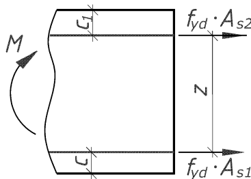
Рис. 2. Схема усилий в сечении колонны при подъеме
