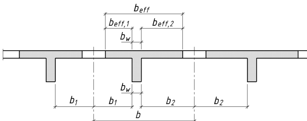
Рис. 2.12. Параметры эффективной ширины полки
