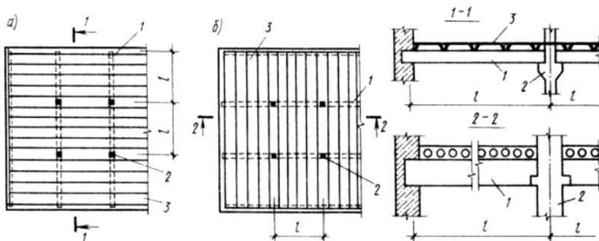
Рис. 4.8. Направление ригелей поперек (а) и вдоль (б) здания в сборном балочном перекрытии 1 – балка; 2 – колонна; 3 – панель
