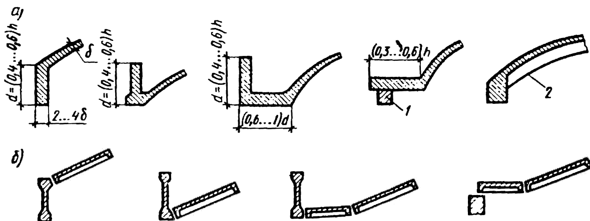
Рис. 5.34. Типы бортовых элементов цилиндрических оболочек:
