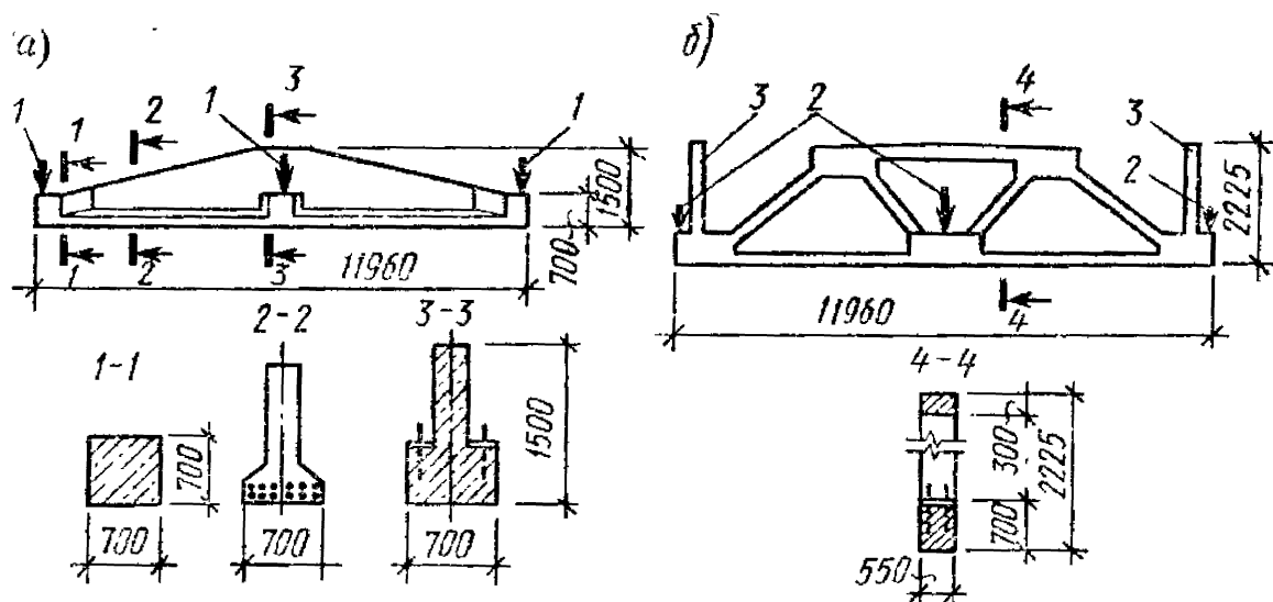
Рис. 5.28 Подстропильные балки (а) и фермы (б)
