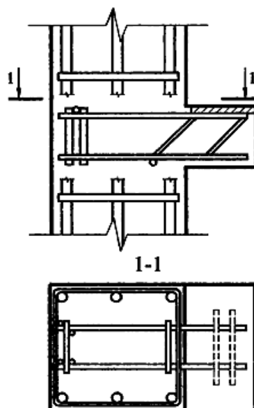
Рис. 4.20. Армирование консоли колонн при шарнирном опирании ригеля
