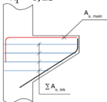
Рис. 5.11. К конструированию горизонтальных хомутов консоли
