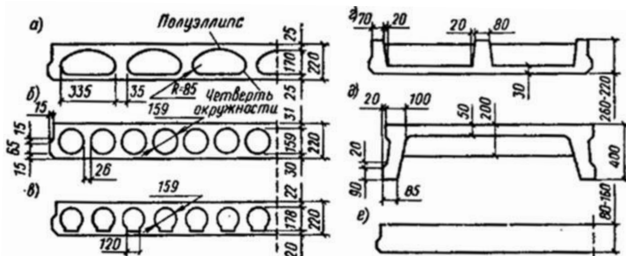
Рис. 4.34. Формы поперечного сечения плит перекрытий
