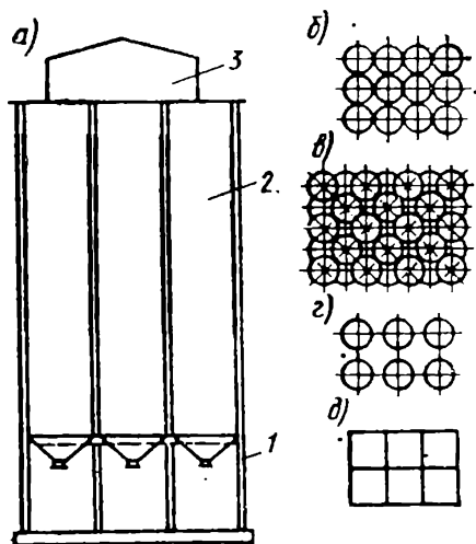
Рис. 6.11. Конструктивная схема силосных корпусов:
