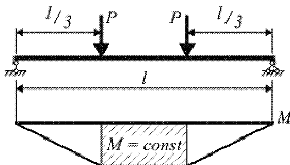
Рис. 1.16. Схема испытания опытной балки
