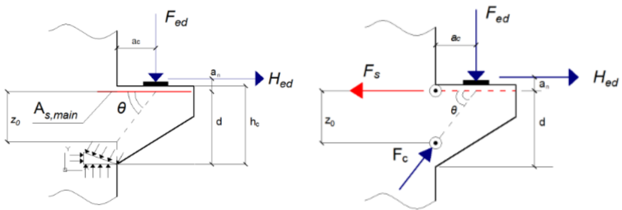
Рис.5.9. К расчету консоли:
