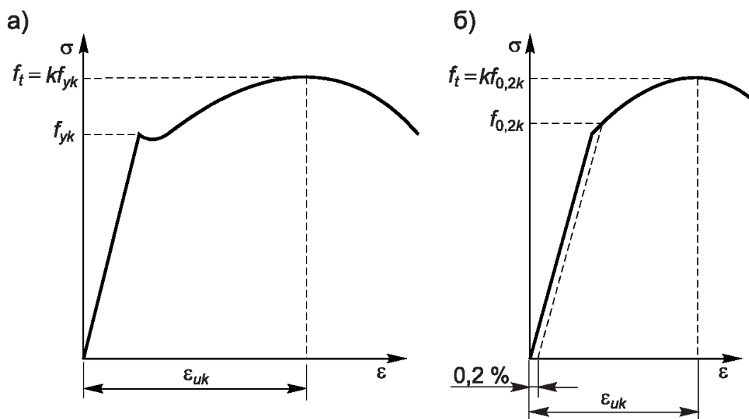
Рис. 1.10. Диаграммы деформирования арматурных сталей: а – горячекатанной; б – холоднодеформируемой
