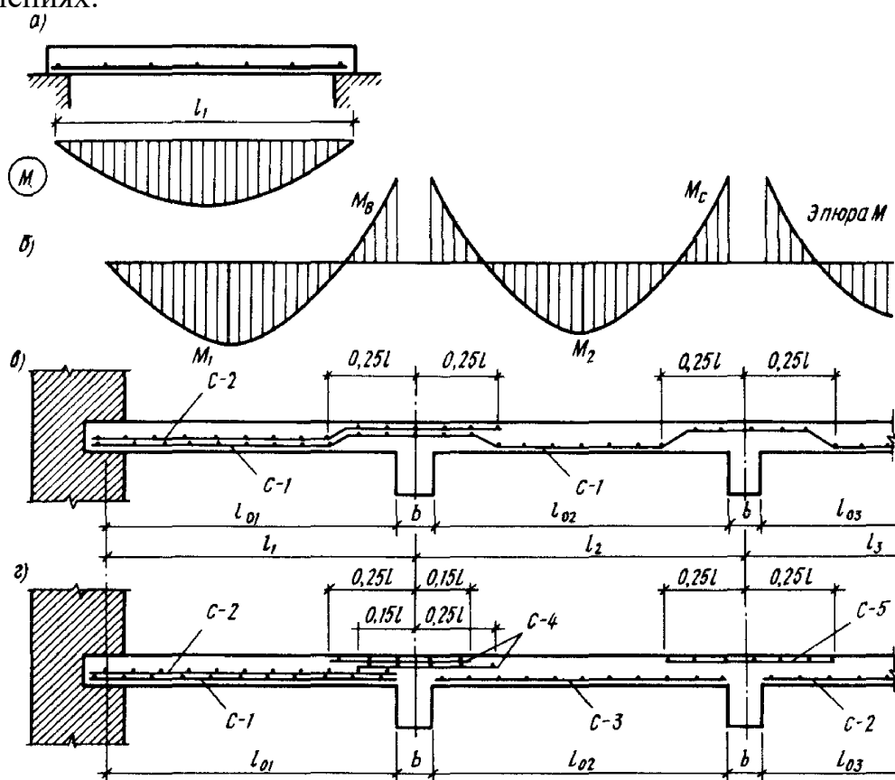
Рис. 2.2 Армирование железобетонных плит:
