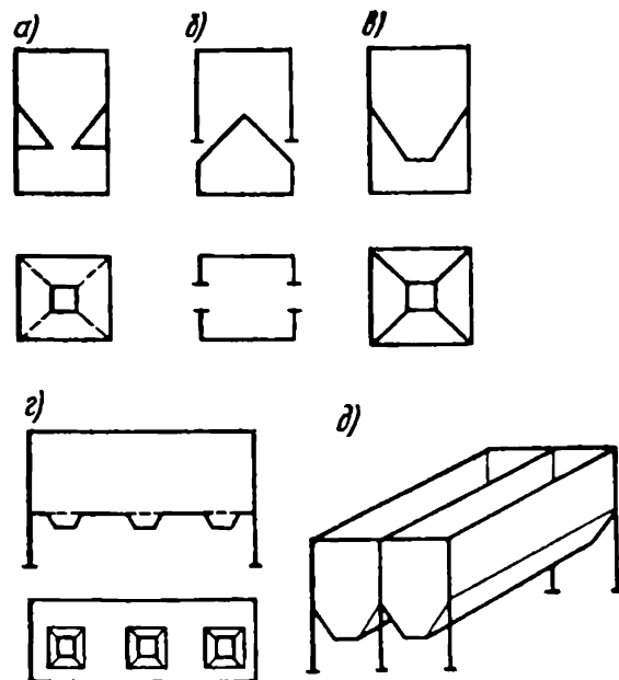
Рис. 6.7. Типы бункеров
