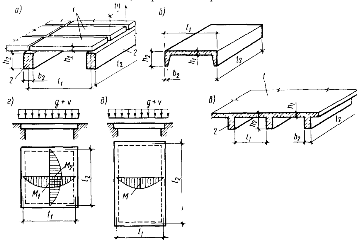
Рис. 2.1 Конструкции изгибаемых железобетонных элементов: а – сборное перекрытие; б – сборная плита; в – монолитное перекрытие; г – схема плиты, опертой по контуру; д – схема балочной плиты; 1 – плита; 2 – балка
