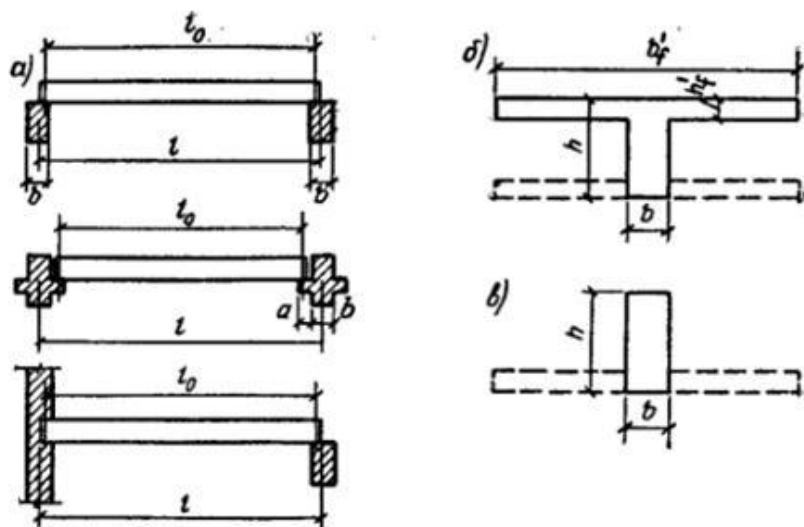
Рис. 4.35. Расчетные пролеты и сечения плит
