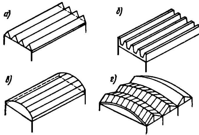
Рис. 5.29. Схемы призматических складок и складчатого свода: а – с треугольным поперечным сечением; б – то же, с трапециевидным; в – то же, со сводчатым; г – складчатый свод
