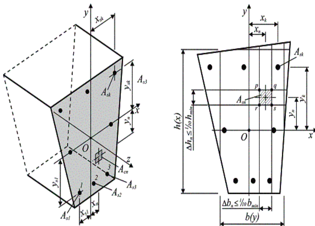
Рис. 1.25. Разбиение поперечного сечения на элементарные участки при расчете на действие изгибающих моментов и продольных сил
