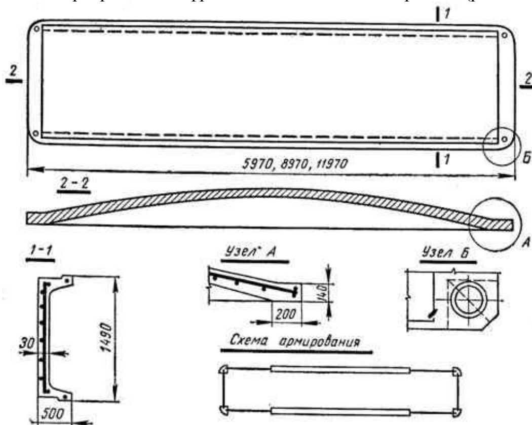
Рис. 5.22. Конструкция сводчатой крупноразмерной панели КЖС
