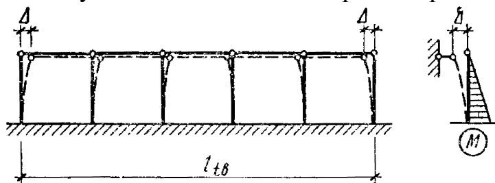
Рис. 5.4. Схема деформаций продольной рамы от температурных воздействий
