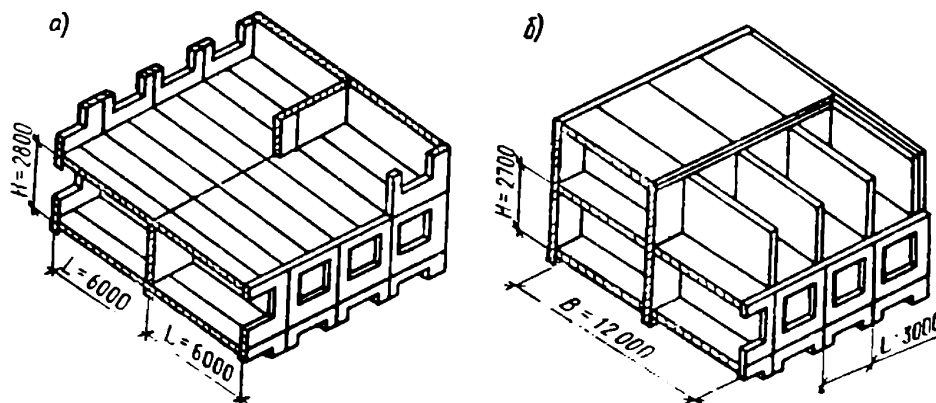
Рис. 4.27. Конструктивные схемы крупнопанельных зданий:
