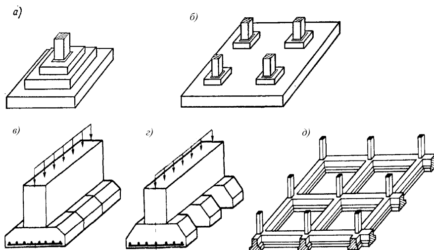
Рис. 4.41. Типы фундаментов
