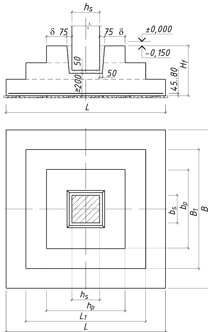
Рис. 4.45. Схема фундамента под колонну
