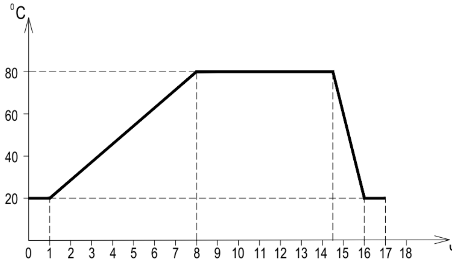
Рис. 1. График режима тепловлажностной обработки (пример)
