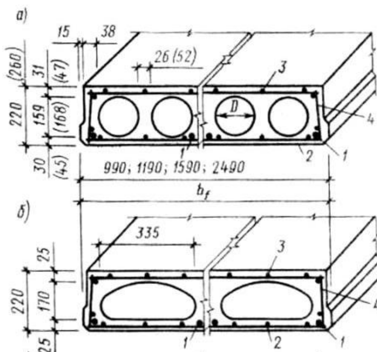
Рис. 4.37. Многопустотные панели с круглыми (а) и овальными (б) пустотами, 1 – продольная напрягаемая арматура; 2 – нижняя сварная сетка; 3 – то же, верхняя; 4 – вертикальный сварной каркас; 5 – то же, сетка
