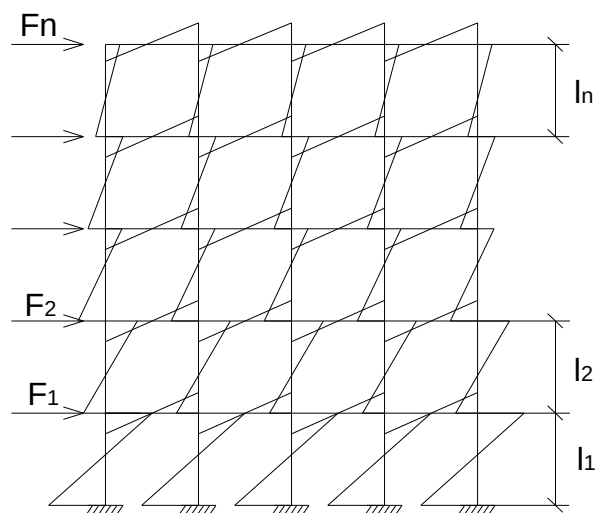
Рис. 4.10. К расчету многоэтажных рам на горизонтальные нагрузки
