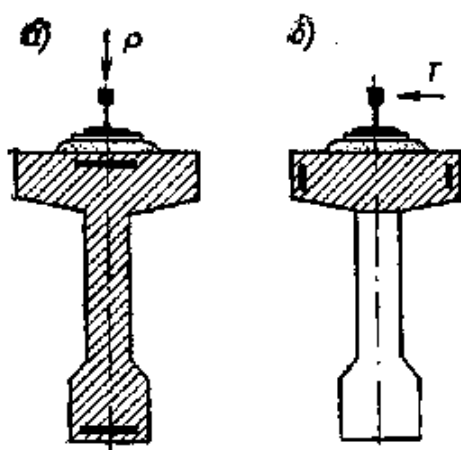
Рис. 5.13. Расчетные сечения подкрановой балки а – на вертикальную нагрузку; б – на горизонтальную нагрузку
