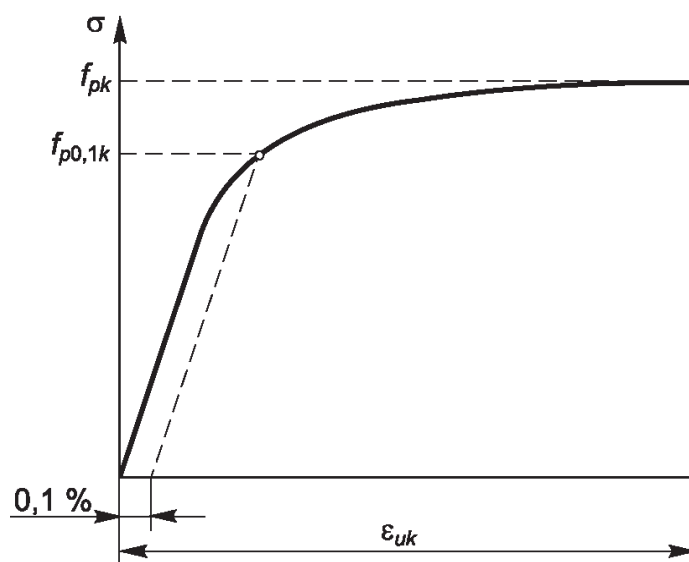
Рис. 1.11. Диаграмма деформирования для напрягаемой арматуры
