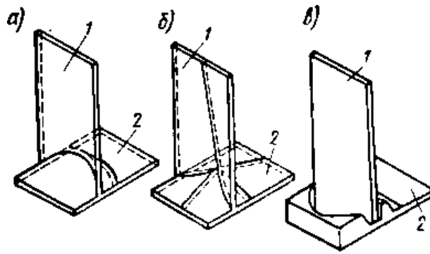
Рис. 6.17. Сборные подпорные стены-оболочки консольного типа:
