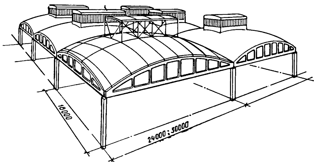
Рис. 5.38. Оболочки положительной гауссовой кривизны из плит размером 3 \times 6 м
