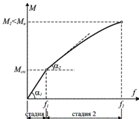
Рис. 1.18. Зависимость « M-f »
