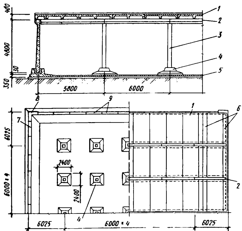
Рис. 6.1. Резервуар вместимостью 6000 м 3 с сеткой колонн 6×6 м:
