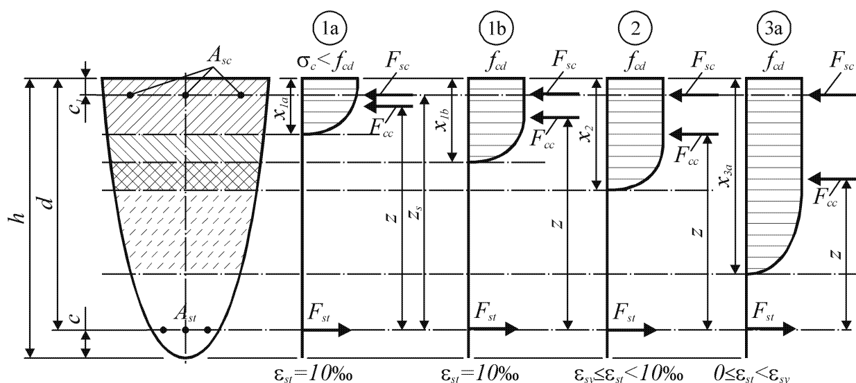
Рис. 1.26. Схемы усилий, действующих в расчетном сечении, для характерных областей деформирования 1, 2, 3
