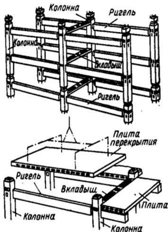
Рис. 4.1. Железобетонный каркас многоэтажного здания 1 – колонна; 2 – ригель; 3 – распорка; 4 – плита перекрытия
