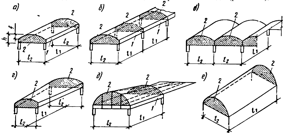
Рис. 5.30. Схемы оболочек и сводов нулевой гауссовой кривизны: а – цилиндрическая однопролетная; б – то же, многопролетная; в – то же, многоволновая; г – коническая; д – коноидальная; е – цилиндрический свод
