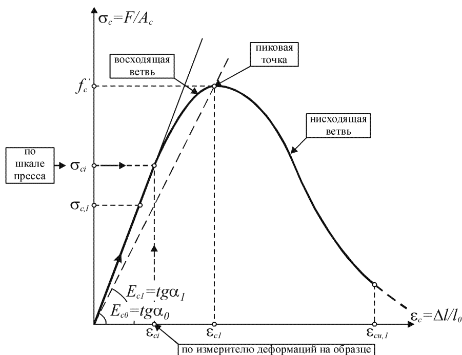
Рис. 1.6. Диаграмма деформирования бетона при кратковременном нагружении
