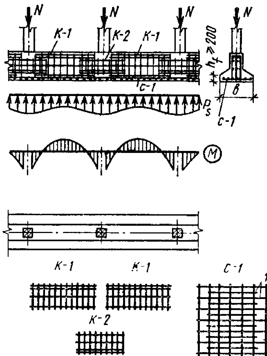
Рис. 4.54. Ленточные фундаменты под колонны: 1 – рабочая арматура
