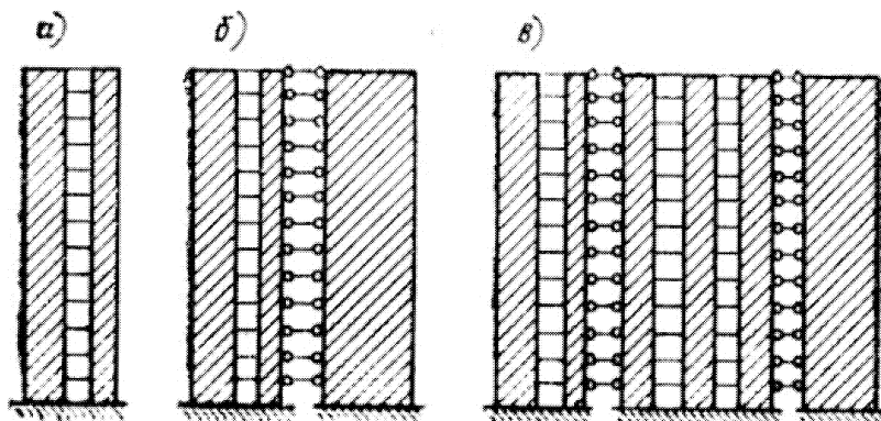
Рис. 4.12. Расчетные схемы связевых систем
