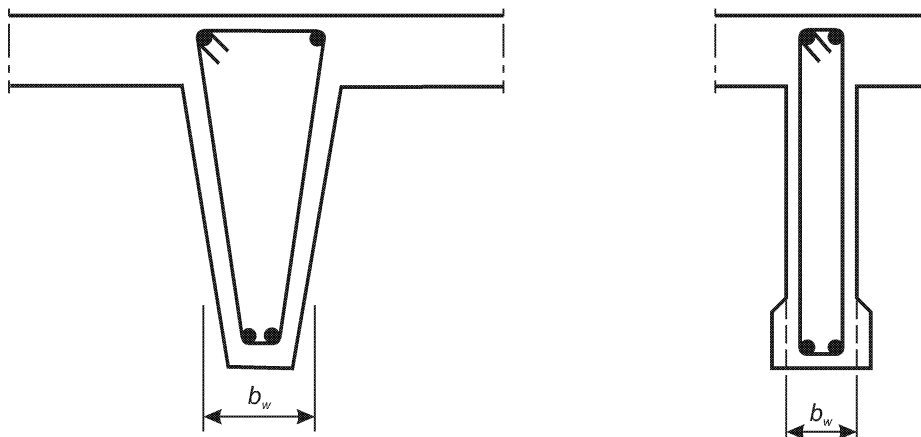
Рис. 2.16. К расчету прочности железобетонных элементов при действии поперечной силы по методу ферменной аналогии
