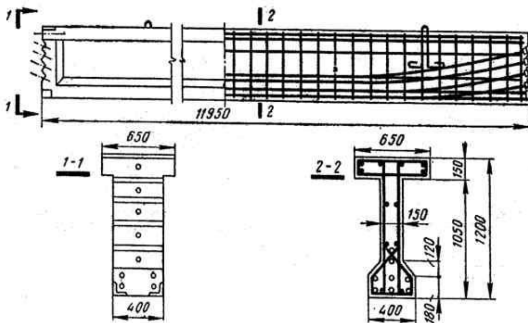
Рис. 5.14. Конструкция предварительно напряженной подкрановой балки пролетом 12 м.
