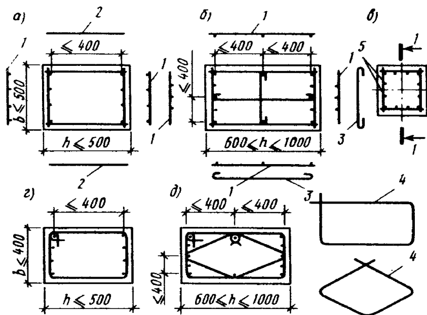
Рис. 2.25. Армирование сжатых элементов с гибкой арматурой а, б, в – сварными каркасами; г, д – вязаными; 1 – сварные каркасы; 2 – соединительные стержни; 3 – шпильки; 4 – вязанные хомуты;
