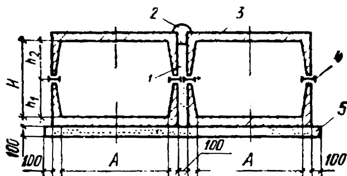
Рис. 6.23. Поперечный разрез двухсекционного канала из верхних и нижних лотковых элементов:
