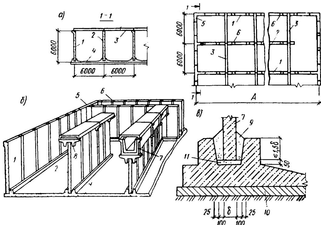
Рис. 6.4. Конструктивное решение аэротенка из железобетонных панелей: а – из панелей балочного типа; б – то же, консольного типа; в – узел сопряжения стеновых панелей с монолитным днищем; 1, 2 – стеновые и перегородочные панели; 3 – распорки через 6 м для восприятия горизонтальных усилия; 4 – монолитное железобетонное днище; 5 – монолитные участки несущих стен; 6 – шпоночные стыки между стеновыми и перегородочными панелями; 7 – прямоугольный лоток, перекрытый плитами; 8 – мостик для прохода и укладки технологических трубопроводов; 9 – бетон замоноличивания паза днища класса не менее C^{20}/_{25} ; 10 – бетонная подготовка из бетона класса C^8/_{10} ; 11 – выравнивающий слой цементного раствора (наносится в процессе монтажа стен)
