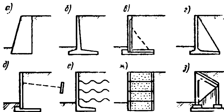
Рис. 6.15 Подпорные стены
