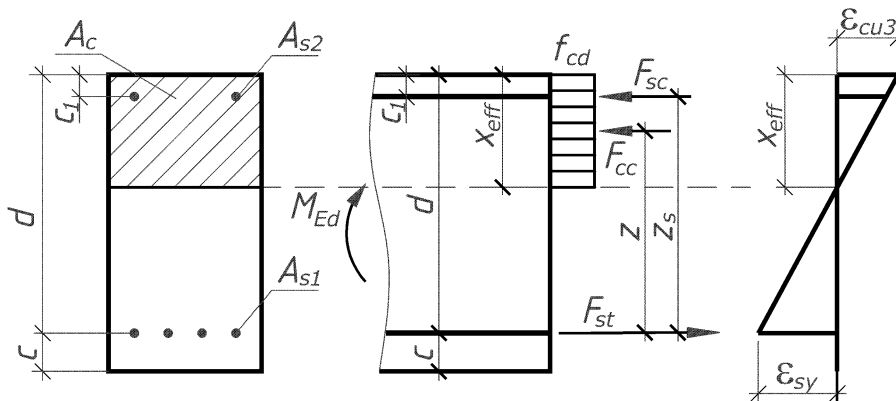
Рис. 2.8. Схема усилий и деформаций в сечении с двойным армированием при расчете методом предельных усилий
