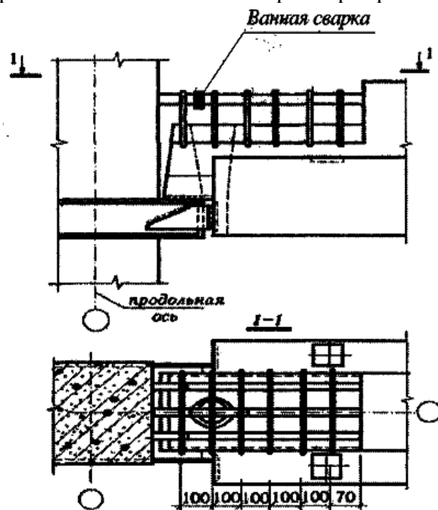
Рис. 4.20. Армирование консоли колонн при шарнирном опирании ригеля
