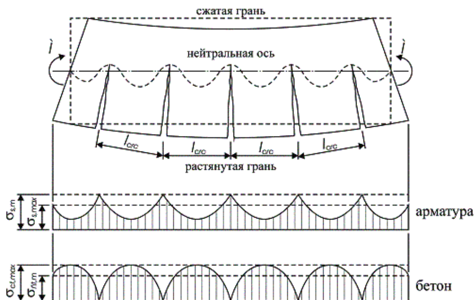
Рис. 1.19. Распределение напряжений в растянутой арматуре и растянутом бетоне для железобетонной конструкции в стадии 2
