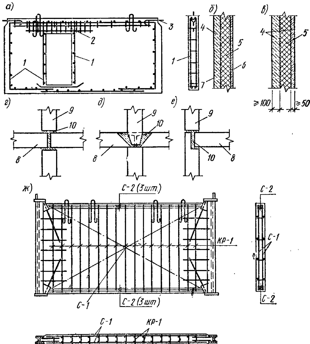
Рис. 4.28. Конструкции панельных зданий:
