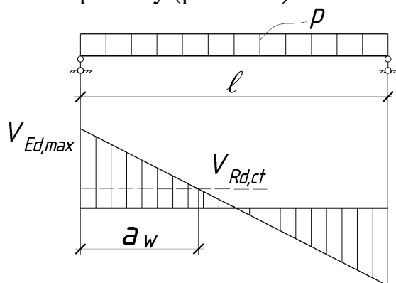
Рис. 2.17. К расчету наклонных сечений
