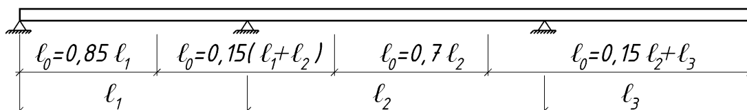
Рис. 2.11. Определение l_0 для расчета эффективной ширины полки
