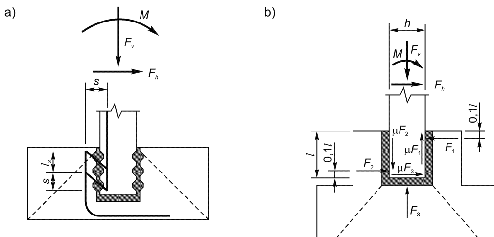
Рис. 4.50. Фундаменты стаканного типа: a – с профилированной поверхностью; b – с гладкой поверхностью Действующие напряжения и расчетная схема представлены на рис. 4.51.
