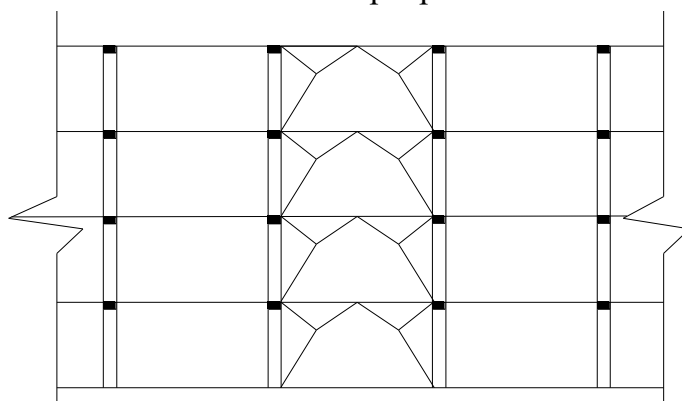
Рис. 4.4. Вертикальные связи многоэтажного каркаса в продольном направлении
