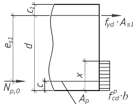
Рис. 2.22. К определению напряжений в бетоне при обжатии
