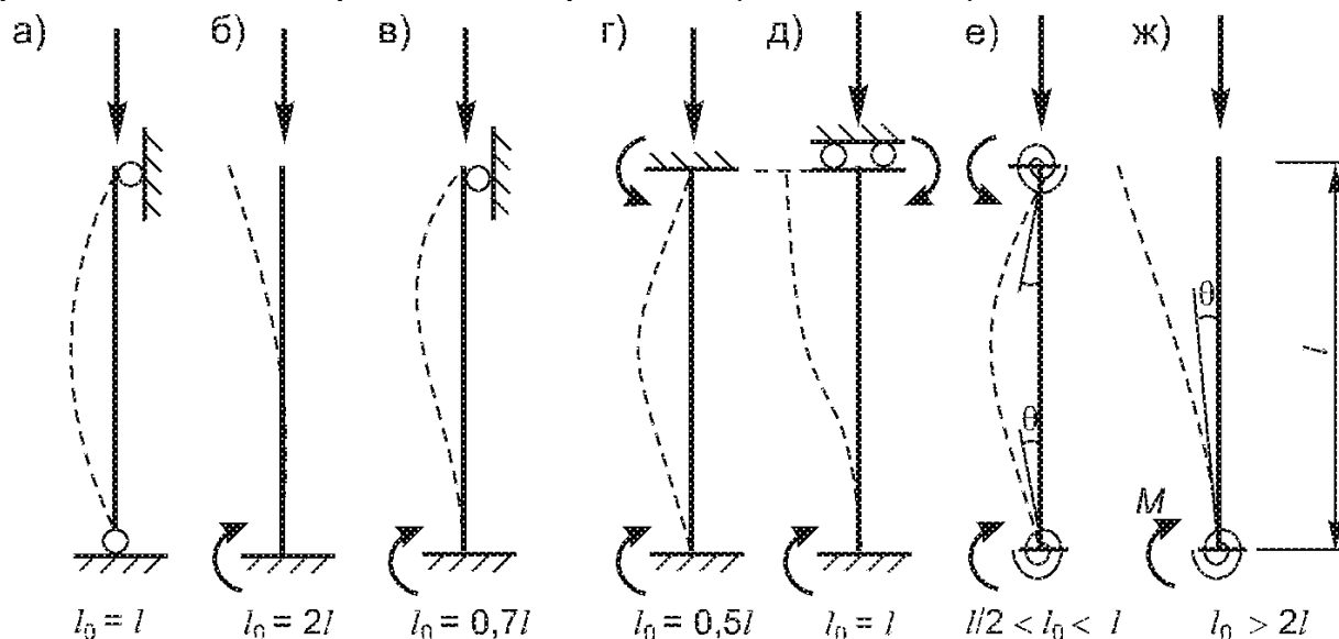
Рис. 2.26. К определению расчетных длин для отдельно стоящих элементов
