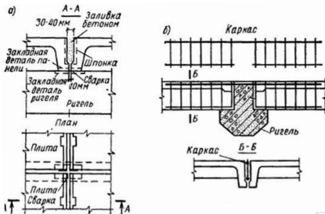
Рис. 4.39. Монтажные соединения плит
