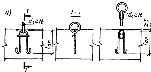
Рис. 7.4. Конструкция строповочной петли с убирающимся (падающим) стационарным кольцом (а) и с инвентарным кольцом (б)
