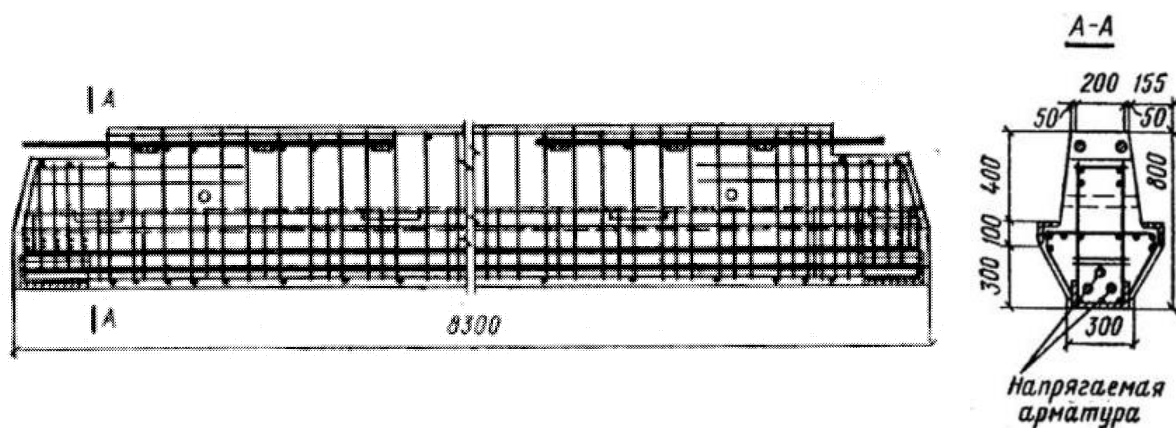
Рис. 4.14. Армирование ригеля поперечной рамы пролетом 9 м
