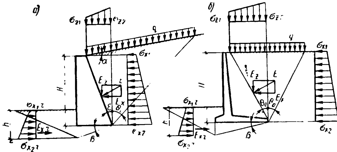
Рис. 6.19. Схема нагрузок на подпорную стену при расчете на устойчивость: а, б – соответственно массивных и консольных уголкового типа
