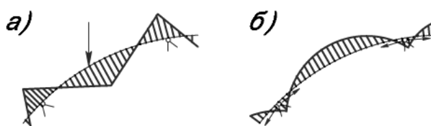
Рис.5.26. Эпюры моментов в верхнем поясе арочной фермы
