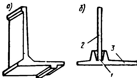
Рис. 6.16. Сборные подпорные стены уголкового типа:
