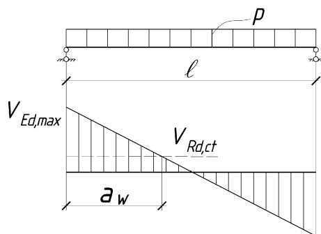
Рис. 1. К расчету наклонных сечений
