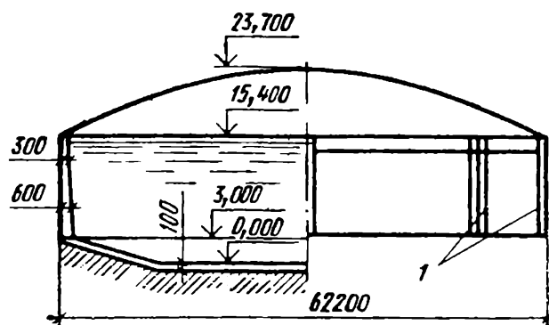
Рис. 6.6. Резервуар из предварительно напряженного железобетона вместимостью 45 000 м 3 (1 – пилястры для заанкеривания предварительно напряженной арматуры)
