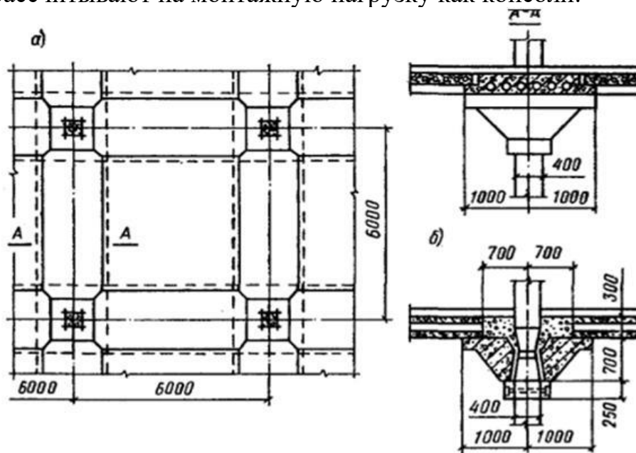
Рис. 4.32. Конструкция безбалочного сборного перекрытия с пустотными панелями:
