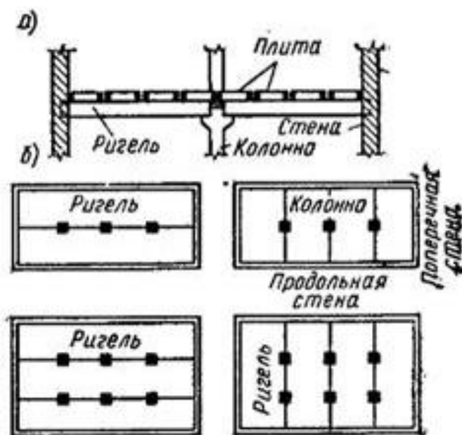
Рис. 4.33. Конструктивные схемы балочных перекрытий
