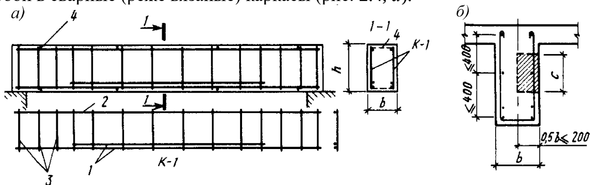
Рис. 2.4. Схема армирования железобетонной балки:
