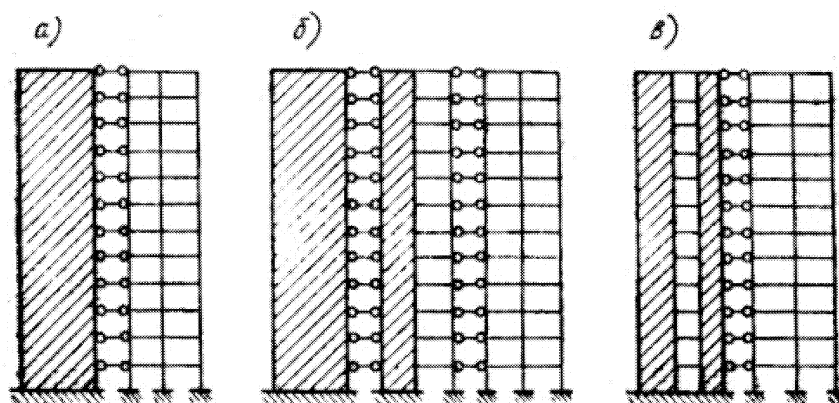
Рис. 4.11. Расчетные схемы рамно-связевых систем: а – со сплошной диафрагмой; б – со сплошной и комбинированной диафрагмами; в – с проемной диафрагмой
