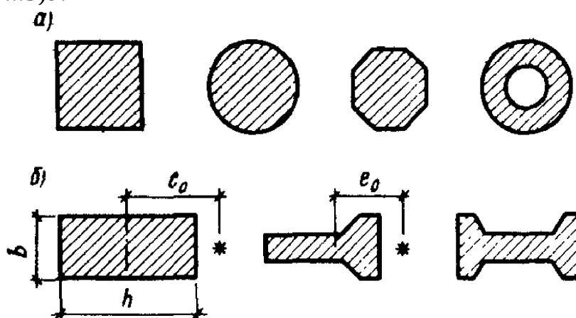
Рис. 2.23. Поперечные сечения внецентренно сжатых элементов
