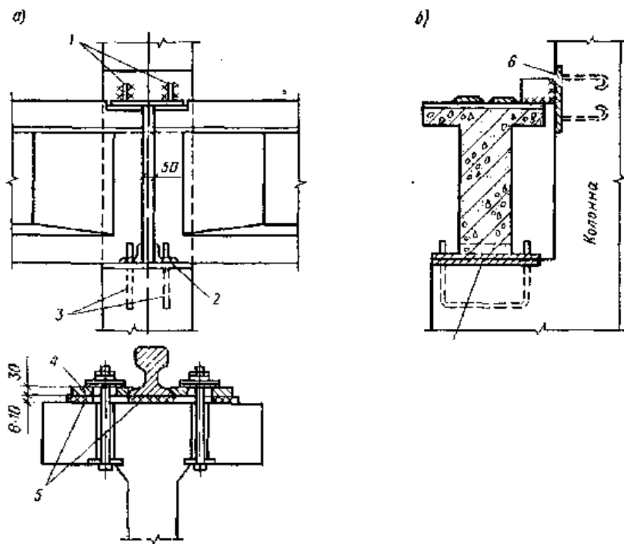
Рис. 5.16. Детали креплений
