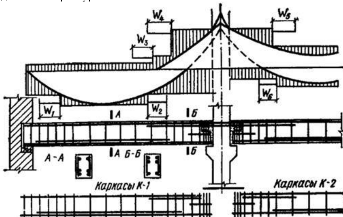
Рис. 4.26. Армирование ригеля и эпюра материалов
