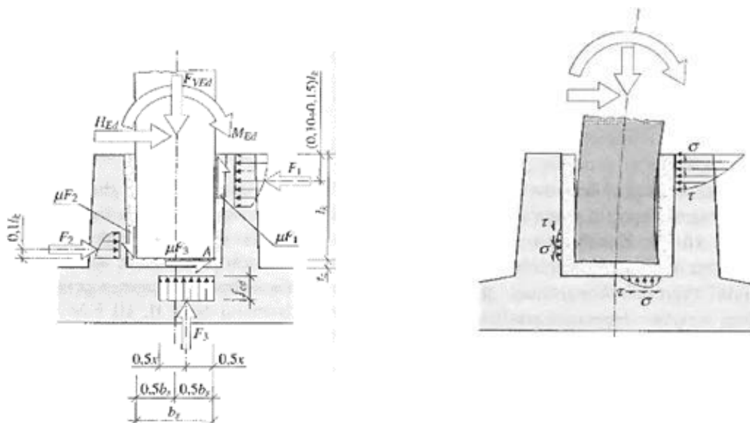
Рис. 4.51. Действующие напряжения и расчетная схема
