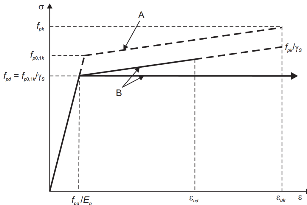
Рис. 1.13. Идеализированные диаграммы деформирования для напрягаемой арматуры: а – характеристическая; б – расчетная
