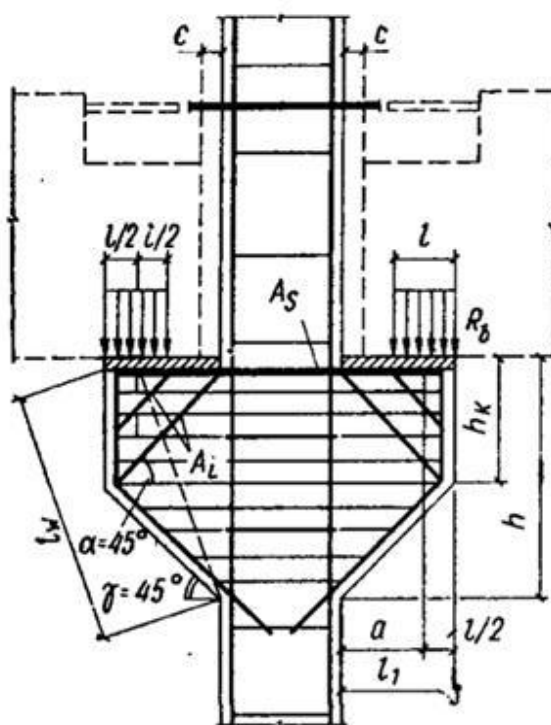
Рис.4.22. Армирование консоли колонны
