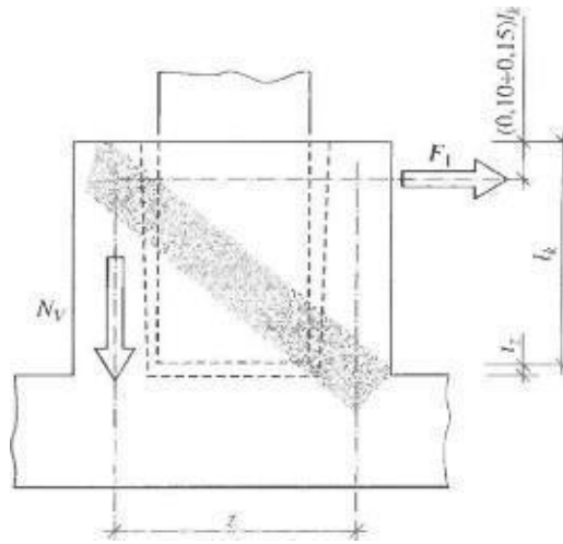
Рис. 4.52. Схема усилий для расчета вертикальной арматуры.
