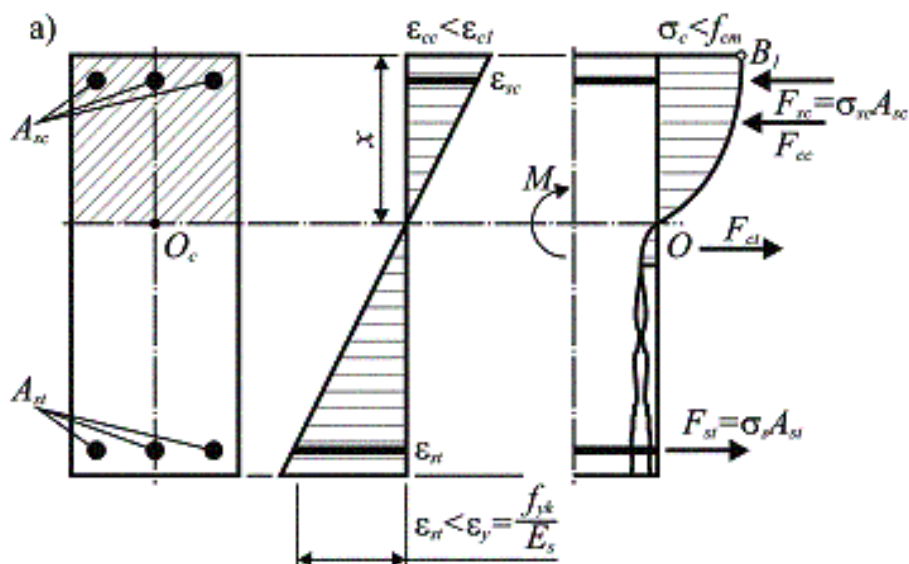
Рис. 1.20. Распределение напряжений и деформаций по высоте нормального сечения в стадии 2 напряженно-деформированного состояния
