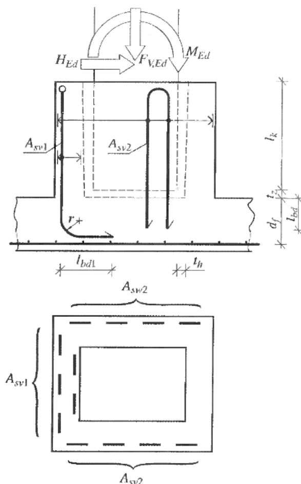
Рис. 4.52. К расчету вертикального армирования стакана
