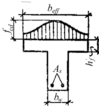
Рис. 2.10. Распределение сжимающих напряжений в полке
