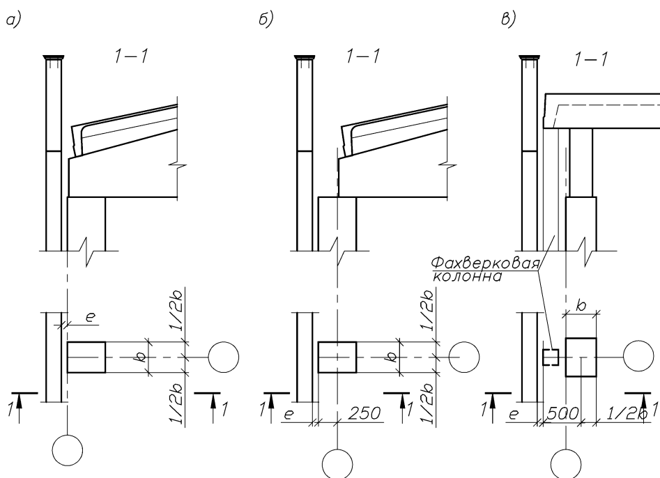
Рис. 5.2. Привязки колонн крайних рядов:
