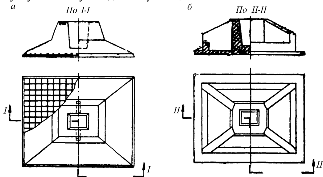
Рис. 4.43. Сборный одноблочный фундамент: а – пирамидальный; б – ребристый
