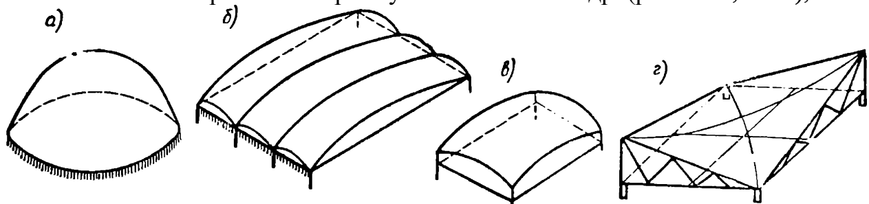
Рис. 5.31. Оболочки положительной ( а...в ) и отрицательной ( г ) гауссовой кривизны
