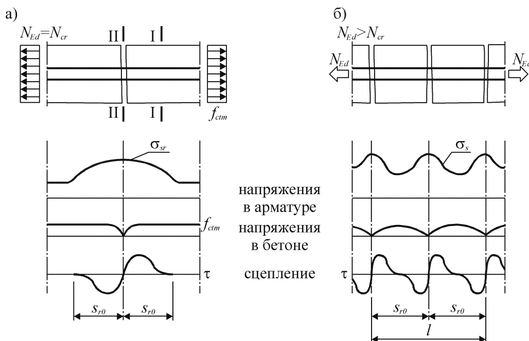
Рис. 3.1. Распределение напряжений в арматуре и бетоне центрально растянутого элемента:
