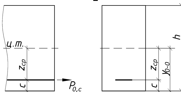
Рис.2. К определению z_{cp}
