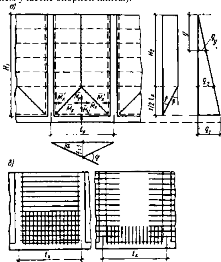
Рис. 6.20. К расчету передней стенки подпорной стены методом предельного равновесия
