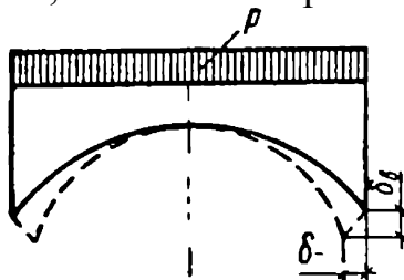
Рис. 5.33. Деформация поперечного сечения цилиндрической оболочки
