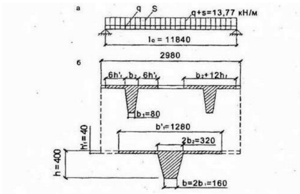
Рис. 5.21. Конструкция крупноразмерной панели покрытия 2Т
