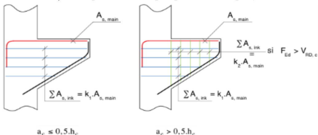
Рис. 5.12. К расчету армирования консоли вертикальными хомутами
