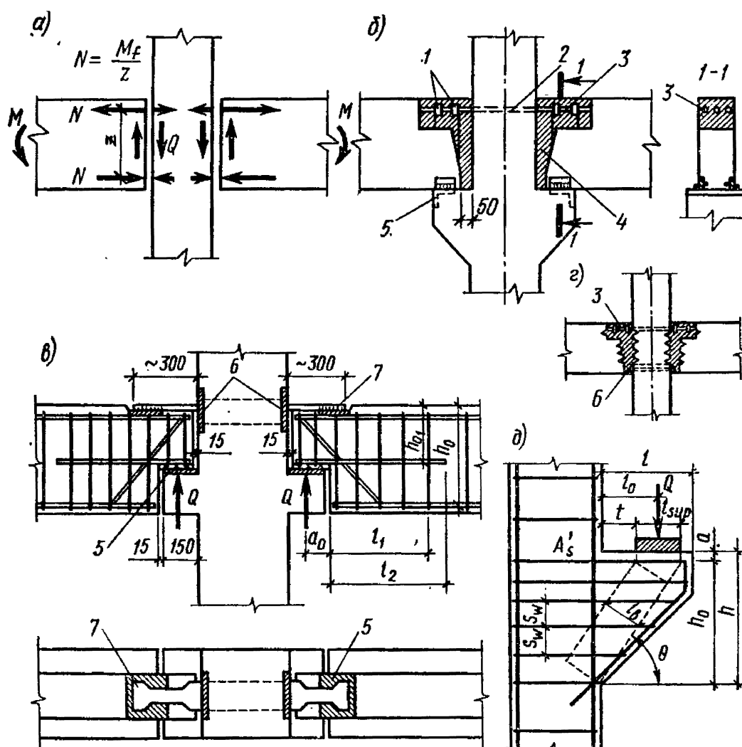
Рис. 4.17. Стыки ригелей с колоннами:
