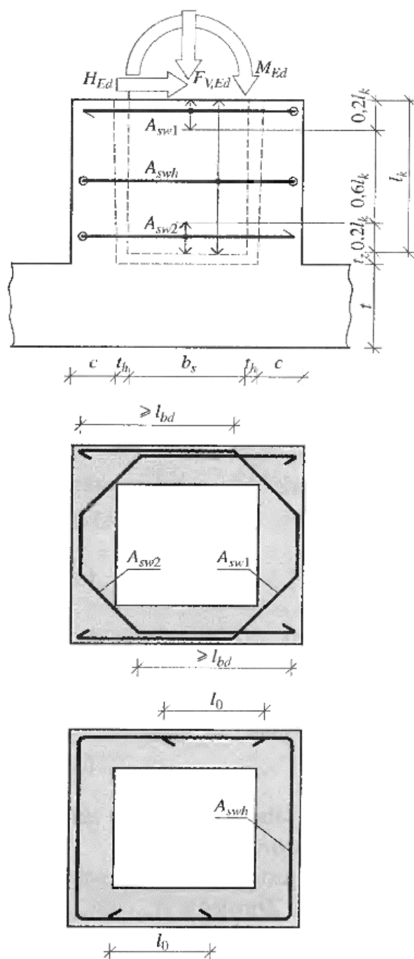
Рис. 4.51. К расчету горизонтального армирования стакана
