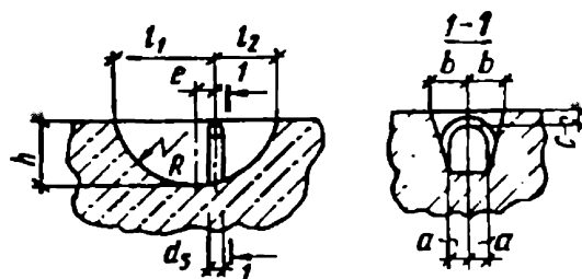
Рис. 7.3. Конструирование утопленной строповочной петли
