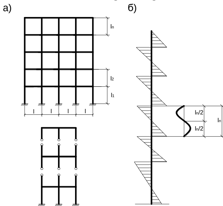
Рис. 4.9. Расчетные схемы многоэтажных рам (а) и эпюра моментов многоэтажной колонны (б)
