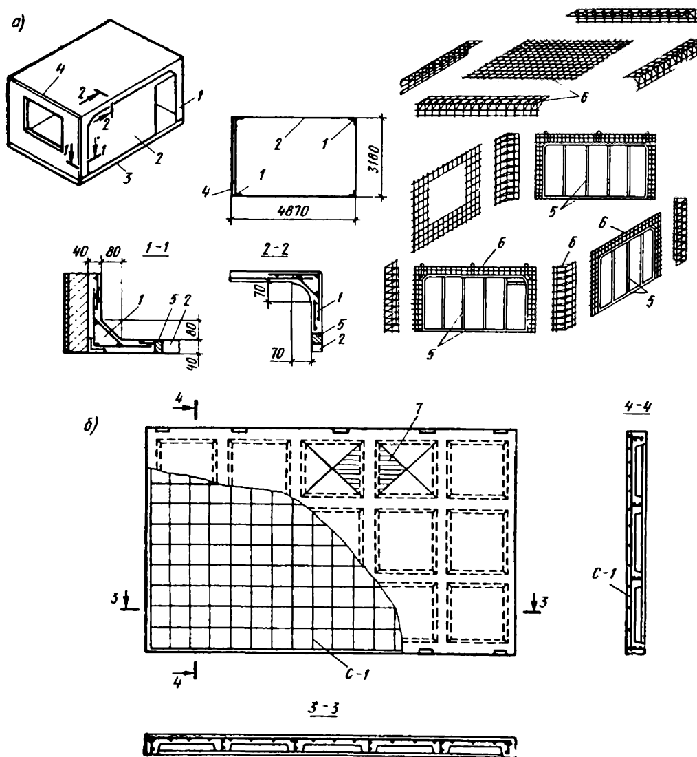
Рис. 4.30. Армирование блока типа «колпак»:
