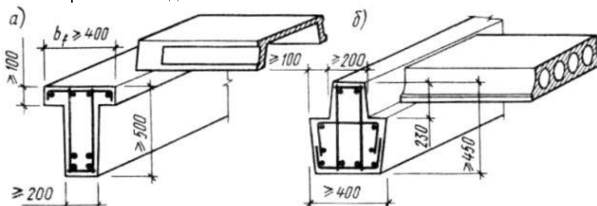
Рис. 4.23. Типы ригелей перекрытий промышленного (а) и гражданского (б) зданий
