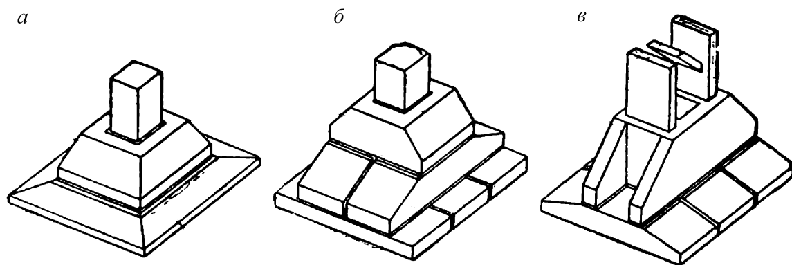
Рис. 4.44. Сборные многоблочные фундаменты:
