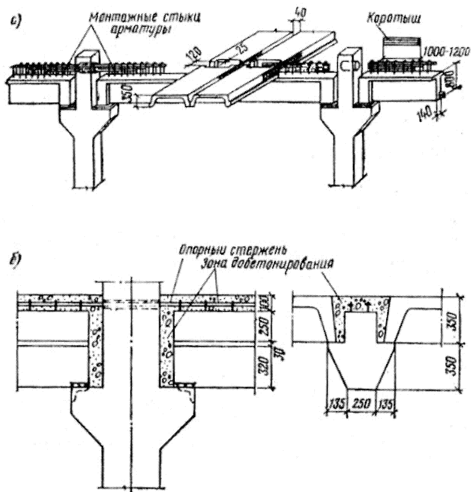
Рис.4.15. Конструкция узлов сборно-монолитной рамы а – до замоноличивания; б – после замоноличивания
