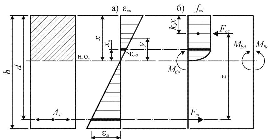
Рис. 2.7. Схемы распределения относительных деформаций (а) и напряжений (б) для прямоугольного сечения с одиночным армированием
