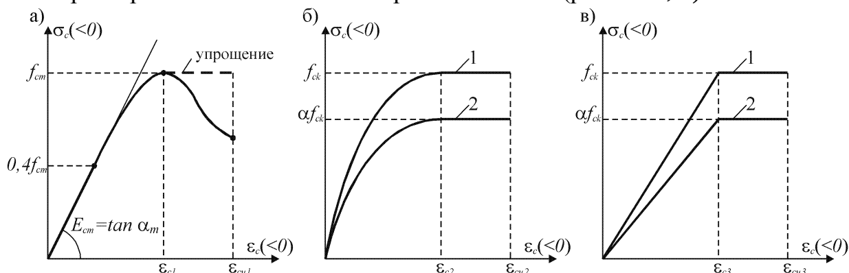
Рис. 1.24 Идеализированные диаграммы деформирования бетона:
