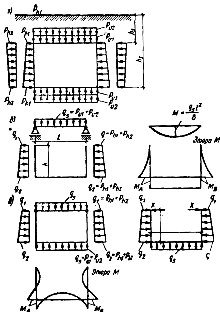
Рис. 6.24. К расчету каналов и тоннелей:
