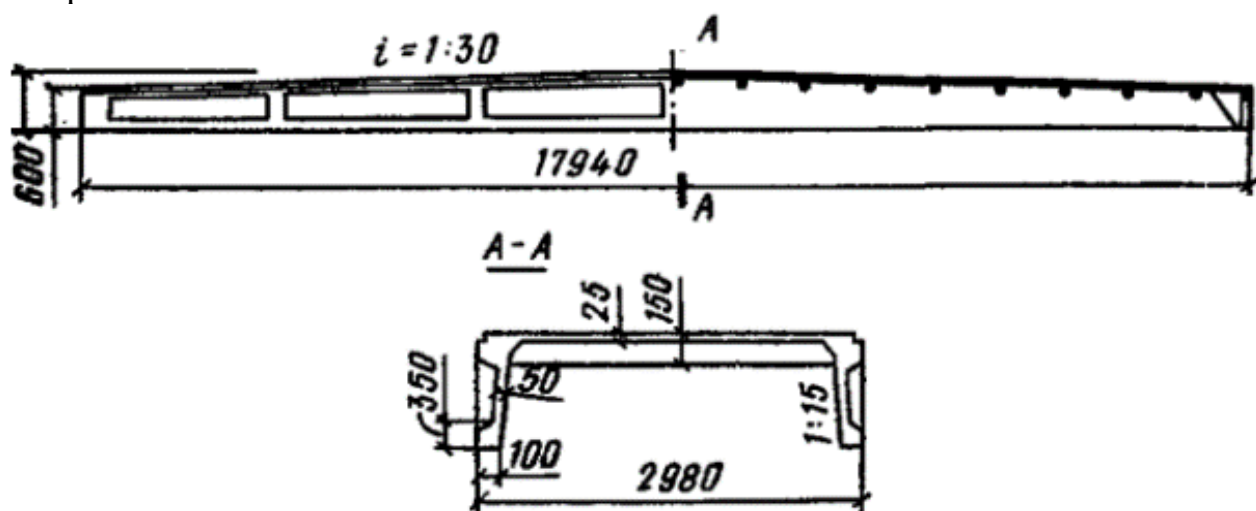
Рис. 5.23. Схема ребристой плиты покрытия под малоуклонную кровлю размером 3 \times 18 м
