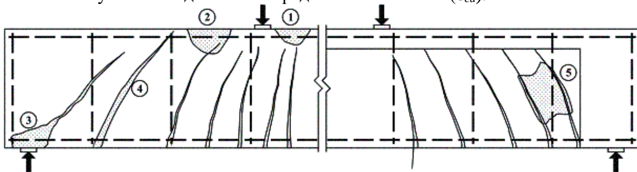
Рис. 2.15. Формы разрушения балки
