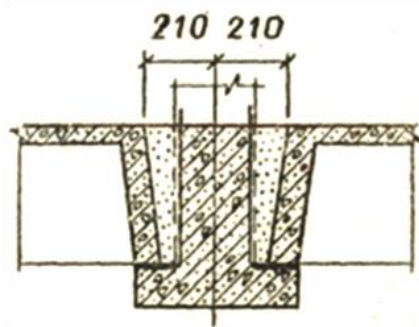
Рис. 4.7. Деталь опирания перекрытия на нижний пояс безраскосных ферм
