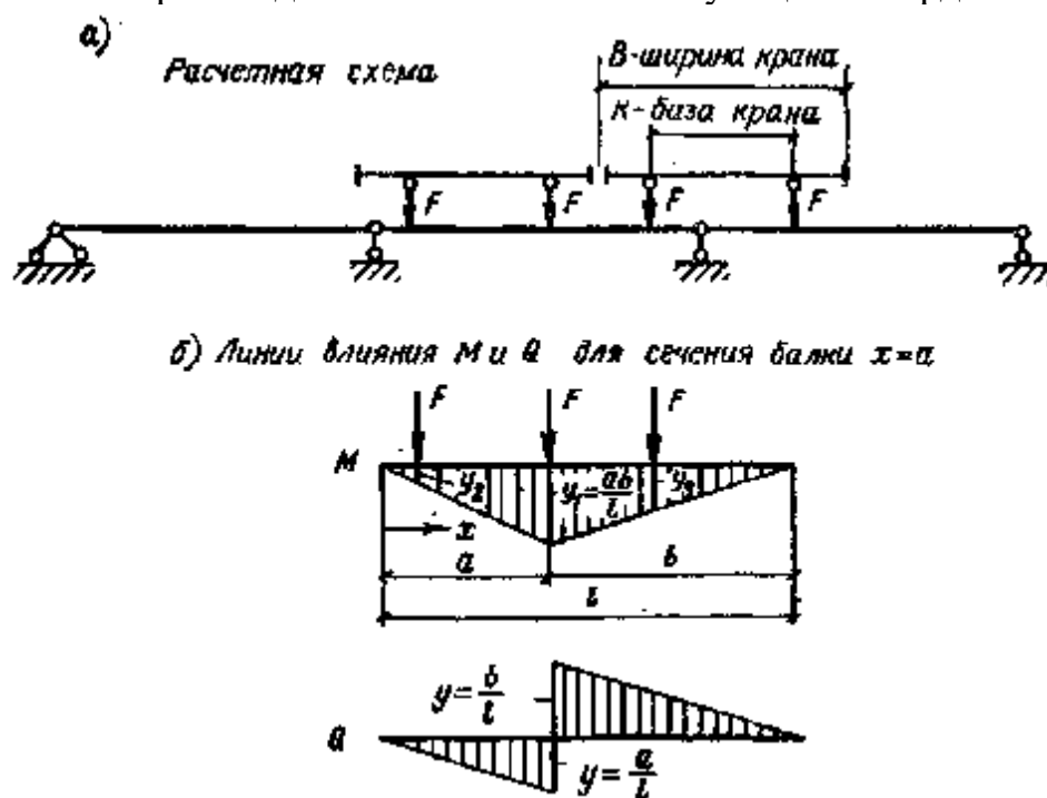
Рис. 5.15. К расчету подкрановой балки
