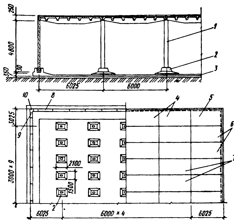
Рис. 6.2. Резервуар вместимостью 6000 м 3 с сеткой колонн 3×6 м и плоскими стеновыми панелями:
