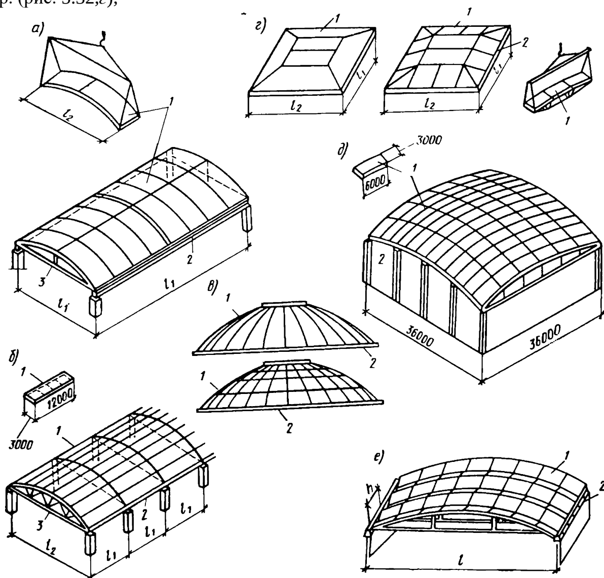
Рис. 5.32. Примеры членения сборных пространственных покрытий: а – длинная цилиндрическая оболочка из панелей размером 3×6 м, бортовых элементов и диафрагм, монтируемая из укрупненных элементов; б – то же, короткая из плоских панелей размером 3×12 м и диафрагм; в – оболочка вращения из трапециевидных криволинейных или плоских панелей; г – шатровая складка из плоских панелей; д – оболочка двоякой кривизны из панелей размером 3×6 м и укрупненных элементов размером 3×18 м; е – волнистый свод из плоских панелей; 1 – панель; 2 – бортовой элемент; 3 – форма-диафрагма;
