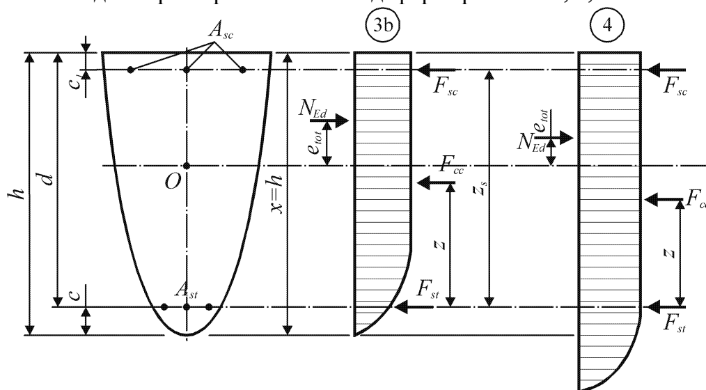
Рис. 1.27. Схемы усилий, действующих в расчетном сечении, для характерных областей деформирования 3b, 4
