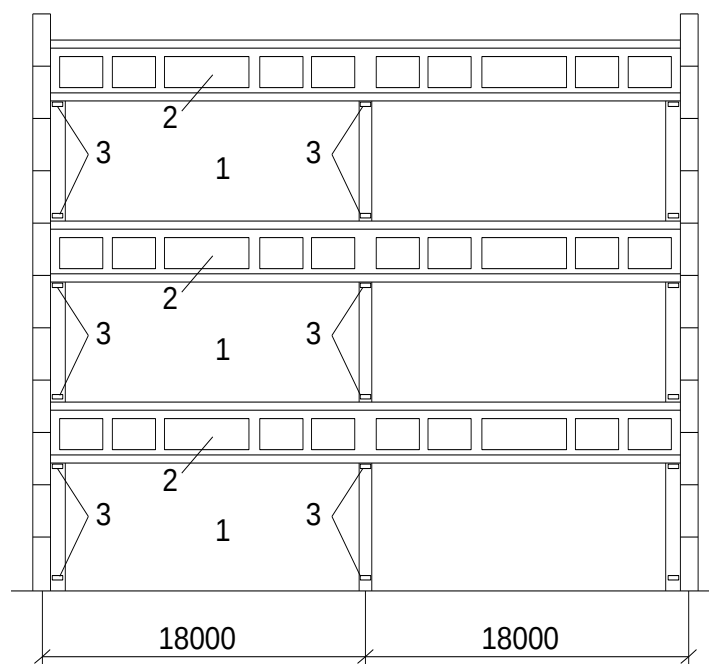
Рис. 4.6. Конструкция многоэтажного промышленного здания с межферменными этажами
