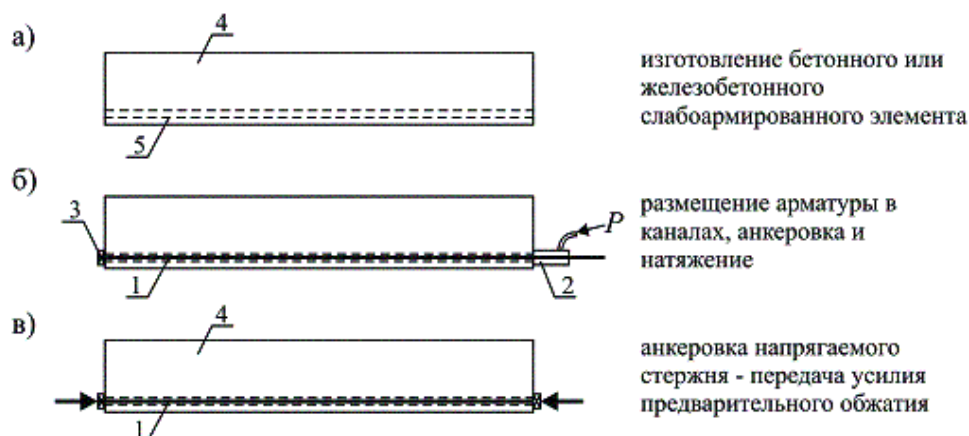
Рис. 2.20. Последовательность технологических операций при предварительном напряжении арматуры на бетон 1 – напрягаемая арматура; 2 – гидравлический домкрат двойного действия; 3 – анкер; 4 – бетонный элемент; 5 – канал или паз
