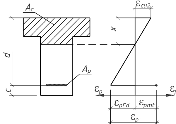
Рис. Распределение деформаций по высоте сечения
