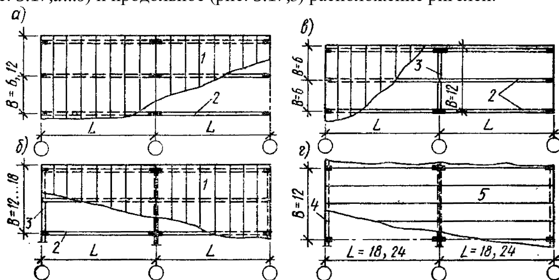
Рис. 5.17. Варианты компоновки покрытия (размеры в м):
