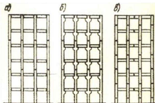
Рис. 4.13. Конструктивные схемы членения многоэтажных рам на сборные элементы
