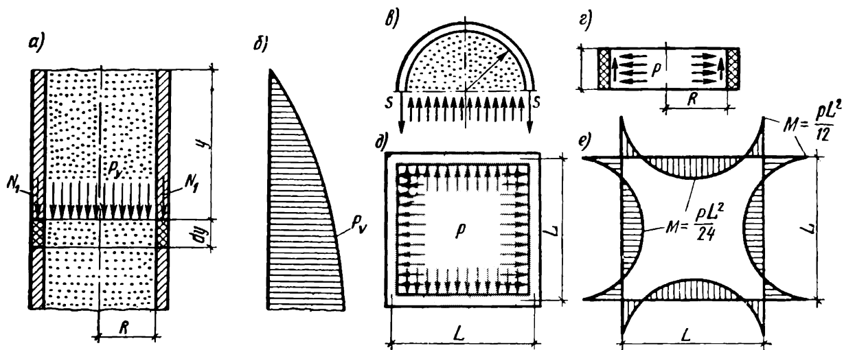
Рис. 6.14. К расчету стен силоса
