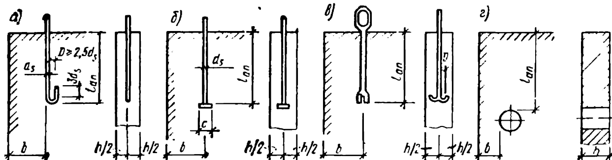
Рис. 7.2. Строповочные приспособления:
