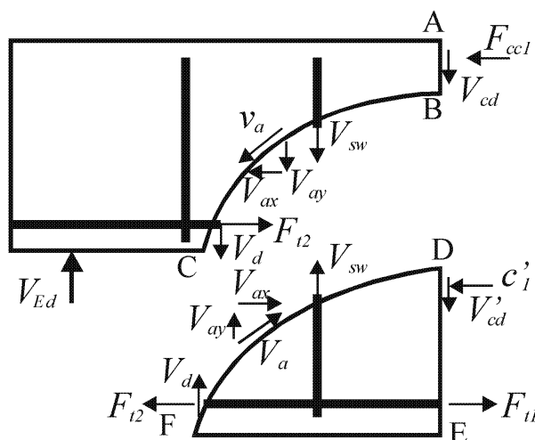
Рис. 2.14. Схема внутренних усилий в наклонном сечении балки
