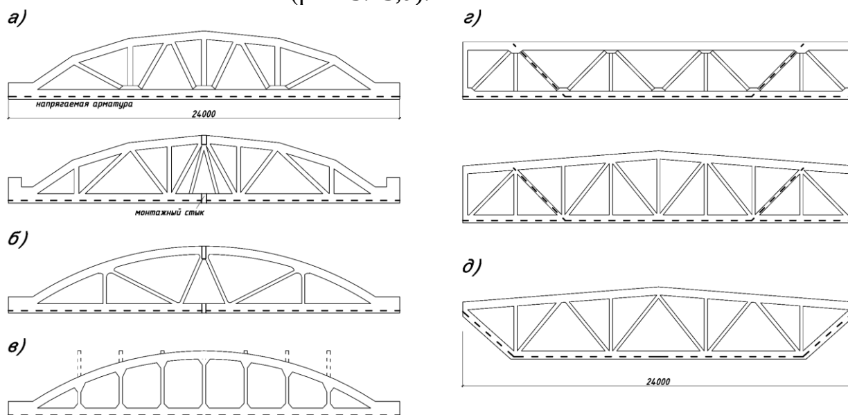
Рис. 5.25. Конструктивные схемы железобетонных ферм
