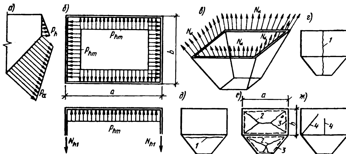
Рис. 6.8. К расчету бункеров:
