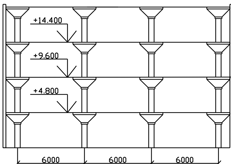
Рис. 4.5. Конструкции зданий многоэтажных промышленных зданий с безбалочными перекрытиями
