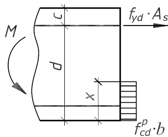
Рис. 3. Схема усилий в сечении балки при подъеме
