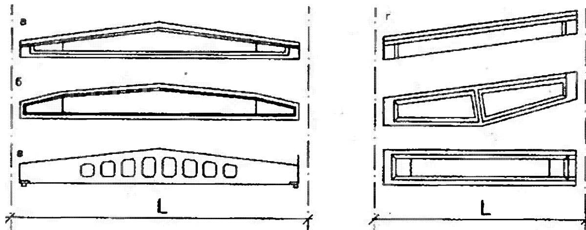
Рис. 5.24. Конструктивные схемы балок покрытий
