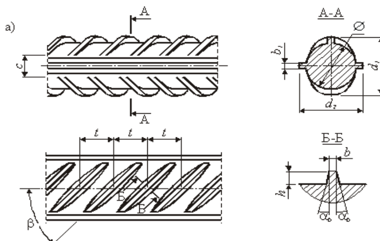
Рис.1.9. Геометрические параметры периодического профиля, наносимого на поверхность арматуры в процессе производства
