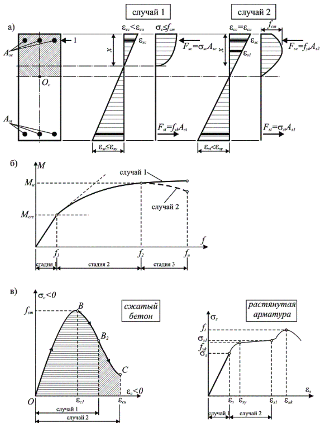
Рис. 1.21. Распределение деформаций и напряжений по высоте нормального сечения в стадии 3 напряженно-деформированного состояния (а), зависимость « M-f » (б) и текущие значения напряжений в бетоне и арматуре (в)
