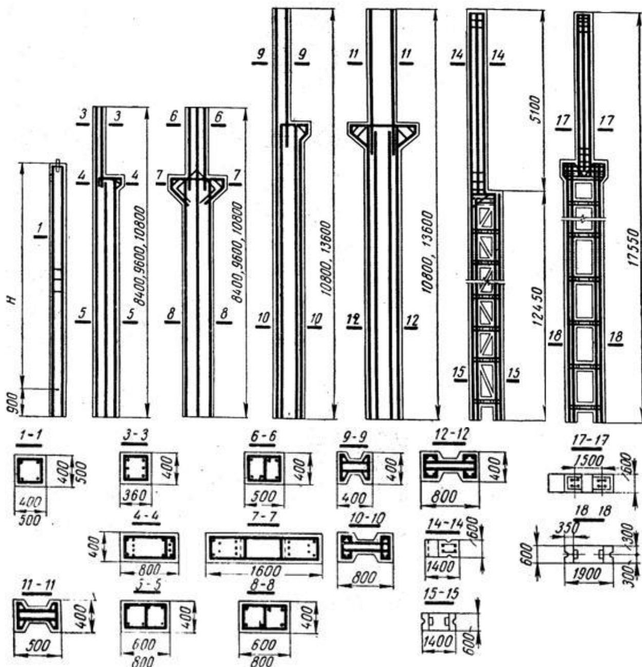
Рис. 5.8. Конструкции колонн одноэтажных зданий
