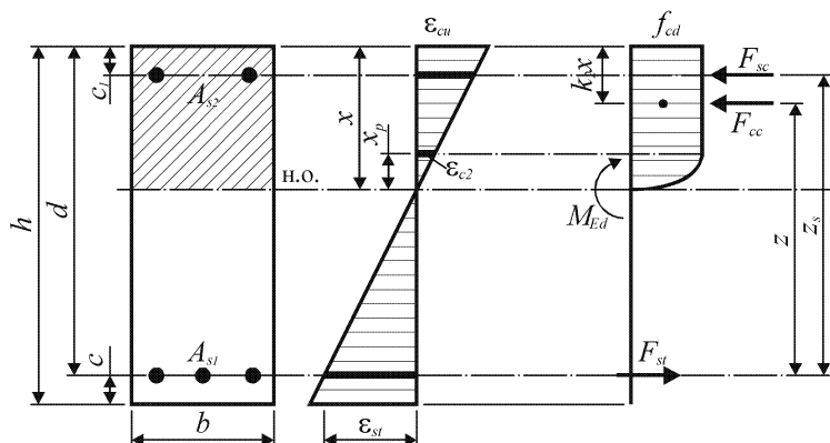
Рис. 2.9. Схема усилий и деформаций в сечении с двойным армированием при расчете упрощенным деформационным методом
