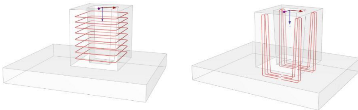
Рис. 4.53. Схематичное изображение горизонтальной и вертикальной арматуры подколонника
