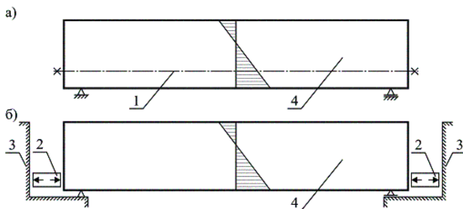
Рис. 2.18. Предварительное напряжение конструкций при обжатии рабочей арматурой (а) и реакциями внешнего ограничения (б) – жесткими упорами
