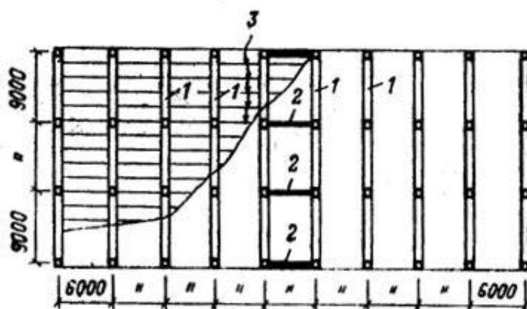
Рис. 4.3. Конструктивный план многоэтажного каркаса промышленного здания 1 – поперечные рамы; 2 – продольные вертикальные связи; 3 – панели перекрытий
