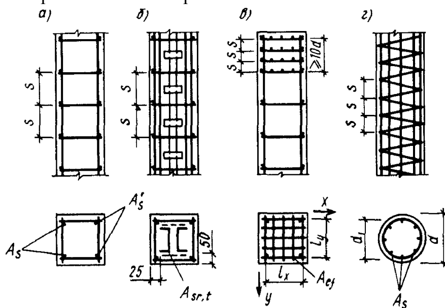
Рис. 2.24. Виды армирования сжатых элементов
