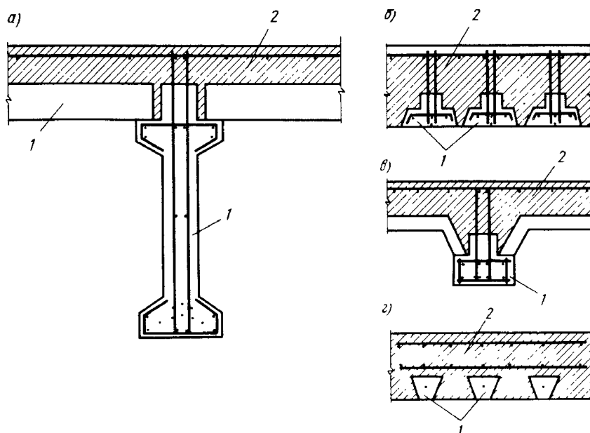
Рис. 4.40. Виды сборно-монолитных перекрытий: 1 – сборные элементы; 2 – монолитный бетон
