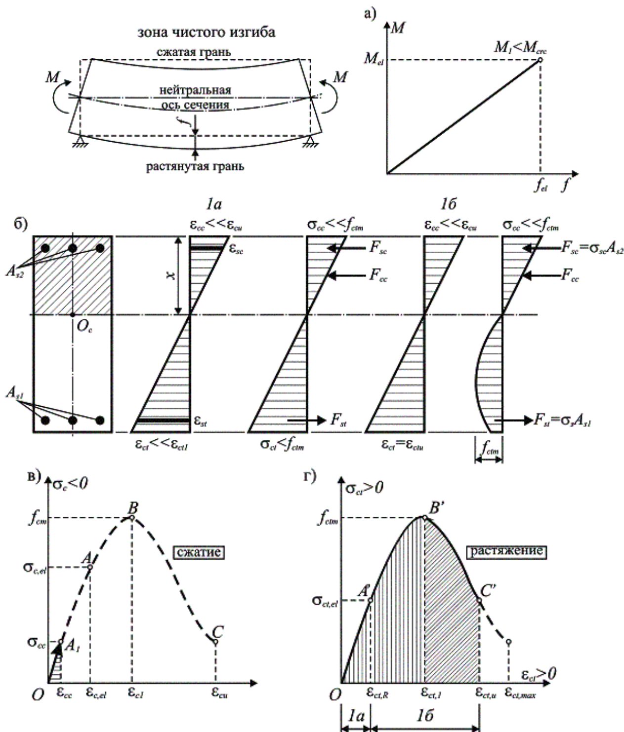
Рис. 1.17. Распределение деформаций и напряжений по высоте нормального сечения в стадии 1 напряженно-деформированного состояния
