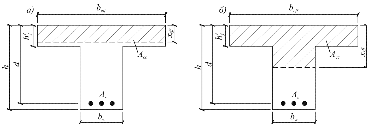
Рис. 2.13. Положение границы условной сжатой зоны в сечении изгибаемого железобетонного элемента таврового сечения
