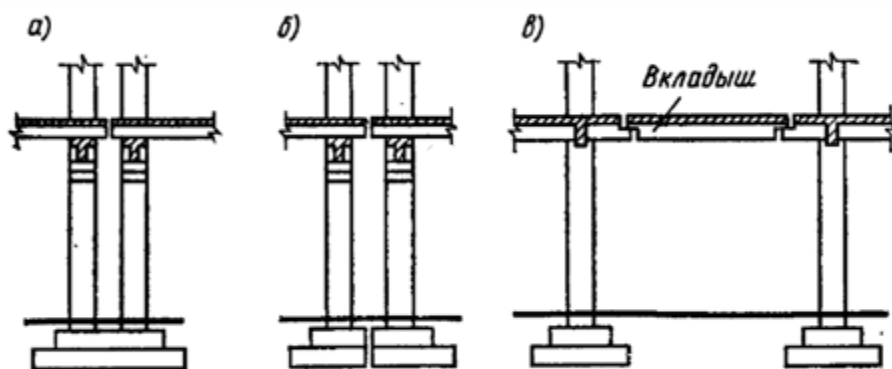
Рис. 4.2. Деформационные швы
