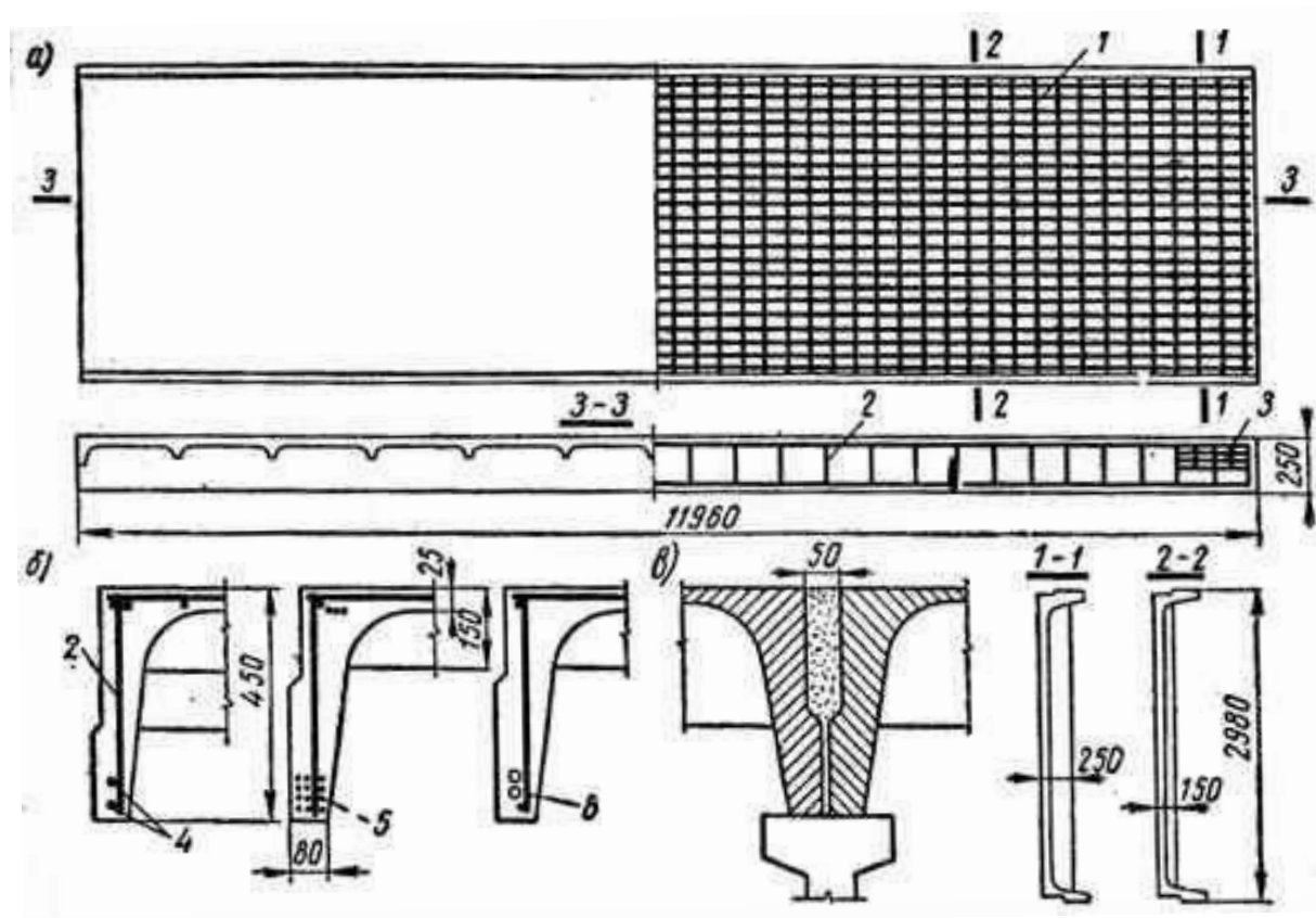
Рис. 5.19. Конструкция крупноразмерной панели покрытия 12×3 м а – конструкция панели; б – варианты армирование стержневой, проволочной и прядевой арматурой; в – сопряжение панелей; 1 – сетка плиты; 2 – каркас ребра; 3 – угловая сетка; 4 – стержни; 5 – предварительно напряженная проволочная арматура; 6 – пряди
