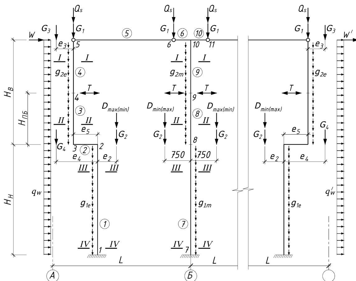
Рис. 5.6. Расчетная схема поперечной рамы с учитываемыми нагрузками
