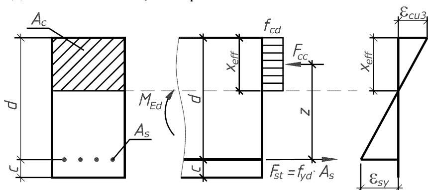
Рис. 2.6. Схема распределения усилий и деформаций в сечении
