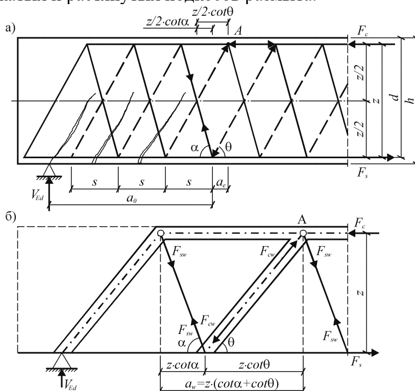
Рис. 2.15. К расчету прочности наклонных сечений по методу ферменной аналогии а – идеализированная ферма; б – заменяющая ферма с подкосами
