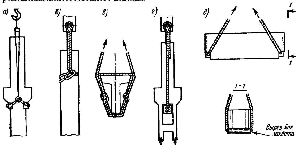
Рис. 7.1. Способы строповки сборных элементов без применения закладных строповочных устройств:
