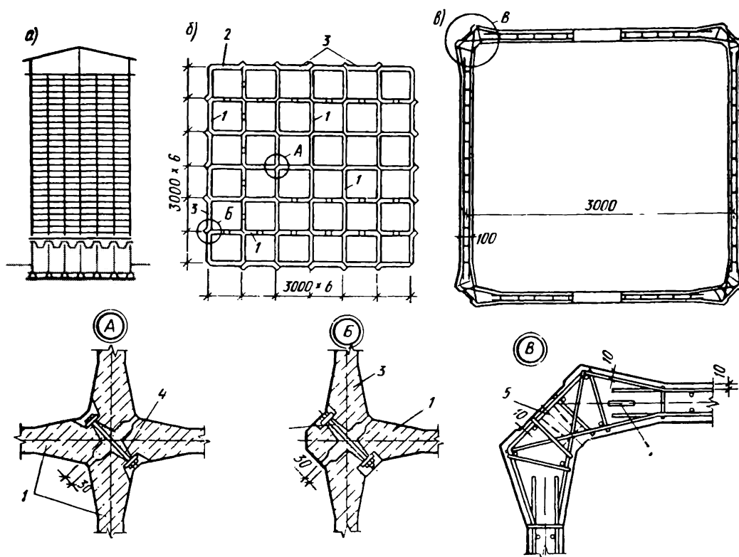
Рис. 6.13. Конструкции сборных прямоугольных силосов: а – поперечный разрез; б – план компоновки силоса; в – объемный блок прямоугольного силоса с гладкими стенами; 1 – объемный блок; 2 – Г-образный угловой элемент; 3 – плоская панель; 4 – соединительные болты; 5 – отверстия для болтов; 6 – петли для подъема
