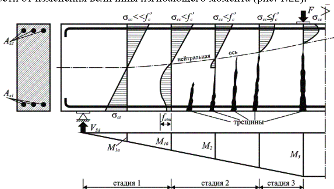
Рис. 1.22. Изменение по длине балки характерных стадий напряженно-деформированного состояния
