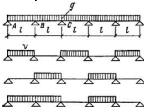
Рис. 4.24. Схемы загрузки неразрезной балки
