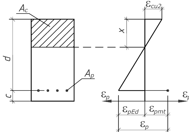
Рис. 1. Распределение деформаций по высоте сечения
