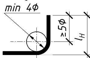
Рис. 4.47. Анкеровка стержней арматурной сетки
