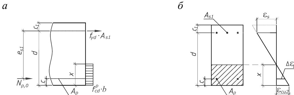
Рис. 4. Сечение балки при отпуске арматуры:
