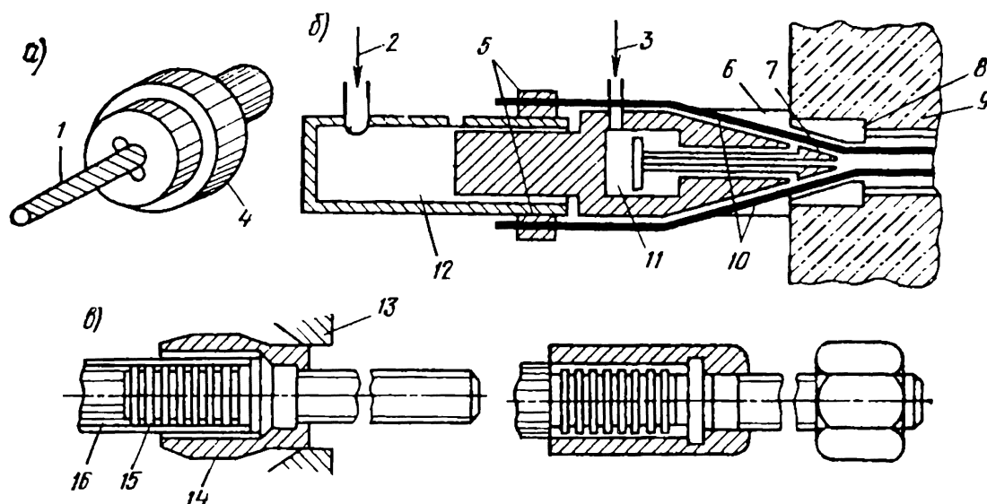
Рис. 2.21. Анкеровка напрягаемой проволоочной арматуры в предварительно напряженных элементах:
