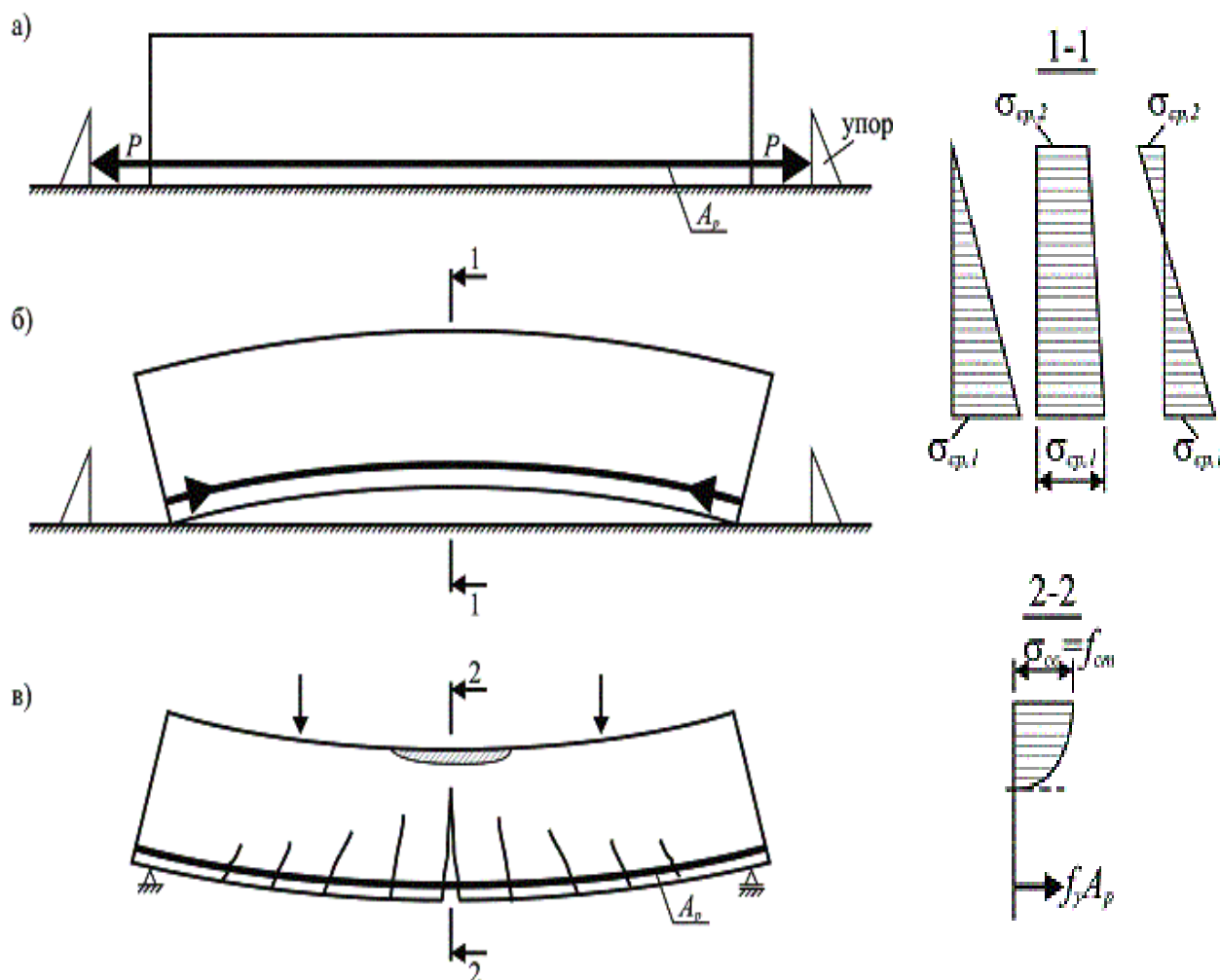
Рис. 1.2. Предварительно напряженная балка:
