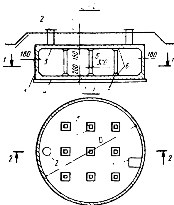
Рис. 6.5. Конструктивное решение круглого монолитного резервуара: 1 – стенка резервуара; 2 – люк; 3 – перекрытие; 4 – днище; 5 – колонна; 6 – капитель колонны; 7 – приямок
