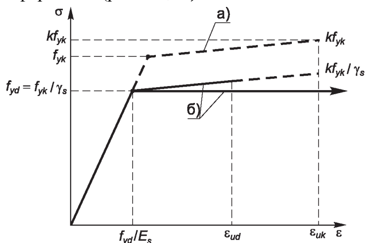
Рис. 1.12. Идеализированные диаграммы деформирования для арматуры (при растяжении и сжатии): а – характеристическая; б – расчетная
