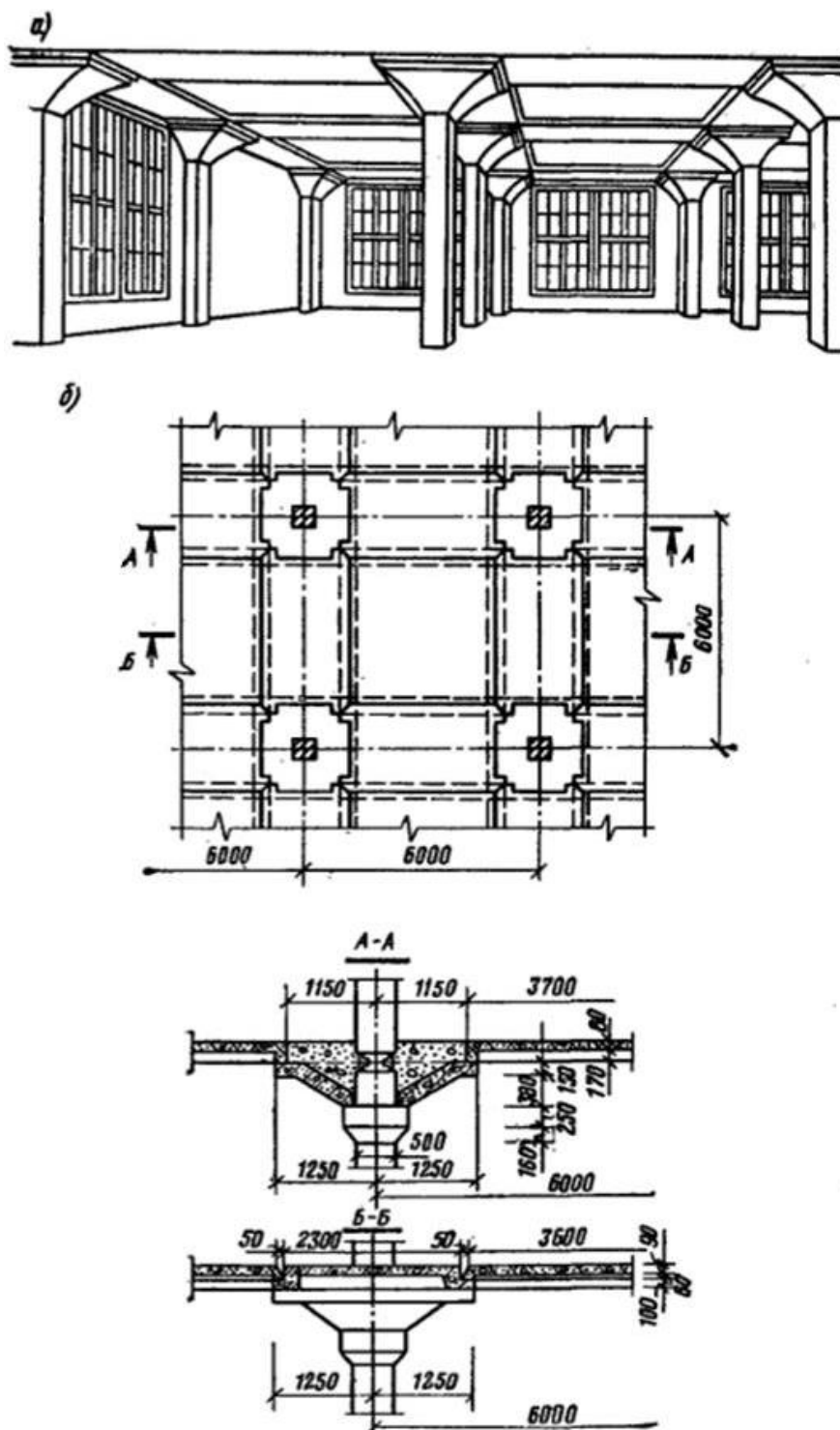
Рис. 4.31. Конструкция безбалочного сборного перекрытия с ребристыми панелями:
