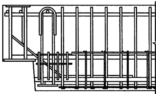
Рис. 4.18. Армирование опорной зоны ригеля
