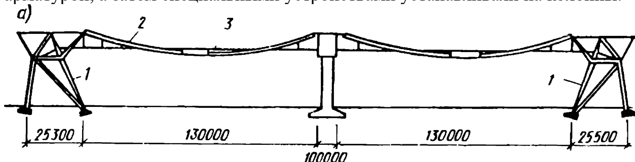
Рис. 5.39. Поперечный разрез висячего покрытия ангара:
