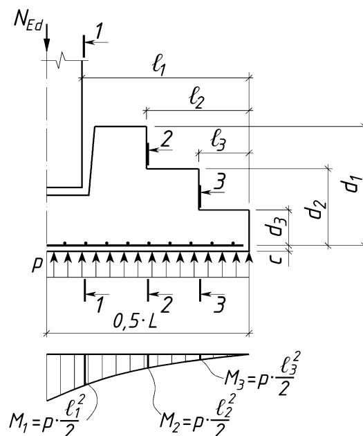
Рис. 4.46. Расчетная схема фундамента при расчете его плитной части
