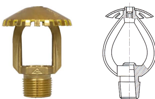
Рис. 8.7. Дренчерный ороситель
