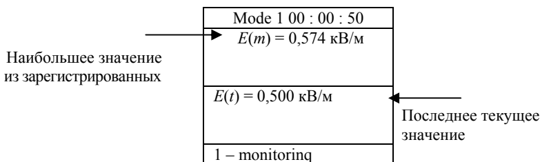
Рис. 7.3. Изображение экрана прибора СТ-01
