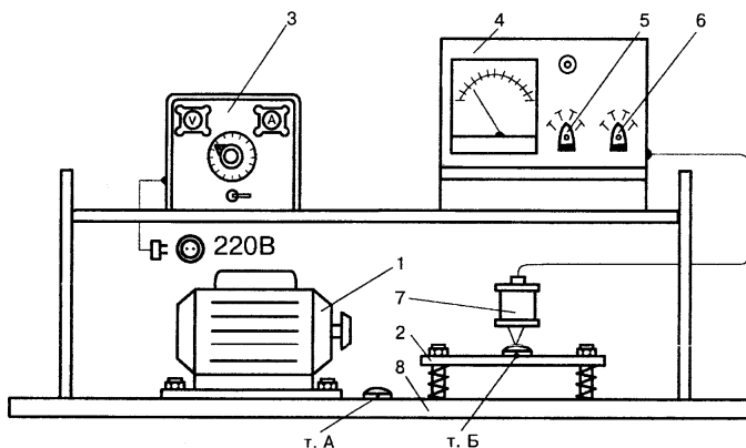
Рис. 6.2. Экспериментальная установка:
