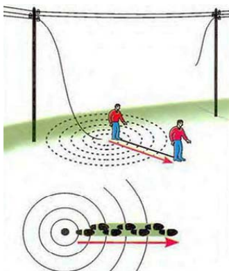
Рис. 9.7. Перемещение в зоне шагового напряжения
