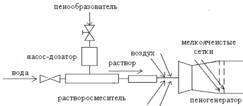
Рис. 8.1. Схема получения воздушно-механической пены
