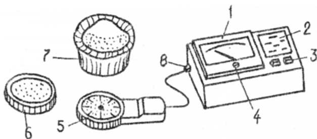
Рис. 2.1. Люксметр Ю-116:
