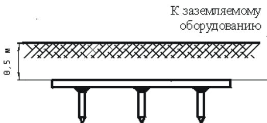
Рис. 1.2. Схема расположения заземляющего устройства в грунте
