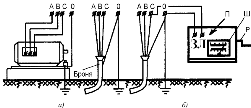
Рис. 1.4. Схема измерения сопротивления изоляции электроустановок
