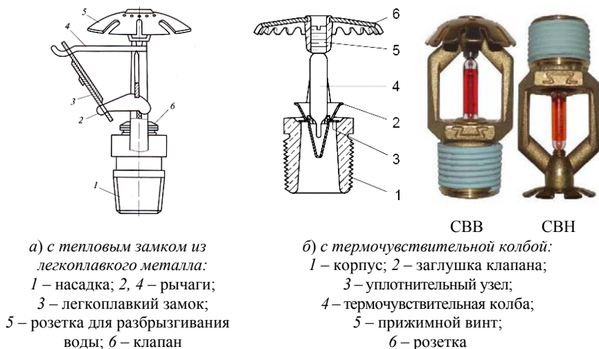
Рис. 8.6. Спринклерные оросители
