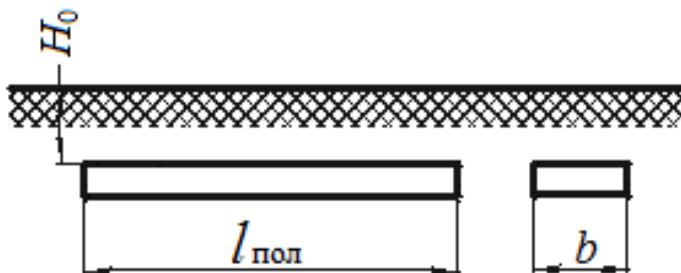
Рис. 1.5. Горизонтальный полосовой заземлитель
