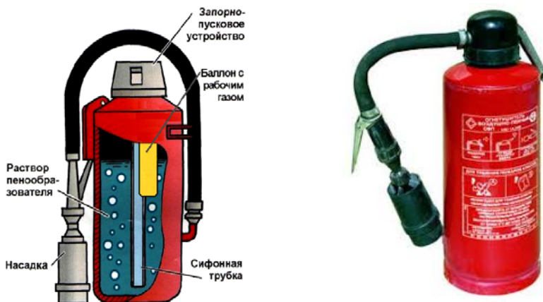
Рис. 8.4 Огнетушитель воздушно-пенный
