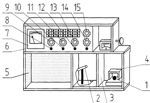
Рис. 5.2. Схема экспериментальной установки:
