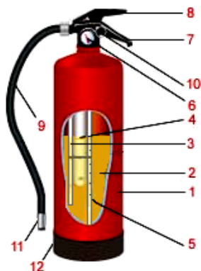
Рис. 8.5. Огнетушитель порошковый ОП-10:
