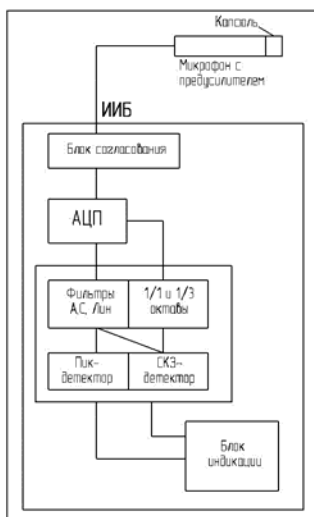
Рис. 5.3. Схема шумомера «Октава-101А»
