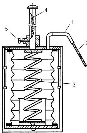
Рис. 4.1. Газоанализатор УГ-2:
