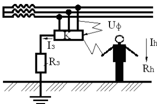
Рис. 1.1. Принципиальная схема защитного заземления:
