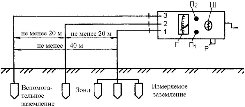
Рис. 1.3. Схема измерения сопротивления заземляющих устройств
