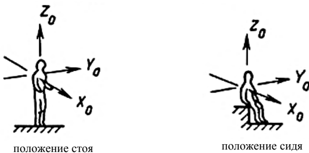
Рис. 6.1. Направление координатных осей при действии вибрации
