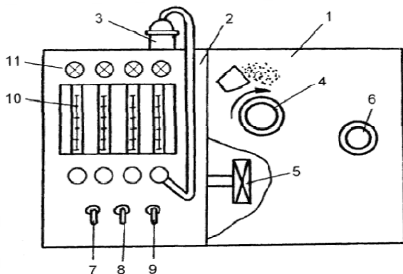
Рис. 4.2. Экспериментальная установка:
