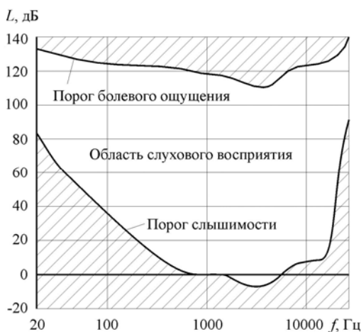
Рис. 5.1. Область слухового восприятия человека
