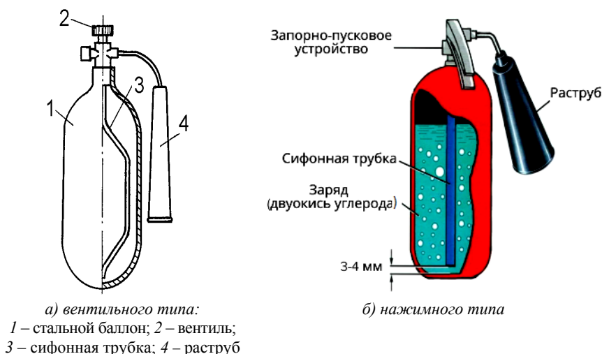
Рис. 8.3. Огнетушитель углекислотный
