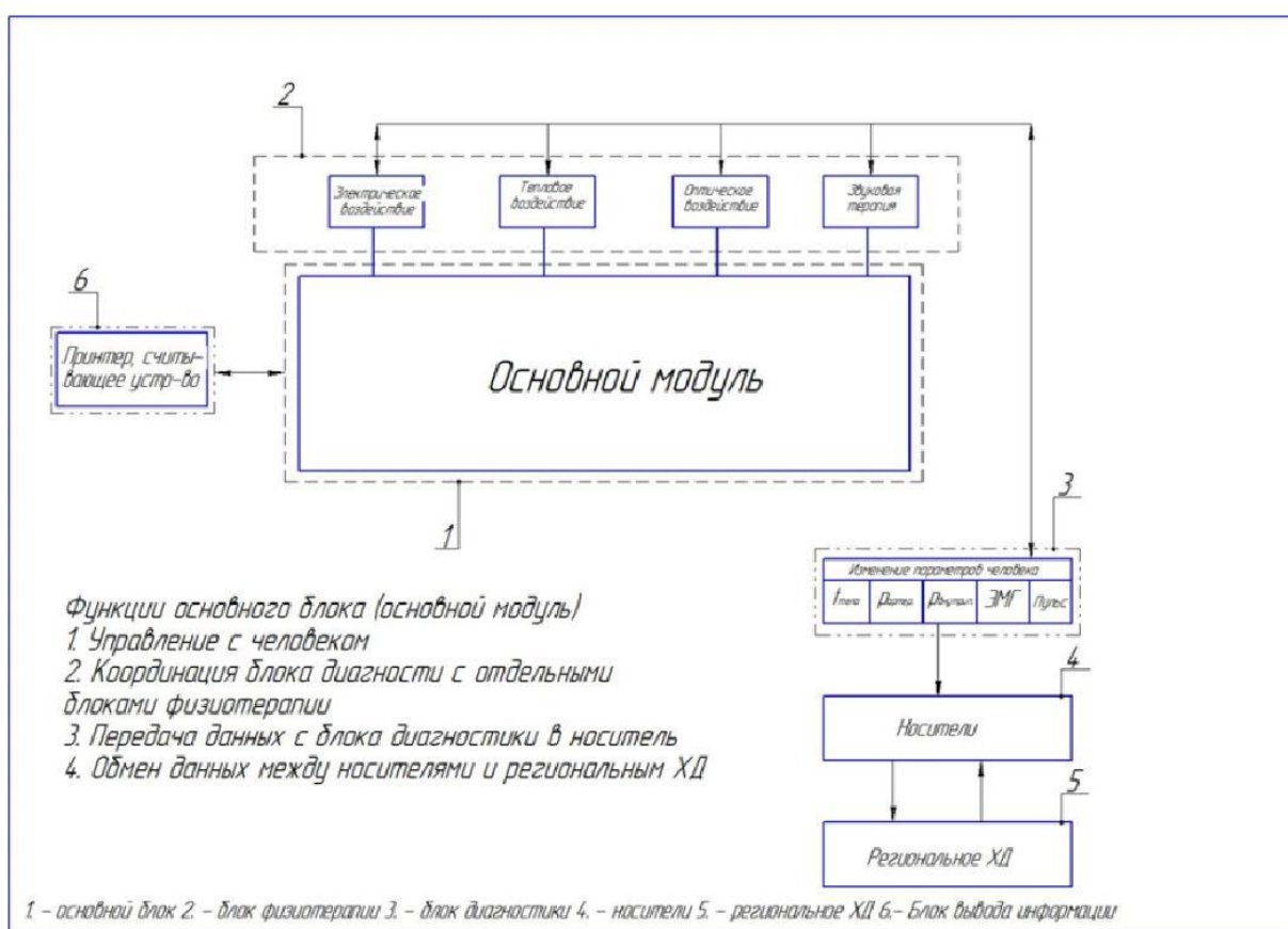
Рисунок 1 - Структура модульного физиотерапевтического комплекса Создание блочно-модульных аппаратов позволит увеличить эффективность физиотерапевтических процедур.
