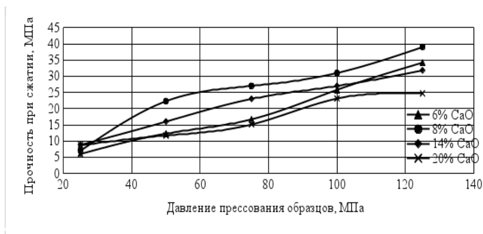
Рис. 1. Влияние давления прессования образцов из гранитного отсева и извести на прочность при сжатии
